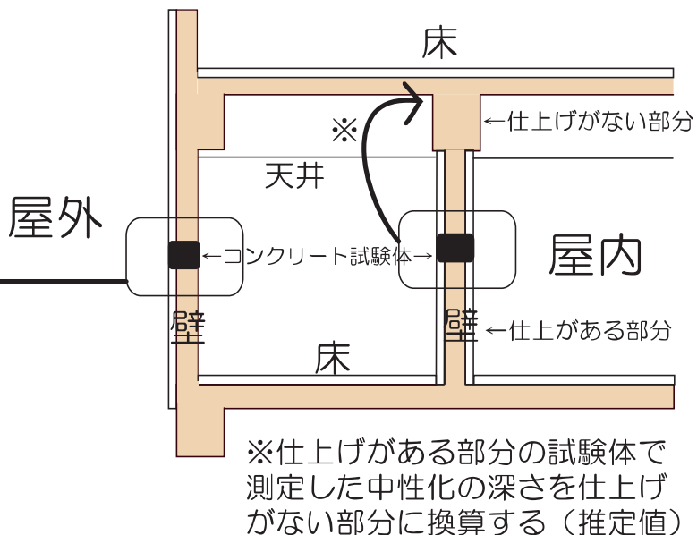
建物断面図
