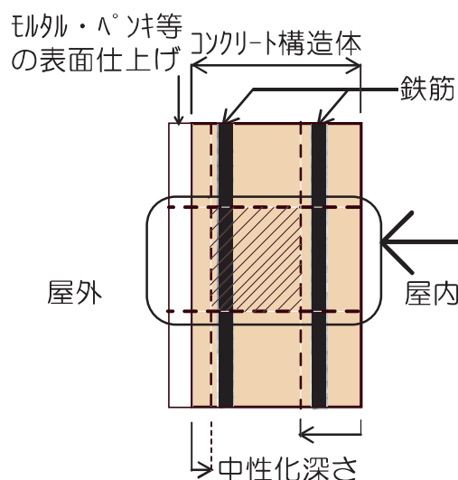
壁 断面図
