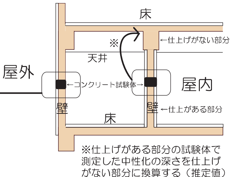
建物断面図
