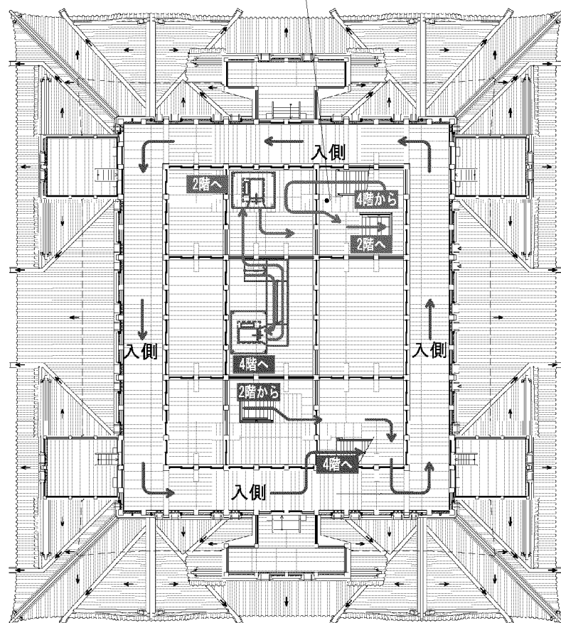
3階 観覧計画
