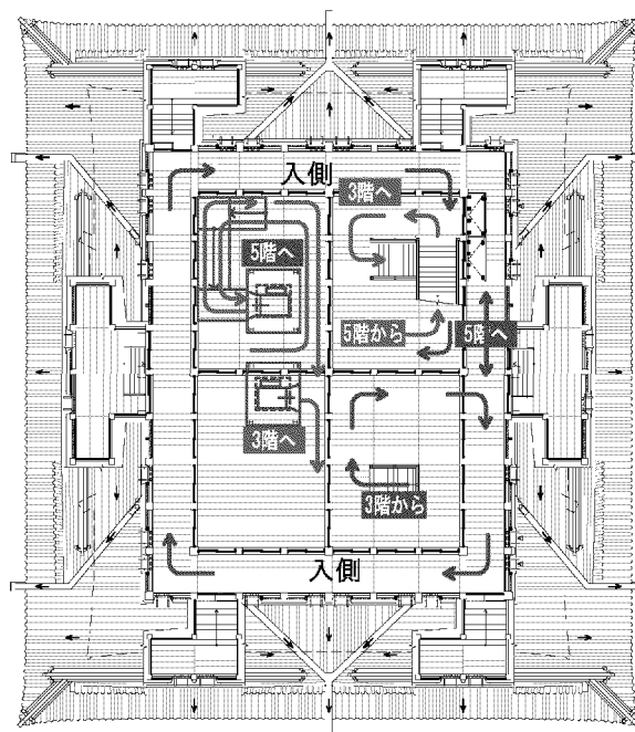
4階 観覧計画
