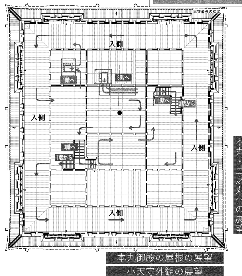
2階 観覧計画
