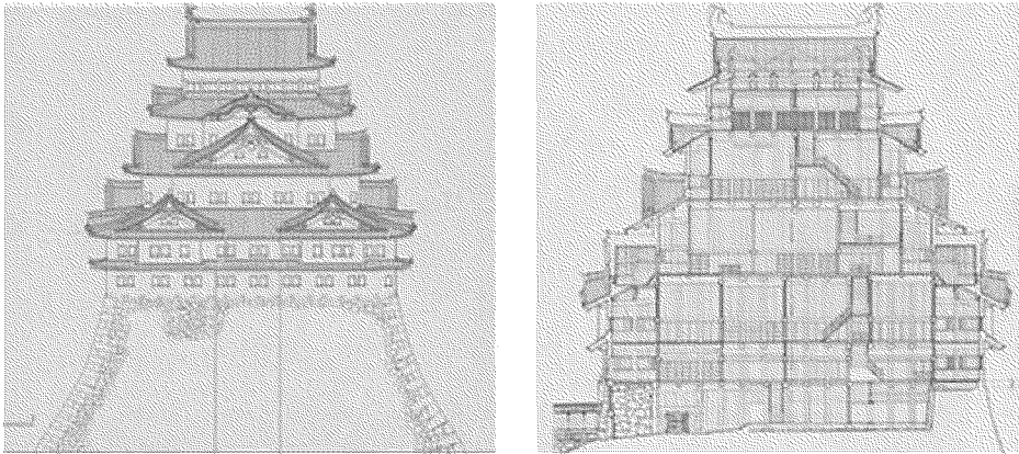
昭和実測図
