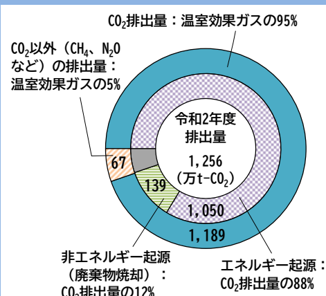
◆図2 温室効果ガス排出量の内訳（2020年度）
