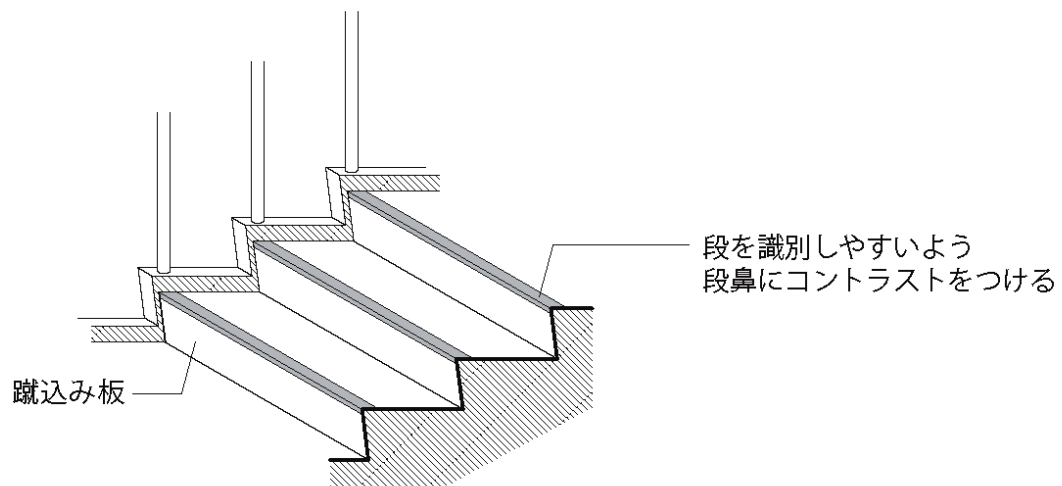
図8 階段の段鼻と蹴込み板（例）
