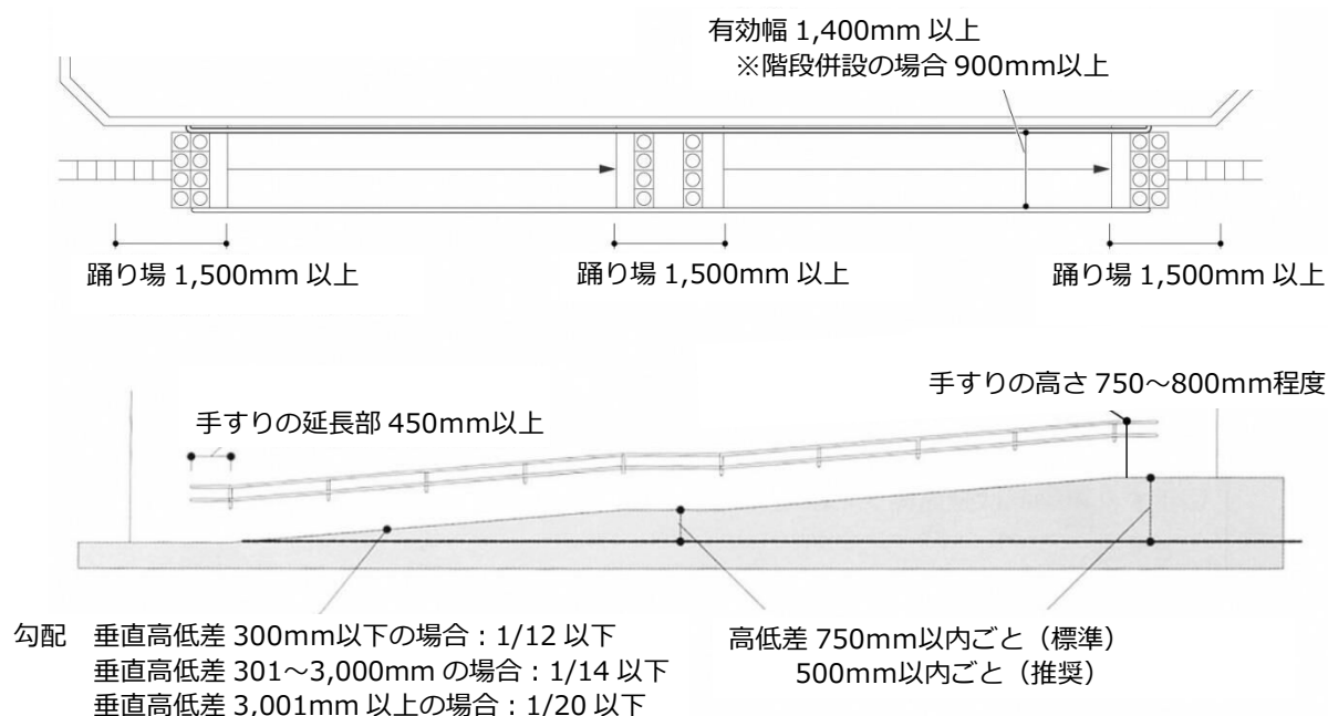
図4 傾斜路(例)
