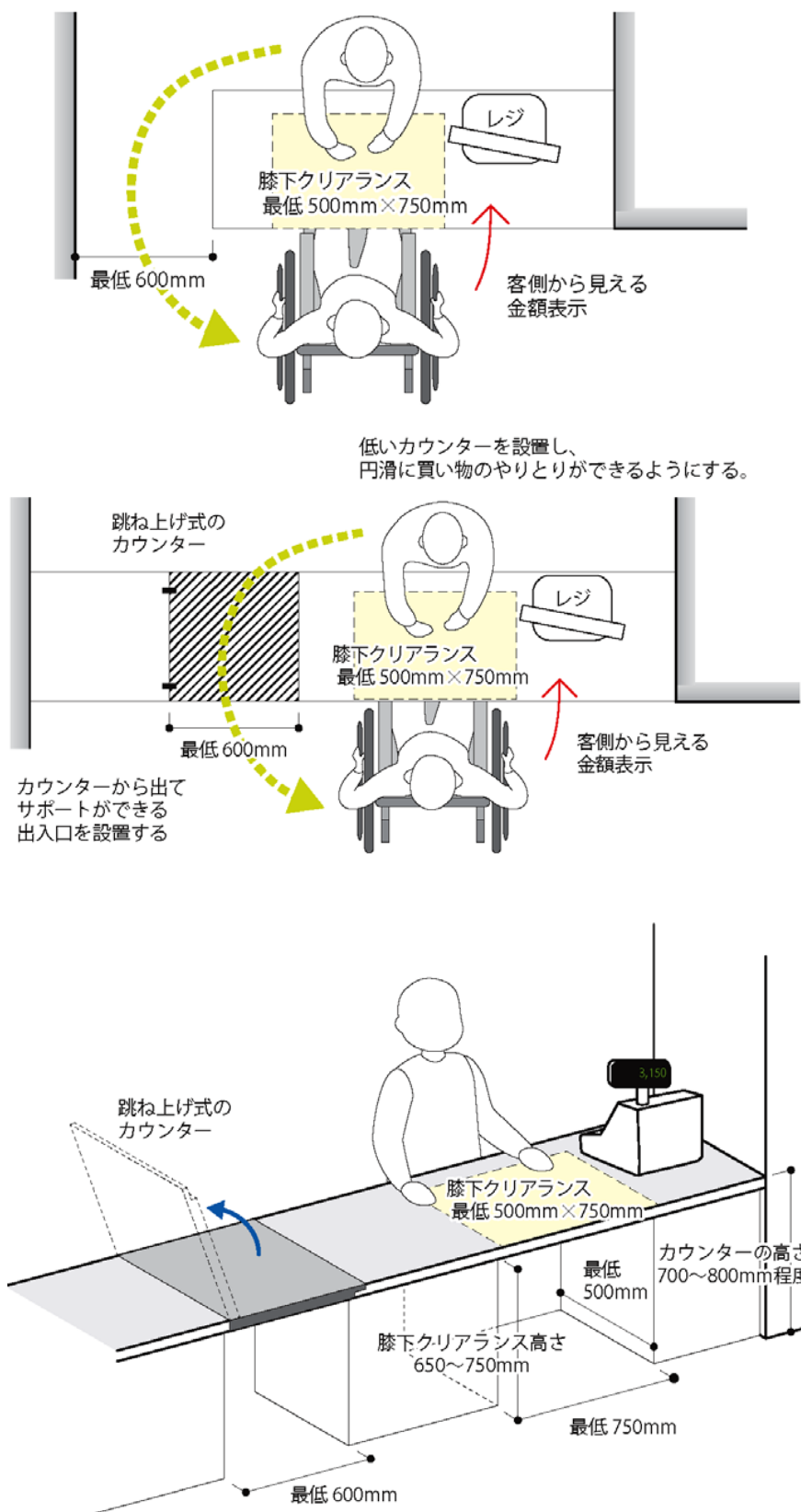
図9 レジ/サービスカウンター（例）
