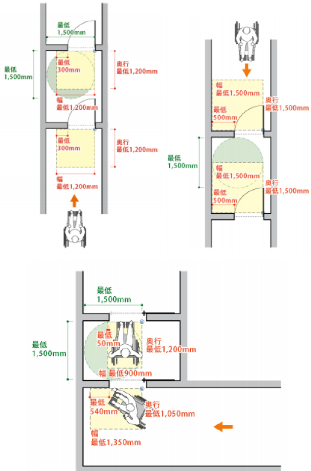
図 14 ドア周辺の操作スペース (例)
