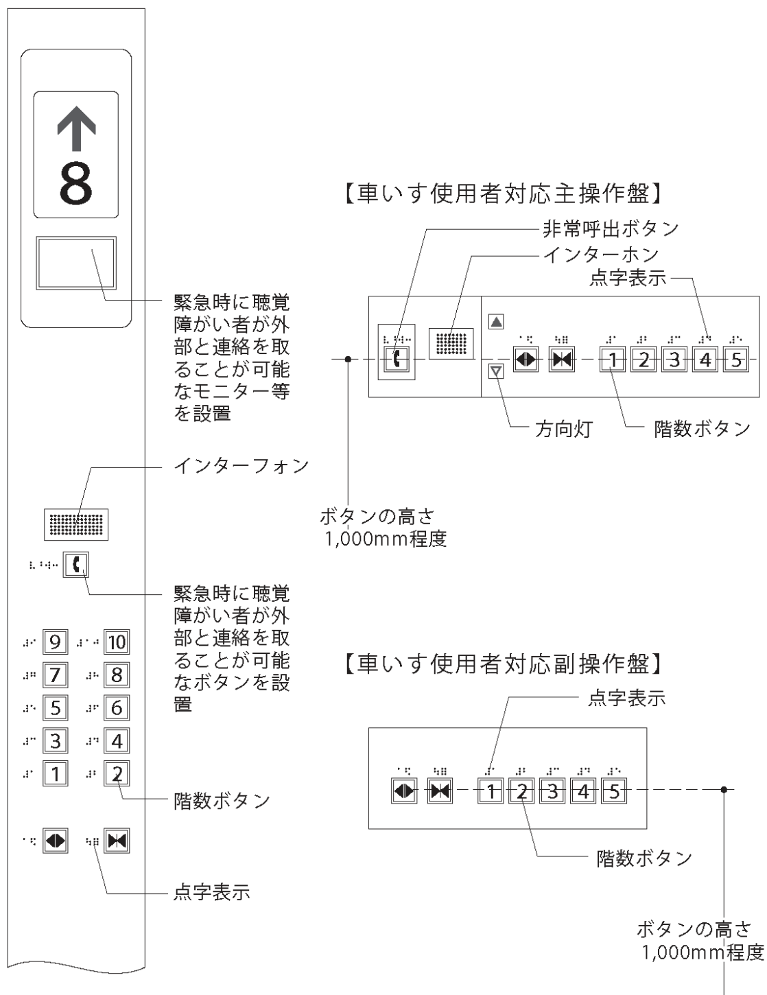
図 17 エレベーターの操作盤（例）
