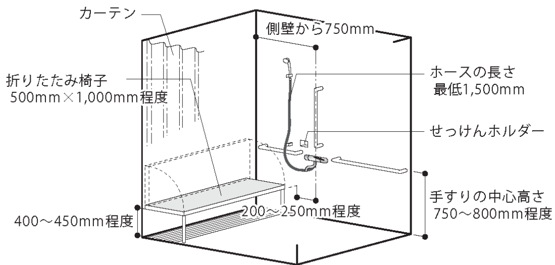
図26 アクセシブルなシャワー（例）
