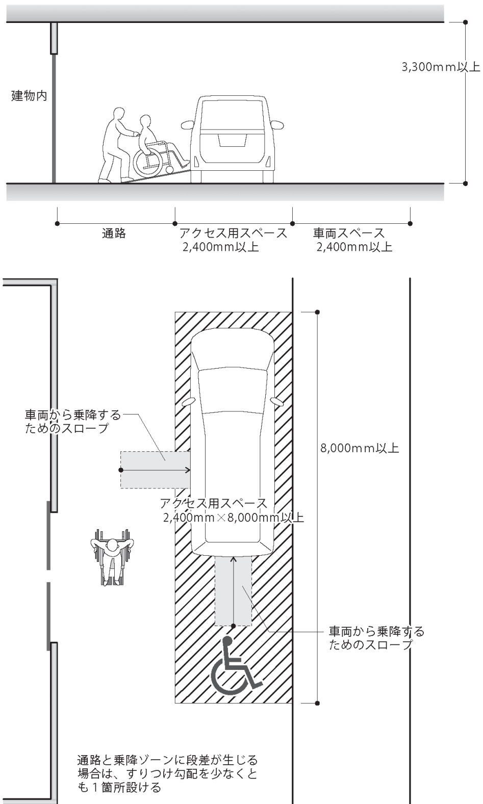
図3 車両乗降ゾーン(例)
