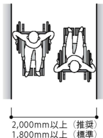
図1 通路の幅(例)
