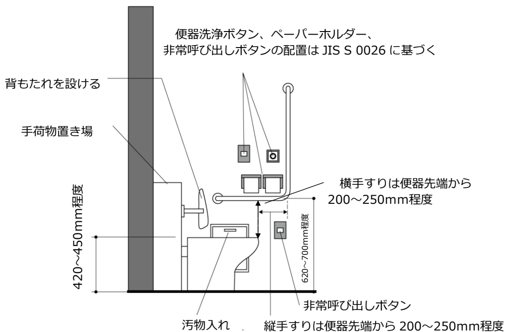
図25 便器周りの配置（例）
