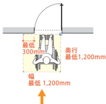
B-2 ラッチ側からアプローチ (押し手側)
