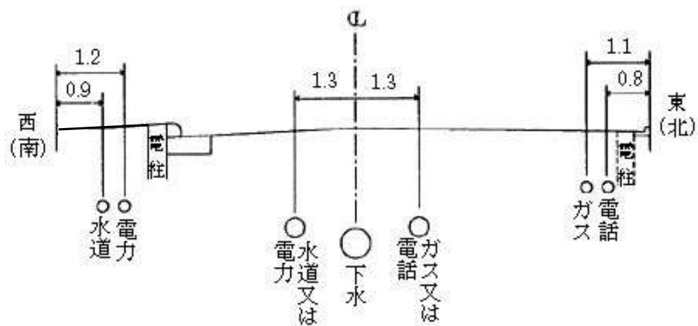
第 4図 道路幅員7.27メートル以上10メートル未満
