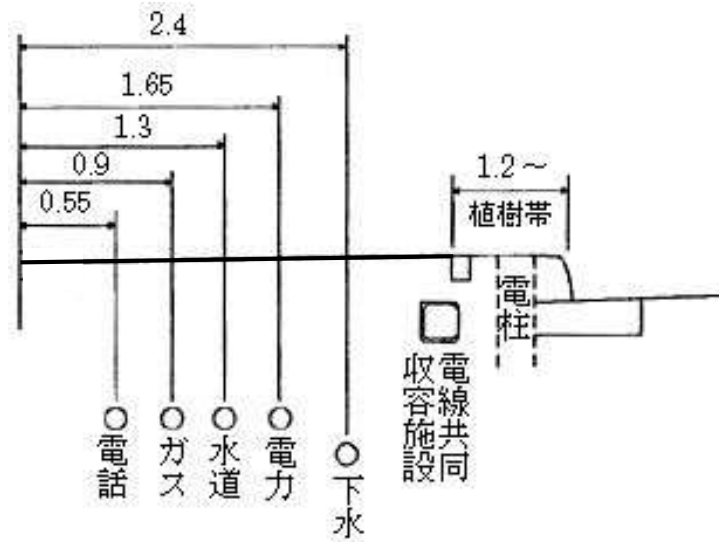
第 9図 歩道幅員 4メートル以上 5.7メートル未満
