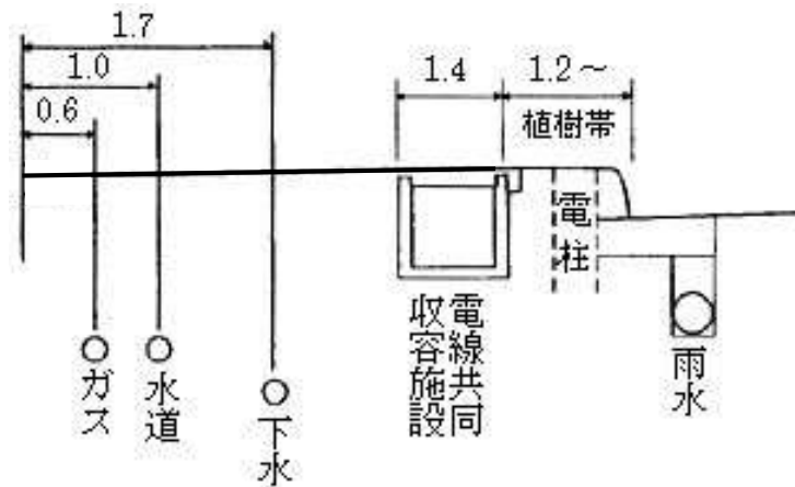
第11図 歩道幅員 5メートル以上（新設の場合に限る。）
