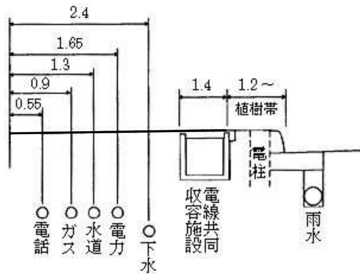
第10図 歩道幅員 5.7メートル以上
