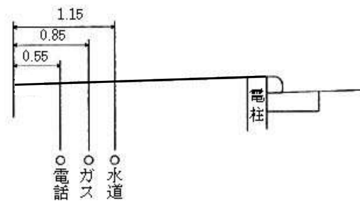
第 5図 歩道幅員 2メートル以下
