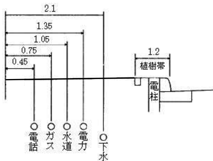
第 8図 歩道幅員 3.5メートル以上 4メートル未満
