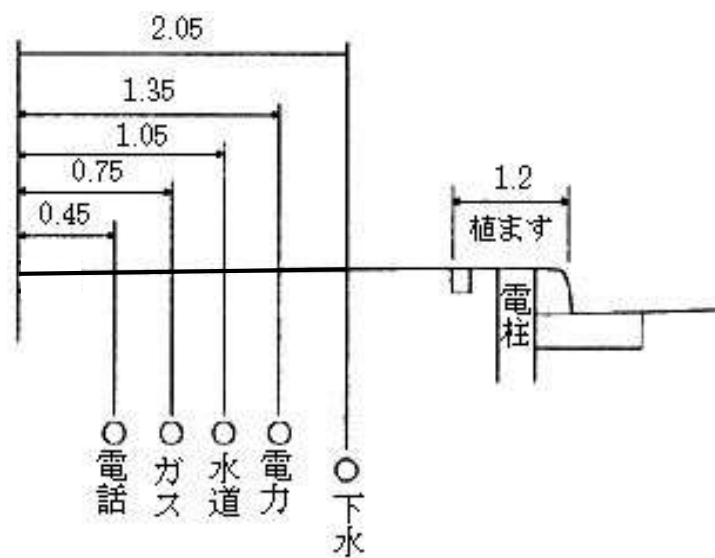
第 7図 歩道幅員 3メートル以上 3.5メートル未満
