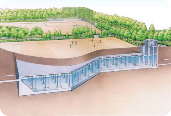
楠調節池完成イメージ
