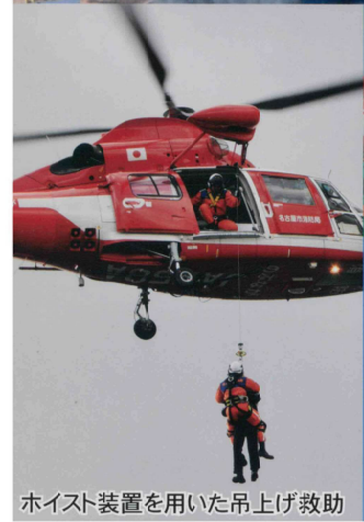
ホイスト装置を用いた吊上げ救助
