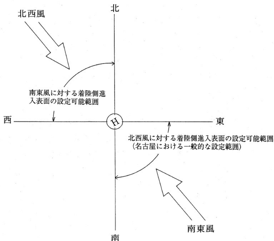
図2-1 風向きに対する進入表面の設定可能範囲
