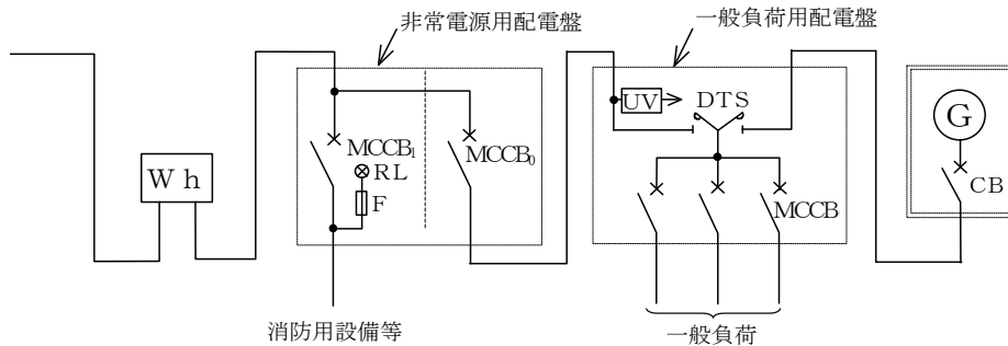
第23-7図d (低圧で受電する場合)
