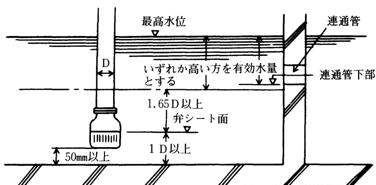
第1-3図 (サクションピットのない場合)
