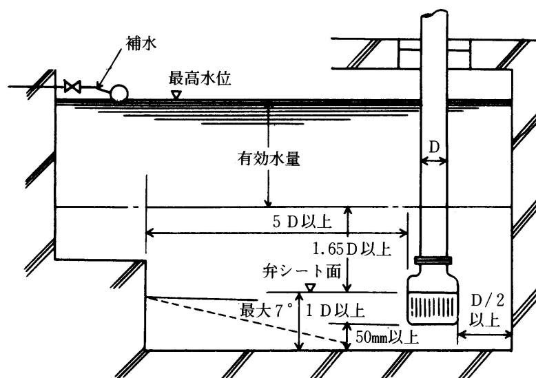
第1－2図（サクシヨンピットのある場合）
