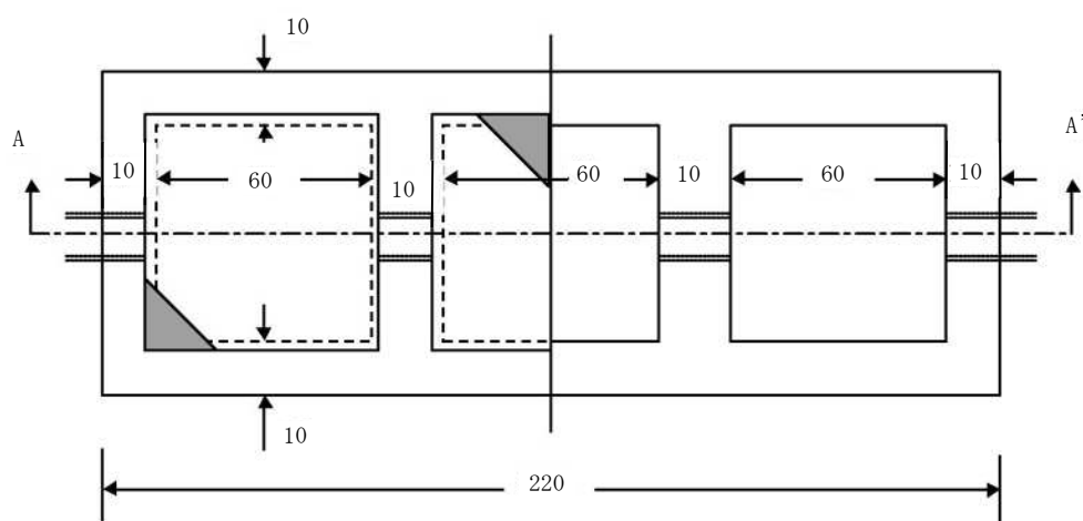
平面図 (B-B'-B'')
