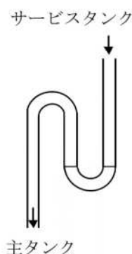
第 5-6 図 トラップ構造
