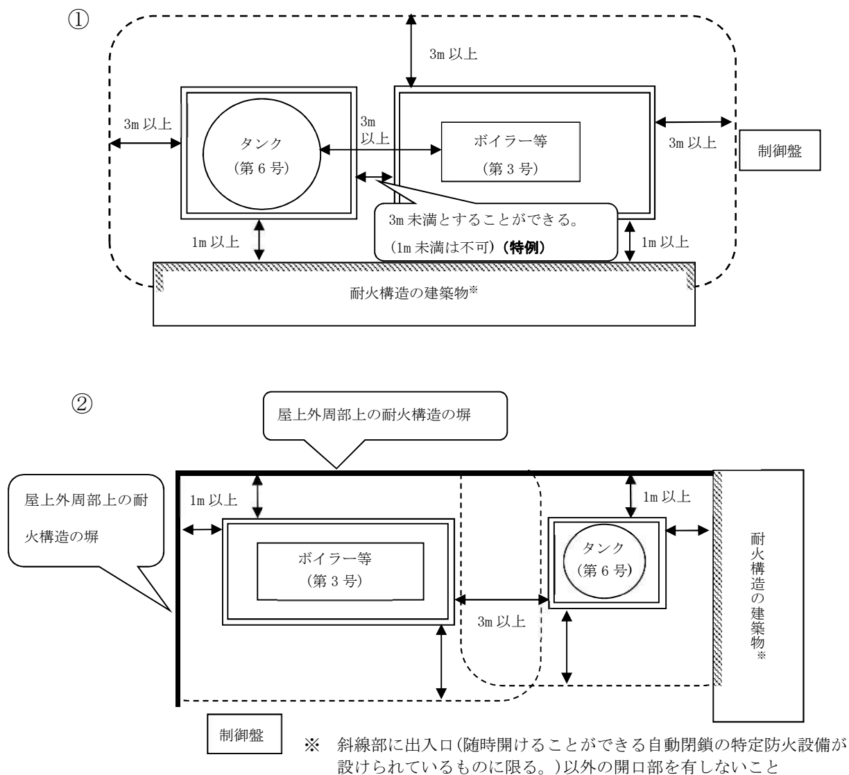
第6-4 図 第7号の空地として認められる例
