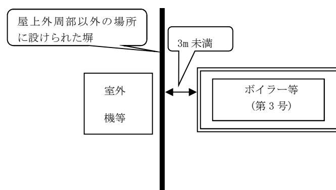
第 6-5 図 第 7 号の空地として認められない例
