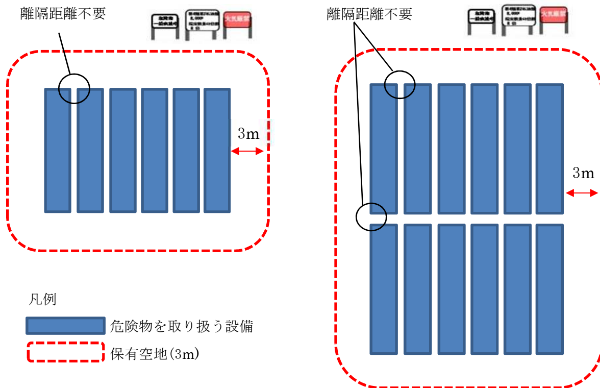
第 6-8 図 全てをまとめて一の一般取扱所とする場合の例
