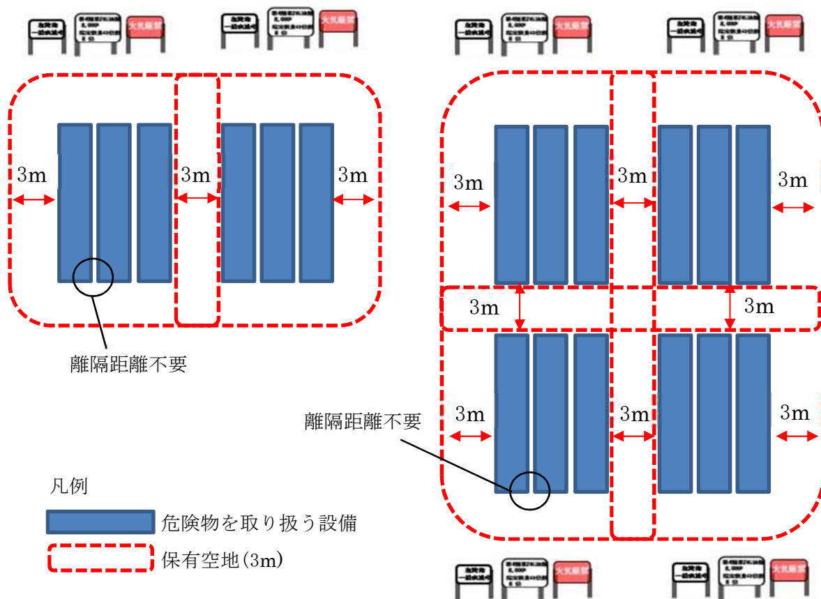
第 6-9 図 複数の一般取扱所とする場合の例
