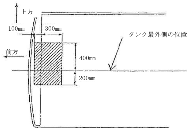
第 12-7 図 タンク本体の応力集中防止範囲
