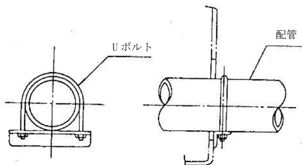
第 12-31 図 吐出口付近の配管の固定方法
