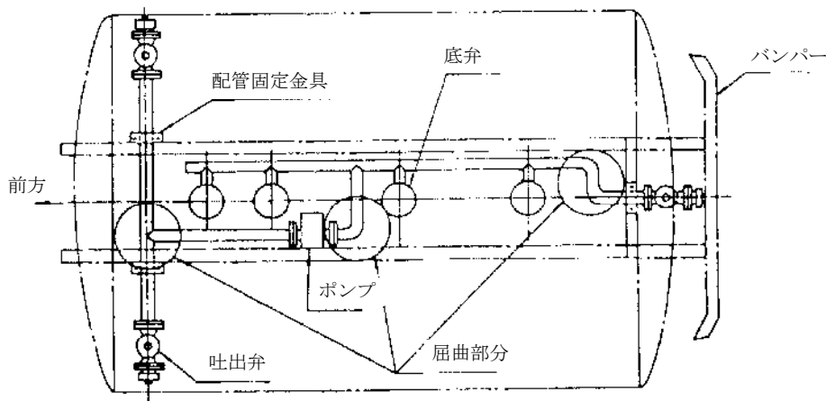
第 12-32 図 配管による底弁に直接衝撃が加わらない措置
