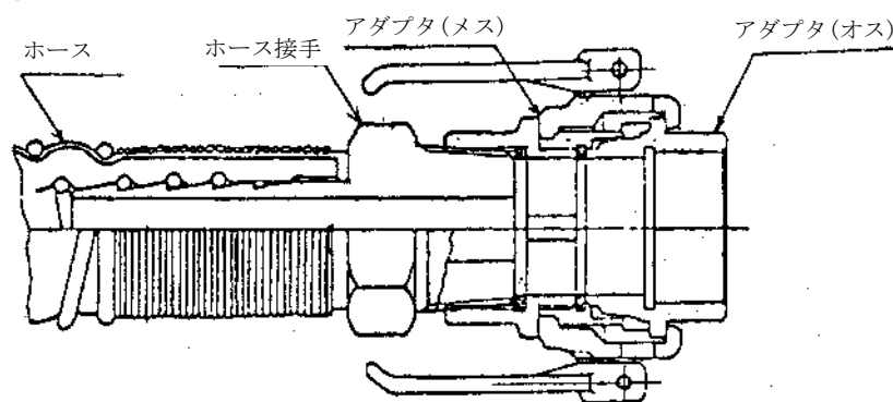
第 12-34 図 突合わせ固定式結合金具の構造例
