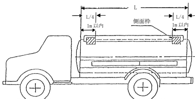
第 12-12 図 単一車形式の移動タンク貯蔵所の側面枠の取付位置
