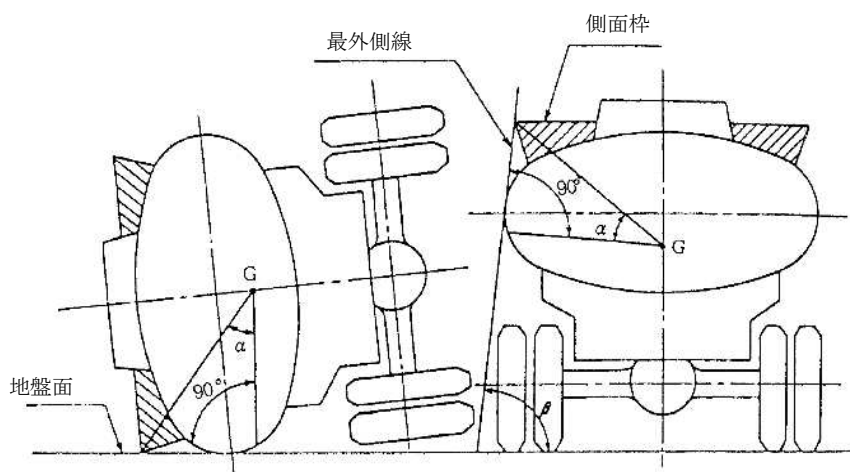
第 12-14 図 接地角度及び取付角度
