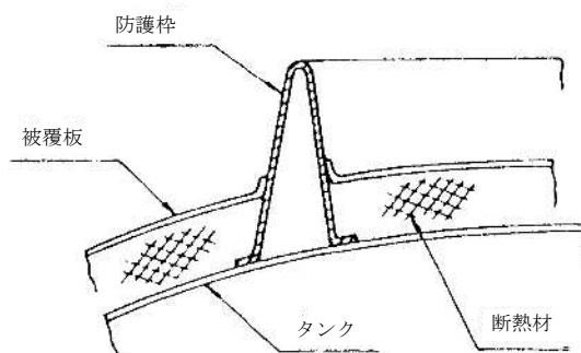
第 12-26 図 タンク胴板に直接取り付ける防護枠
