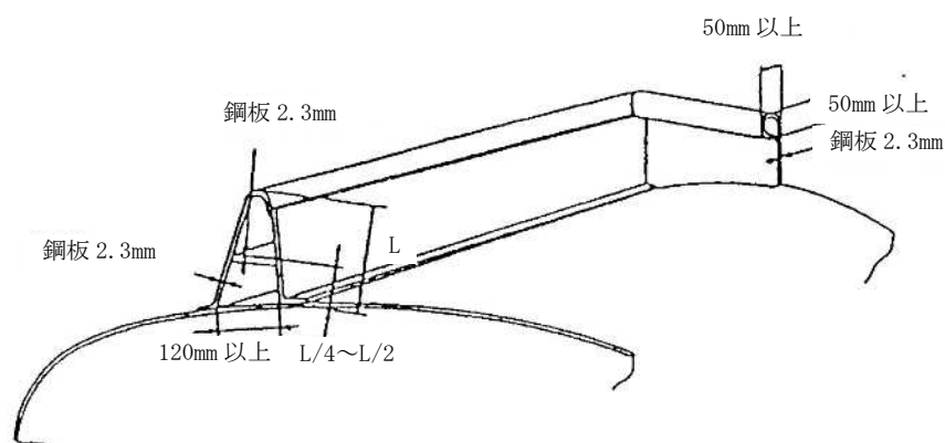
第 12-22 図 防護枠の構造
