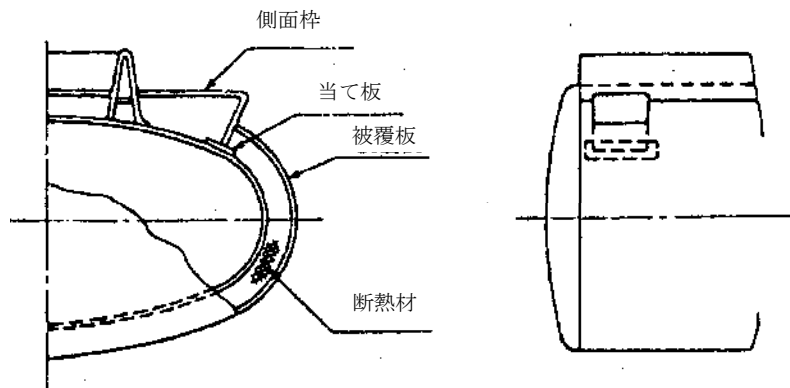
第 12-16 図 タンク胴板に直接取り付ける側面枠の方法
