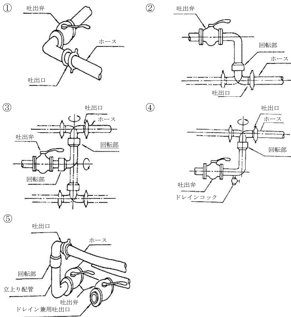
第 12-35 図 配管先端部の構造
