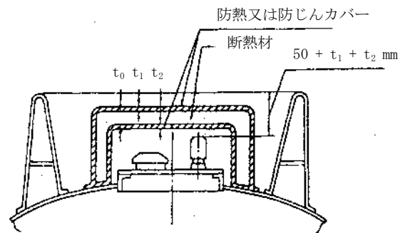
第 12-24 図 防熱又は防じんカバーを設ける移動貯蔵タンクの防護枠
