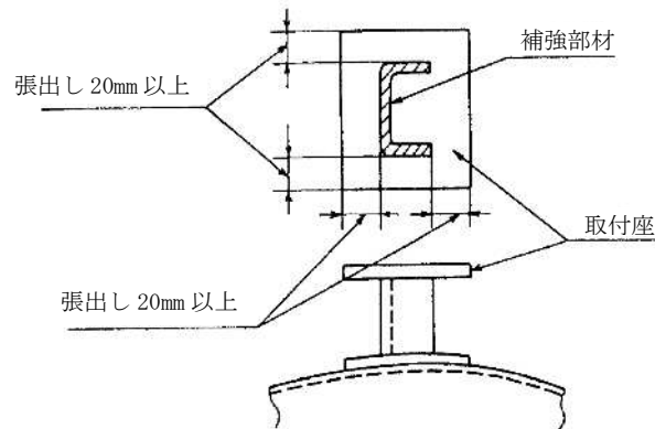
第 12-19 図 補強部材の取付座の大きさ
