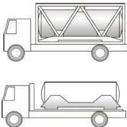
第 12-3 図 単一車形式で積載式の移動タンク貯蔵所の例
