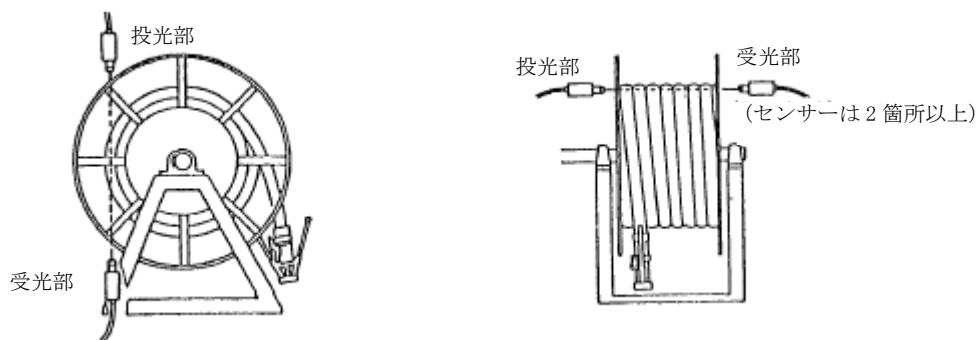
第 12-40 図 ホース巻取装置による誤発進を防止する方法
