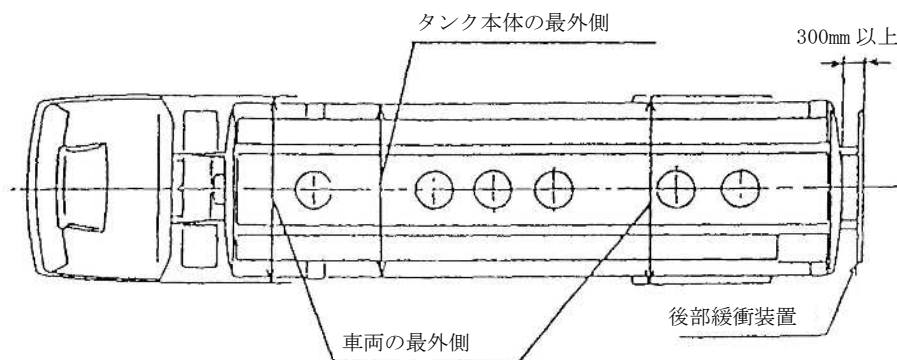
第 12-38 図 最大容量が 20kL を超える移動タンク貯蔵所のタンクの位置
