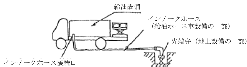
第 12-43 図 給油ホース車のインテークホースの概要
