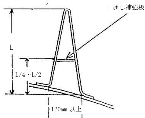
第 12-23 図 防護枠の通し板補強構造
