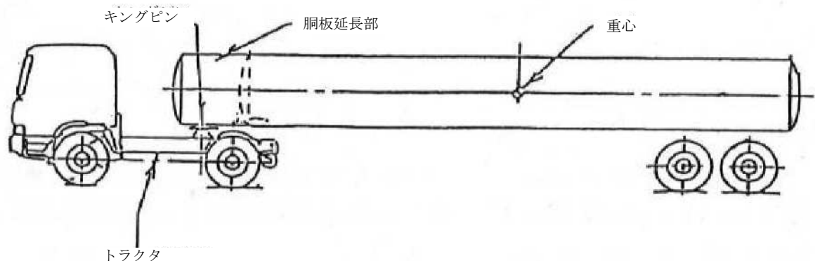
第 12-39 図 胴板を延長した移動タンク貯蔵所
