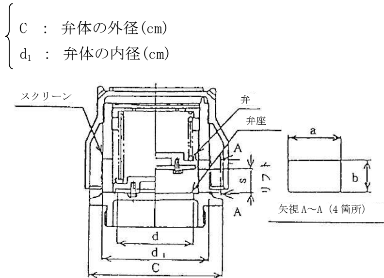
第 12-8 図 安全装置の構造
