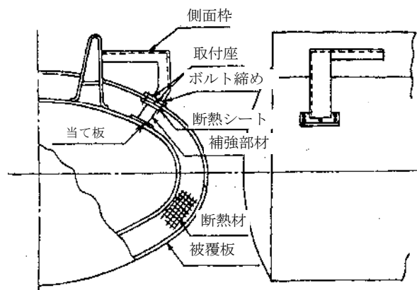
第 12-18 図 外板の下部に補強部材を設け、側面枠と補強部材をボルト締めにより接合する場合の取付方法
