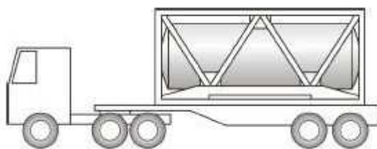
第 12-4 図 被けん引車形式で積載式の移動タンク貯蔵所の例
