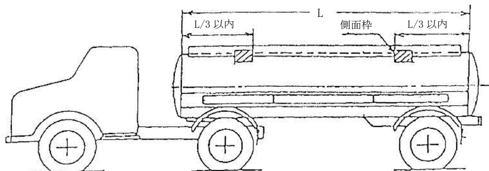
第 12-13 図 被けん引車形式の移動タンク貯蔵所の側面枠の取付位置
