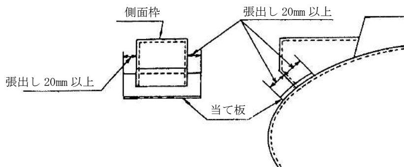
第 12-10 図 箱形の側面枠に設ける当て板の取付方法
