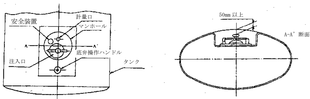
第 12-21 図 防護枠を設けないことができる附属装置が陥没しているタンクの構造
