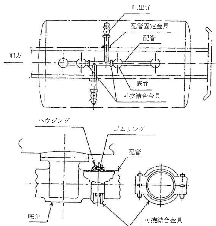
第 12-33 図 緩衝用継手による底弁に直接衝撃が加わらない措置
