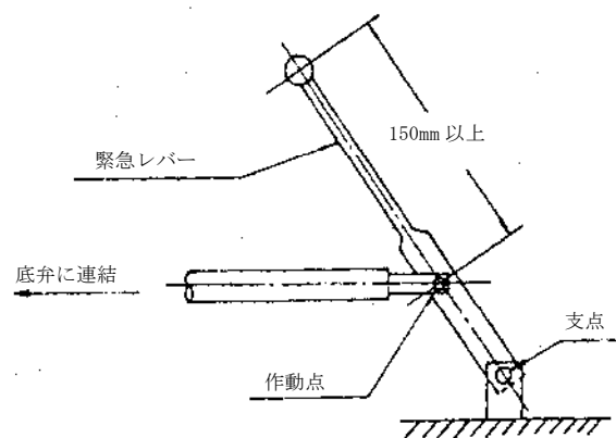
第 12-28 図 緊急レバーの構造
