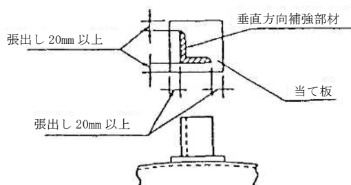
第 12-27 図 補強部材用当て板の大きさ
