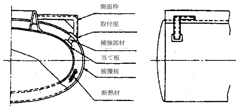
第 12-17 図 被覆板の下部に補強部材を設け、側面枠と補強部材を溶接接合する場合の取付方法
