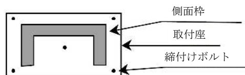
第 12-20 図 1 の締付けボルトに応力集中が発生しない締付け配列方法
