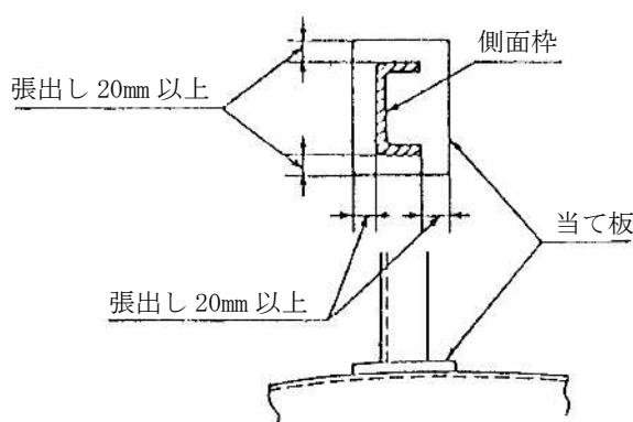
第 12-11 図 枠形の側面枠に設ける当て板の取付方法
