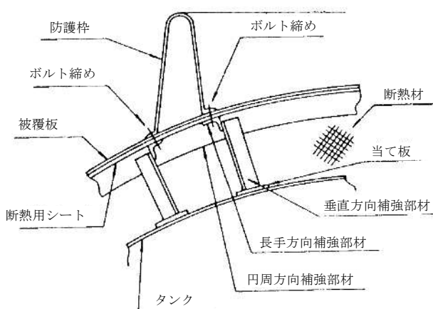
第 12-25 図 被覆板の下部に補強部材を設ける防護枠の接合方法
