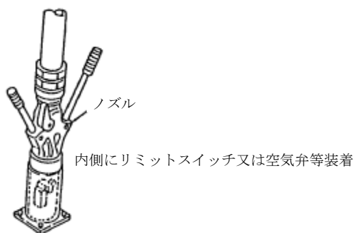
第 12-41 図 ノズル格納装置による誤発進を防止する方法
