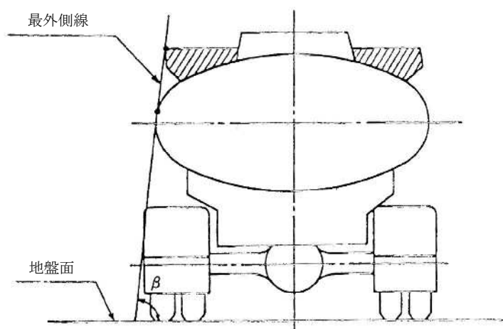
第 12-15 図 最外側線の決定方法
