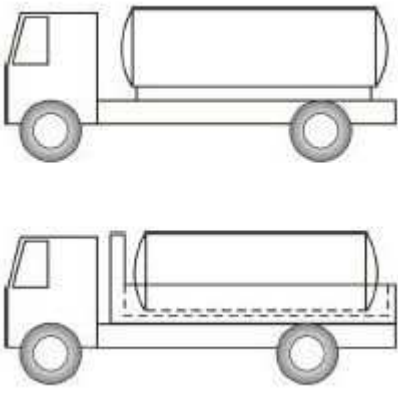
第 12-1 図 単一車形式で積載式以外の移動タンク貯蔵所の例
