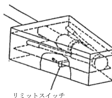
第 12-41 図 ノズル格納装置による誤発進を防止する方法
