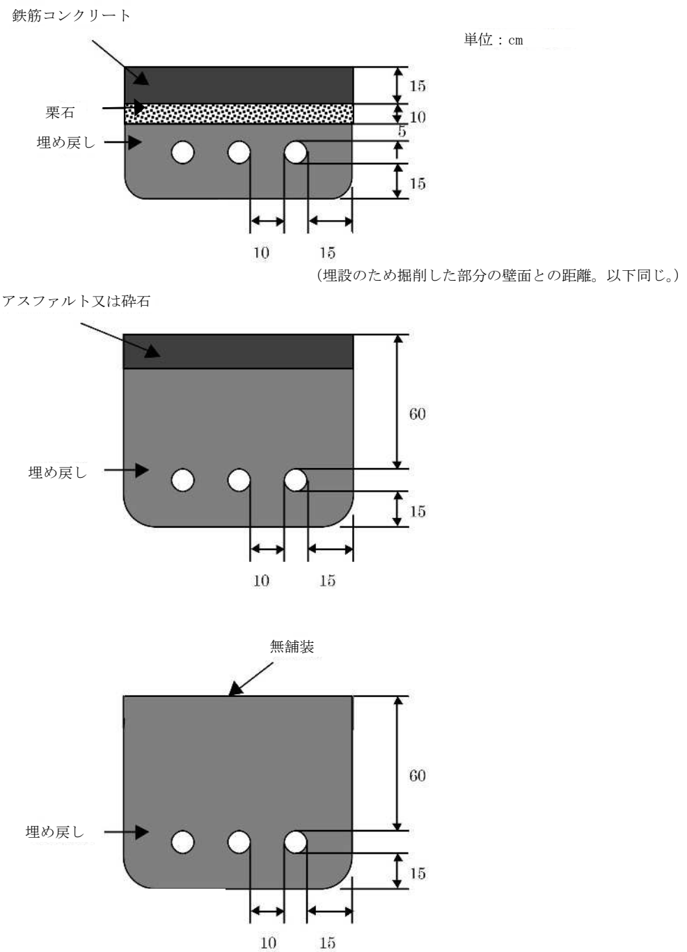
第 2 図 埋没構造例
