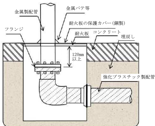
第 1 図 金属製配管と強化プラスチック製配管の接続例
