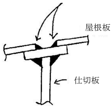
例図 4（片隅肉溶接）
