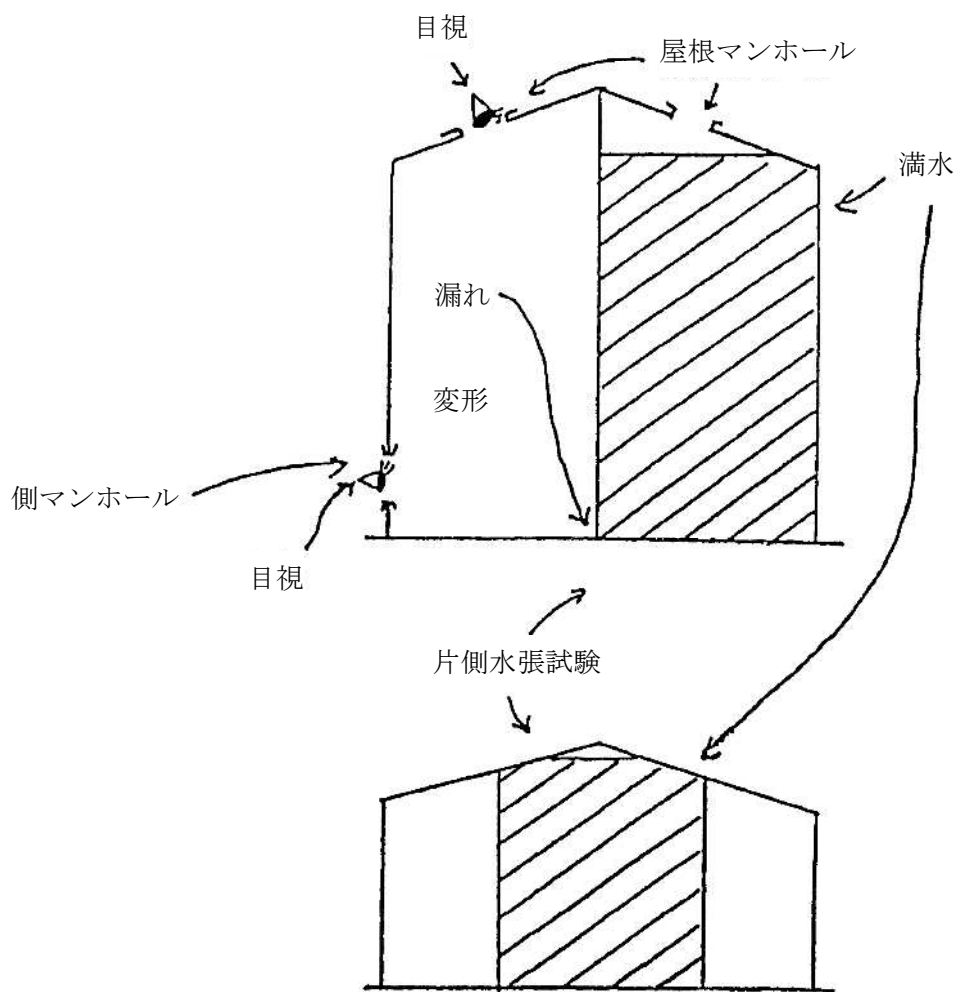
例図 5 (設置方法、検査等の例)
