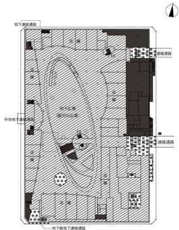
管理区分（地下 1 階平面図）
