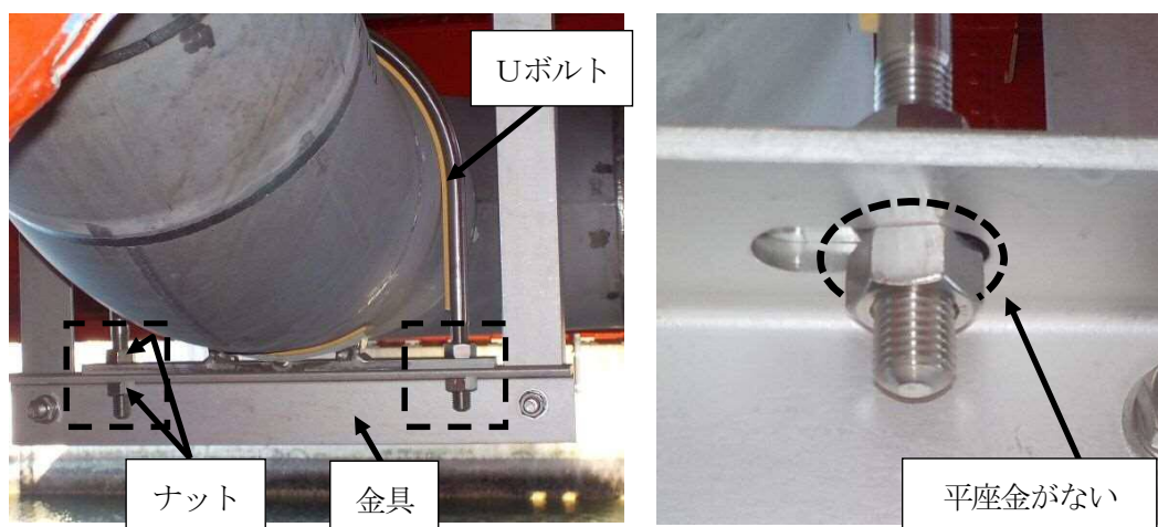
Uボルトとナットの締め付け箇所の状況
