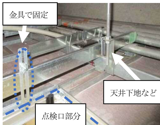
固定された点検口
