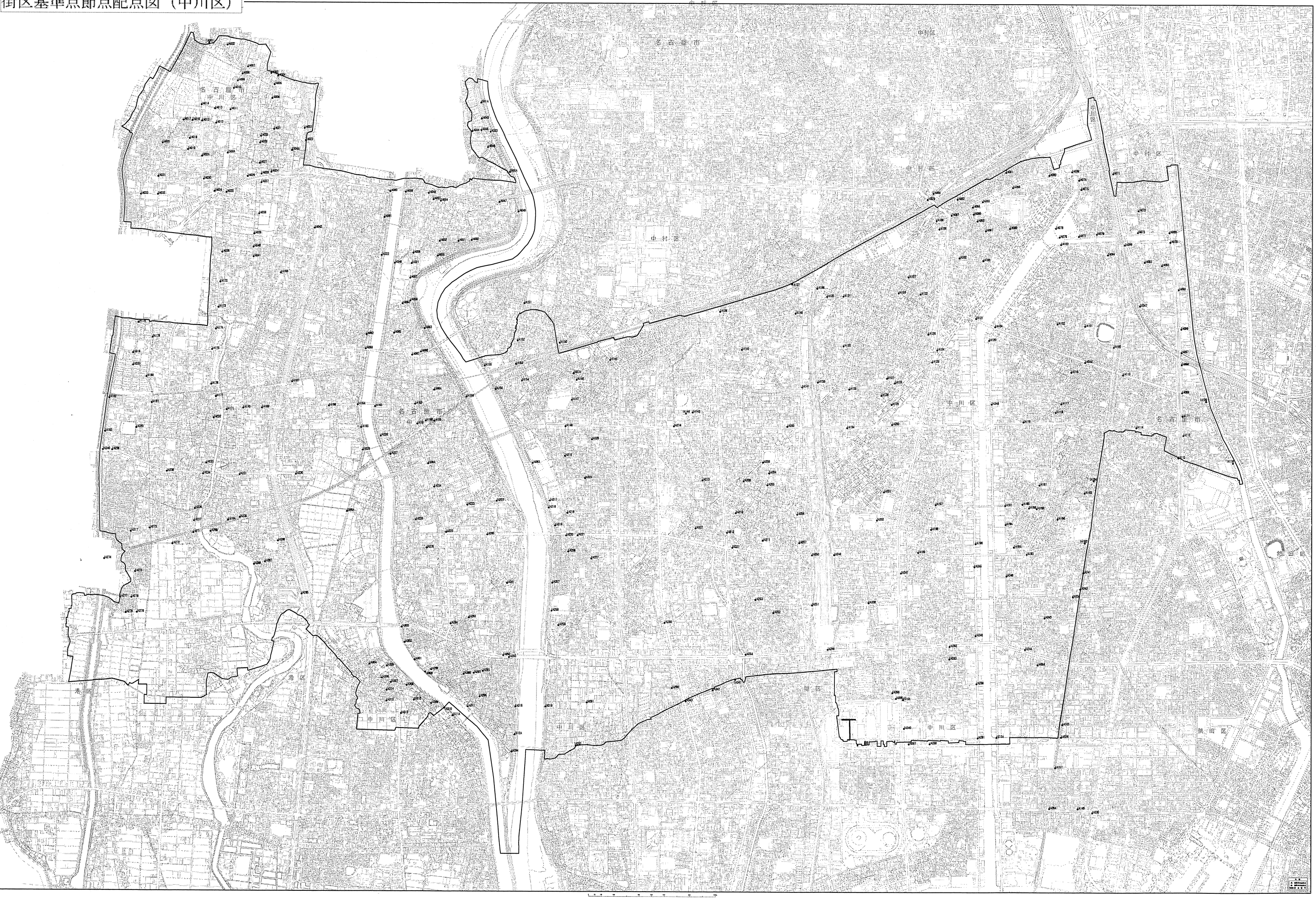
街区基準点節点配点図（中川区）
