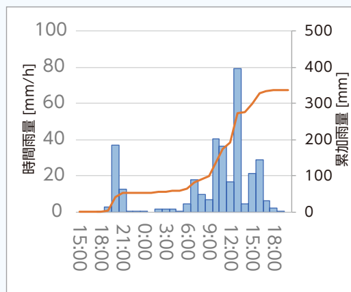
雨量(東谷山)
