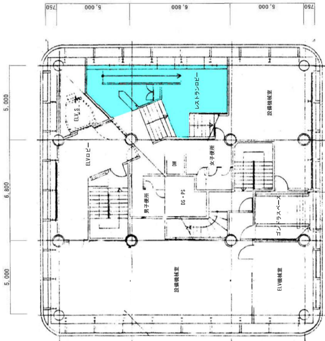
中6階平面図 S=1:100
