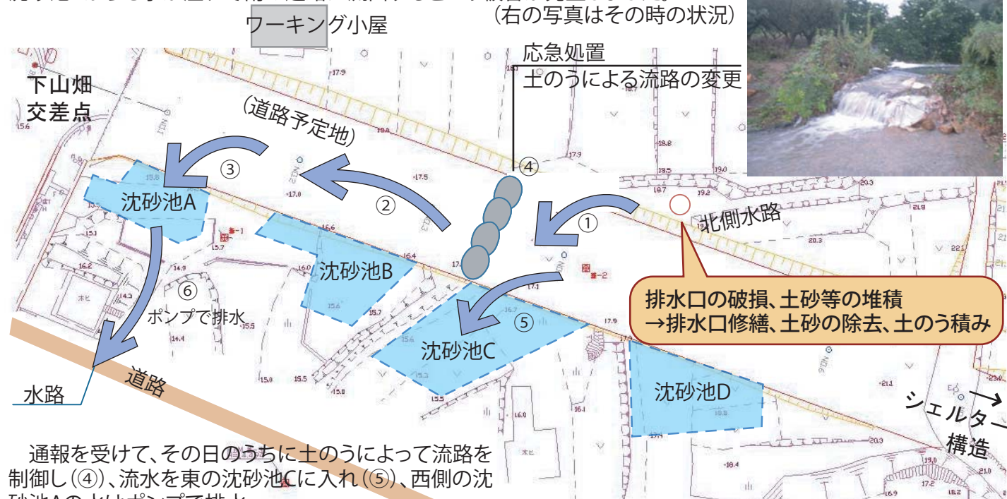
排水口の破損 土砂等の堆積
