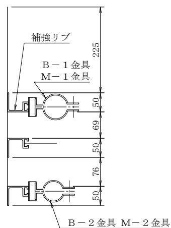
M-2 金具
