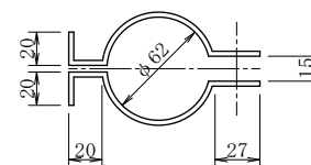
B-1 金具
