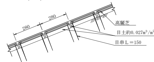
(E') 断面図
