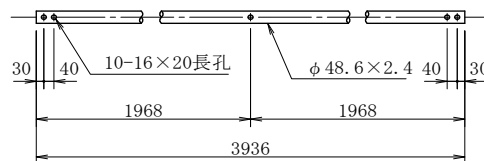
中間部詳細図
