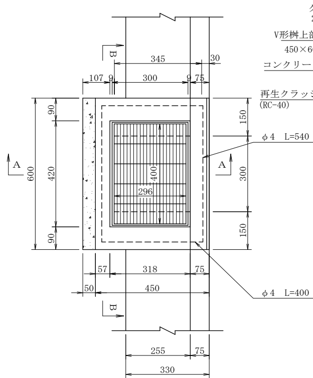
平 面 図
