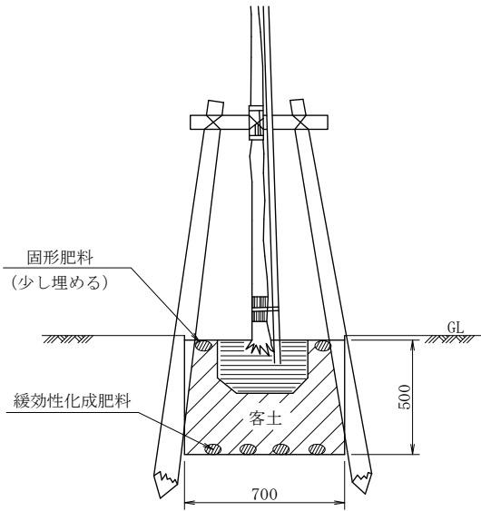
断 面 図
