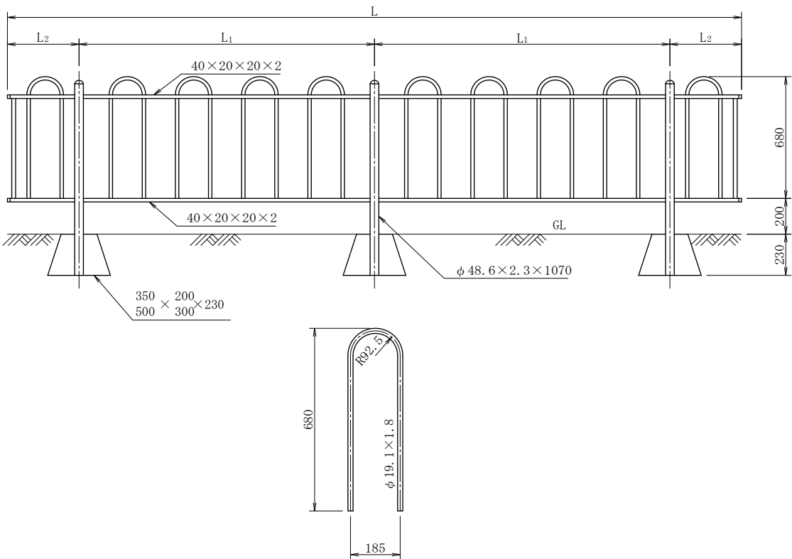
側面図
