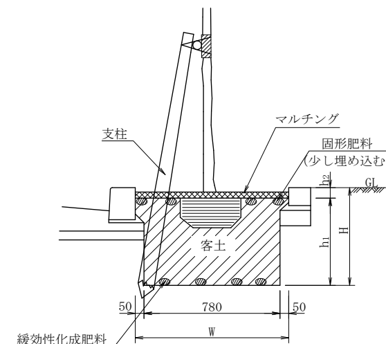
断 面 図
