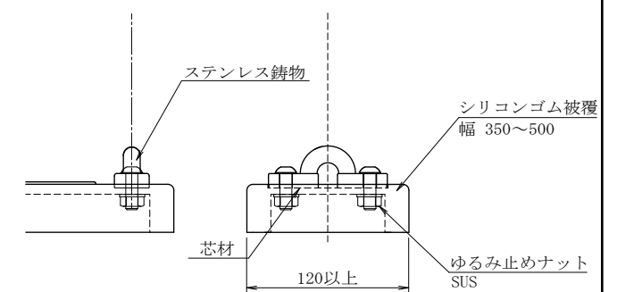
乗板参考図
