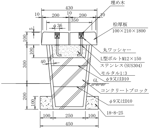
断面図
