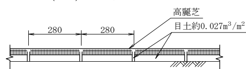
(D') 断面図
