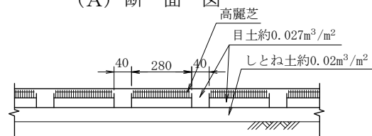
(A) 断面図
