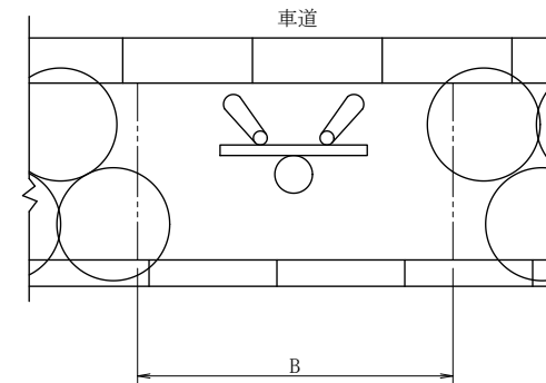
断 面 図
