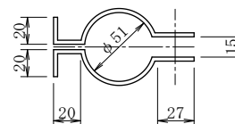
B-2 金具
