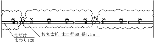
正面図
