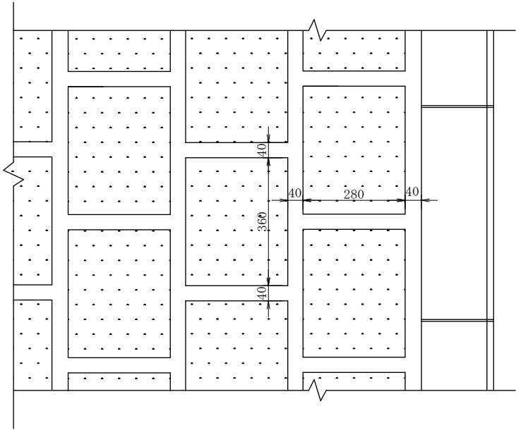
平 面 図
