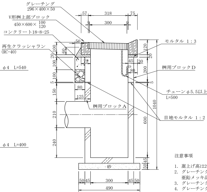
A-A 断 面 図
