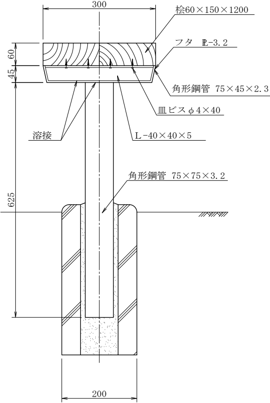
側面図
