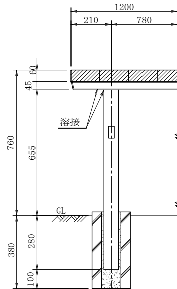
正 面 図
