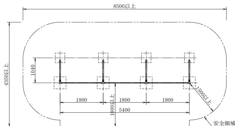
平面图
