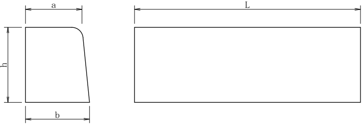
片面歩車道境界ブロック
