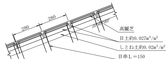
(E') 断面図
