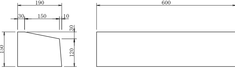
ブロック寸法
