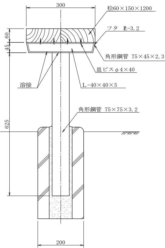
側面図
