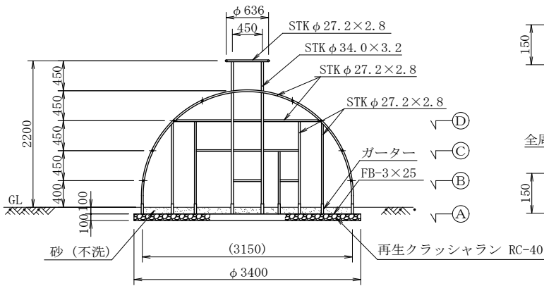
側 面 図
