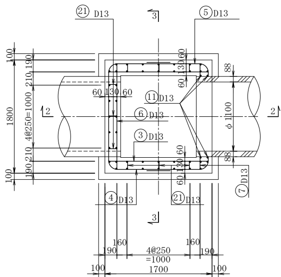
1 - 1 断 面
