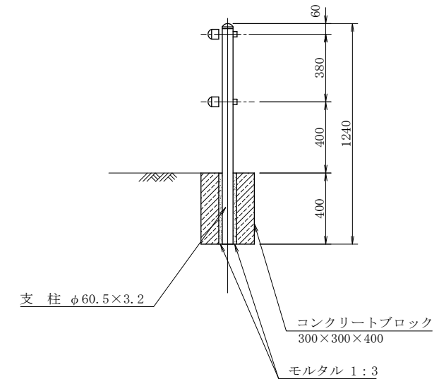
コンクリートブロック
