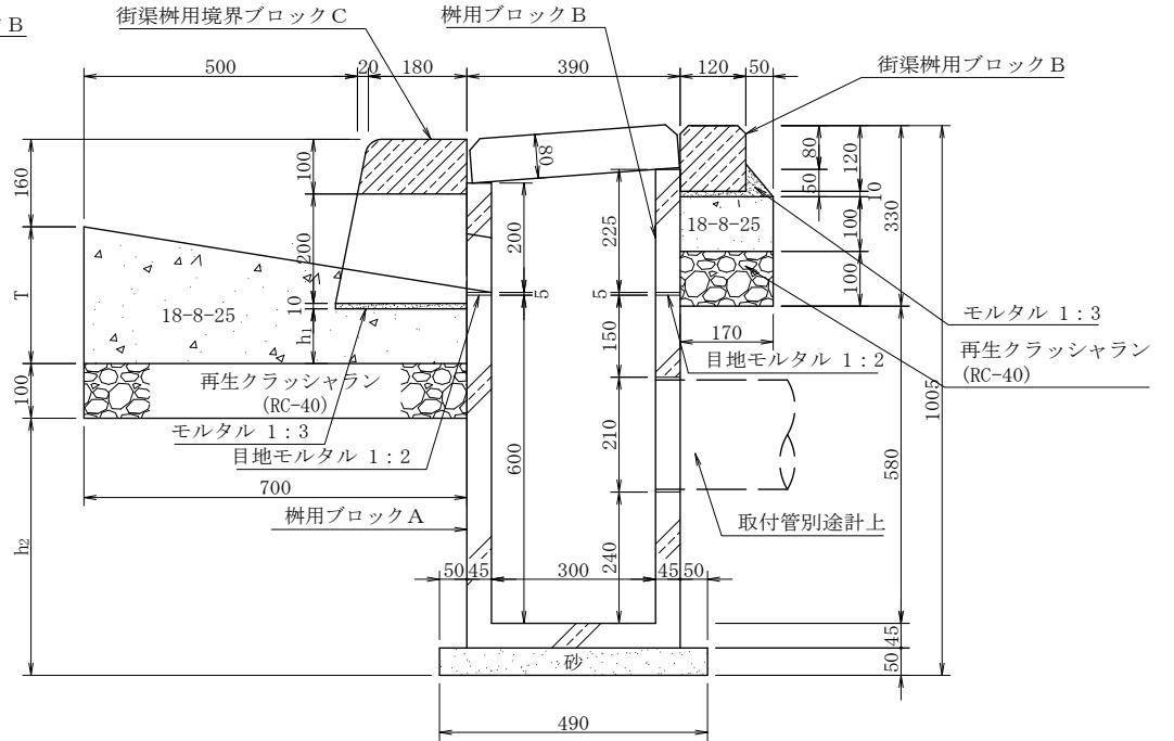
A-A 断面図
