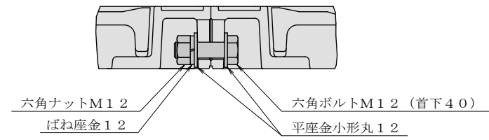
C - C 断面詳細図
