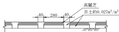
(A') 断面図
