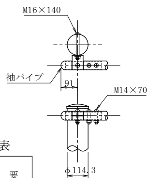
端部詳細図
