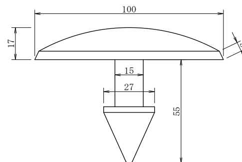
測量標(水準点・多角水準点)設置工材料表
