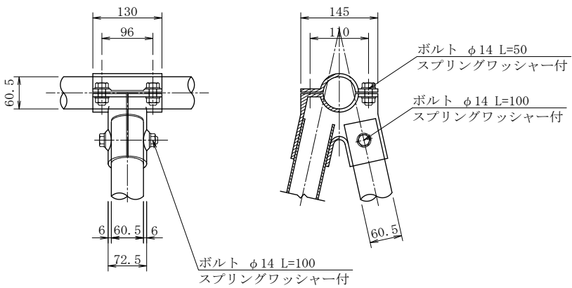
鋳鉄角岐金具詳細図
