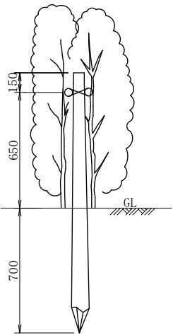
断 面 図
