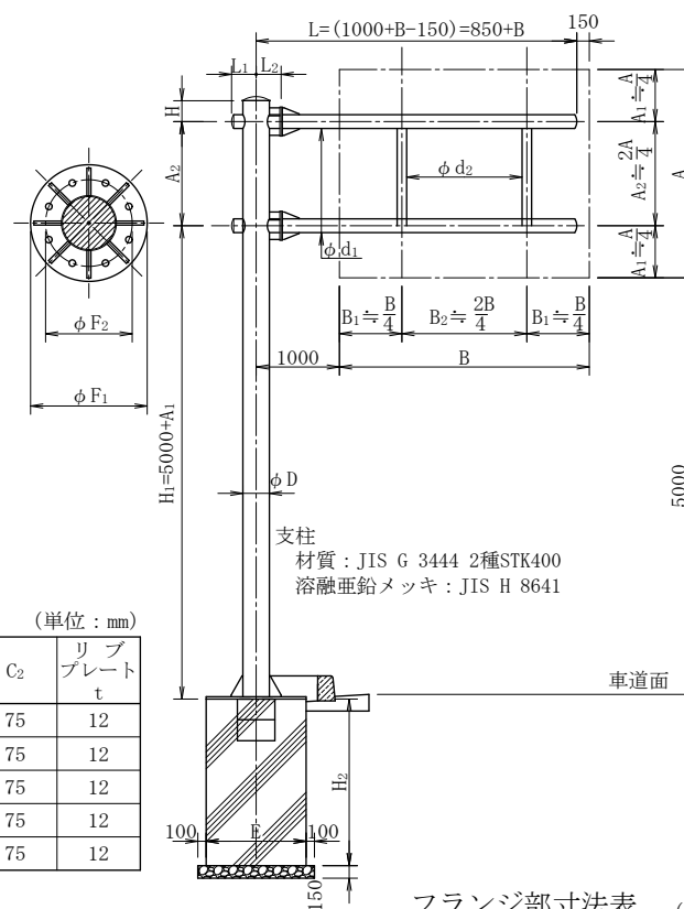
フランジ部寸法表 (単位: mm)
