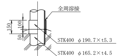
① 地際補強図
