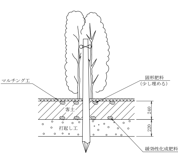
断 面 図
