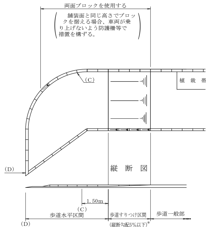
平面図
