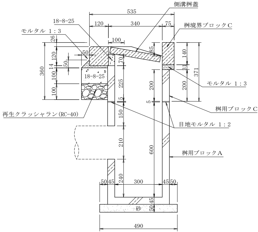
A-A 断 面 図
