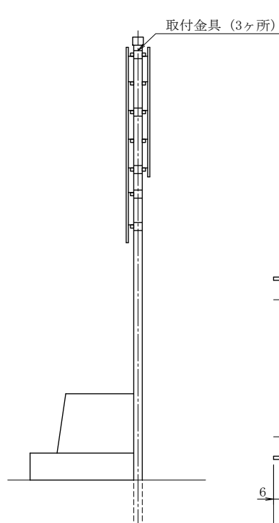
取付金具
