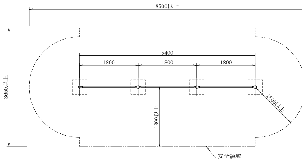
平面图
