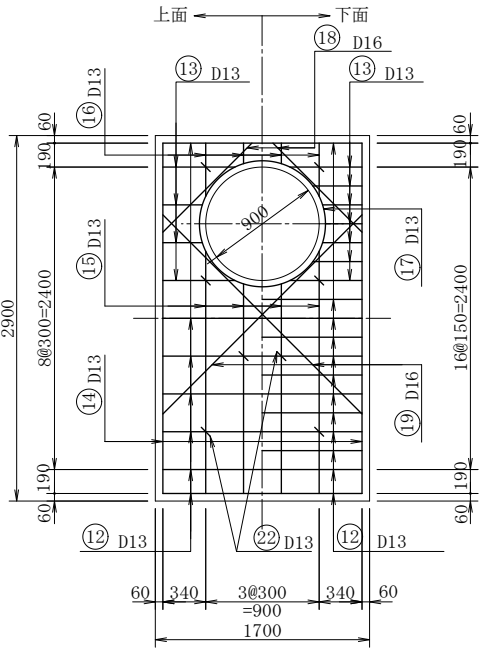
頂 版
