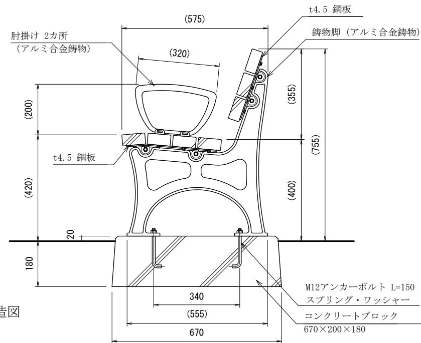
断面図
