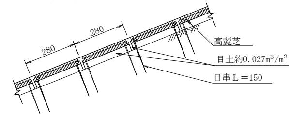
(E') 断面図
