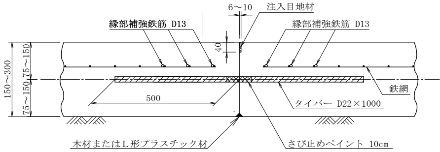
ダ ミ ー 目 地
