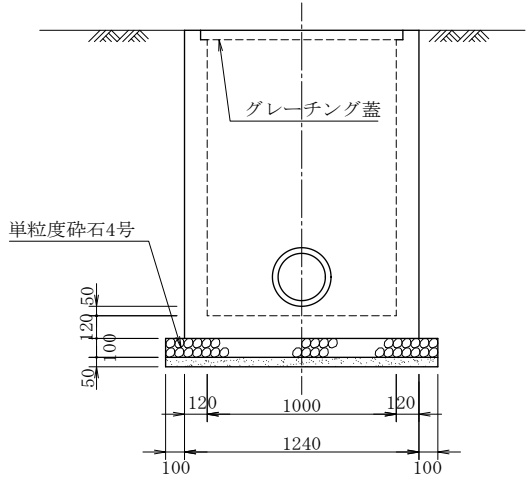
C-C 断面図
