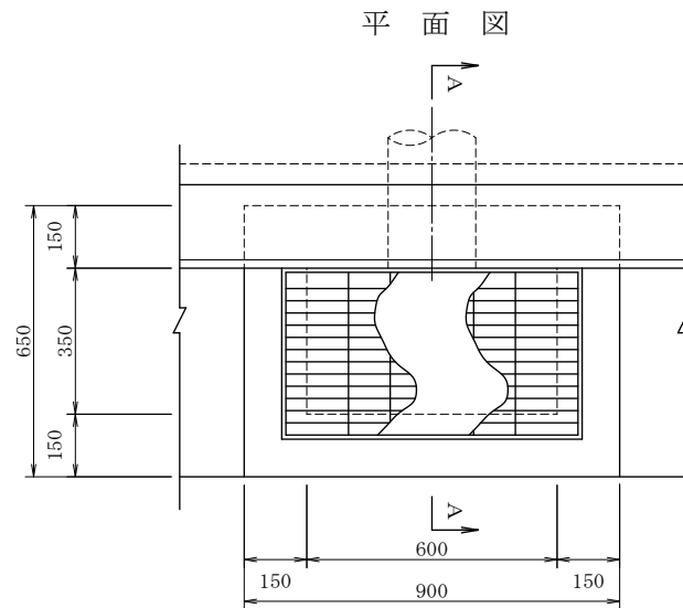
特殊街渠枋寸法表
