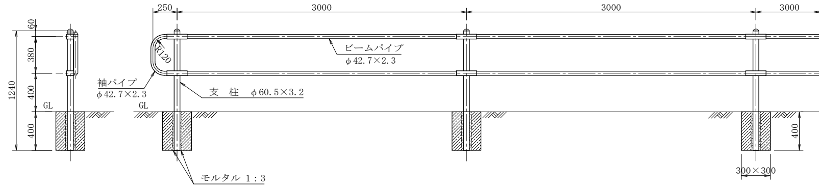
側 面 図
