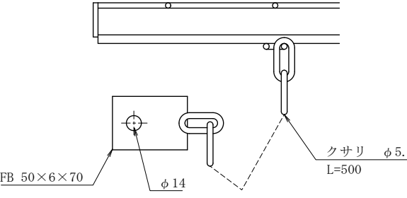
細目用クサリ・FBアンカー詳細
