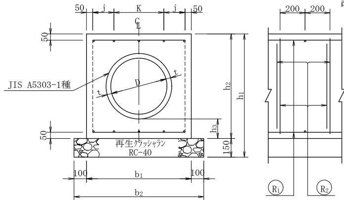
P3型（管きょ：360°固定基礎）寸法および材料表
