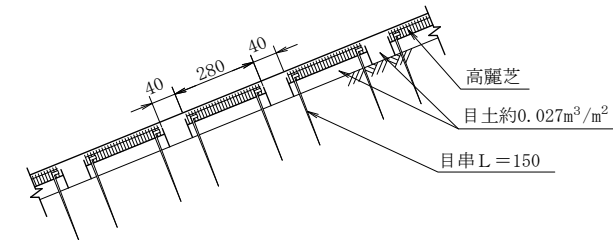
(B') 断面図
