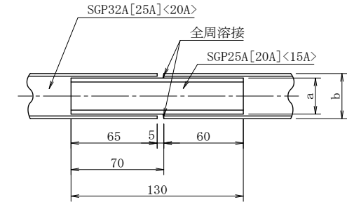
伸縮継手詳細図
