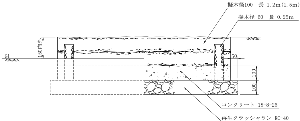
立 面 图
