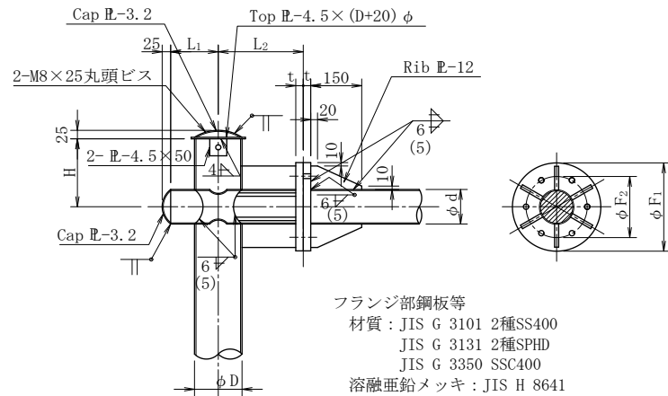
フランジ部詳細図
