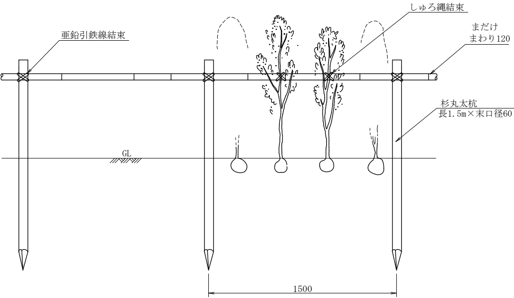
側 面 図
