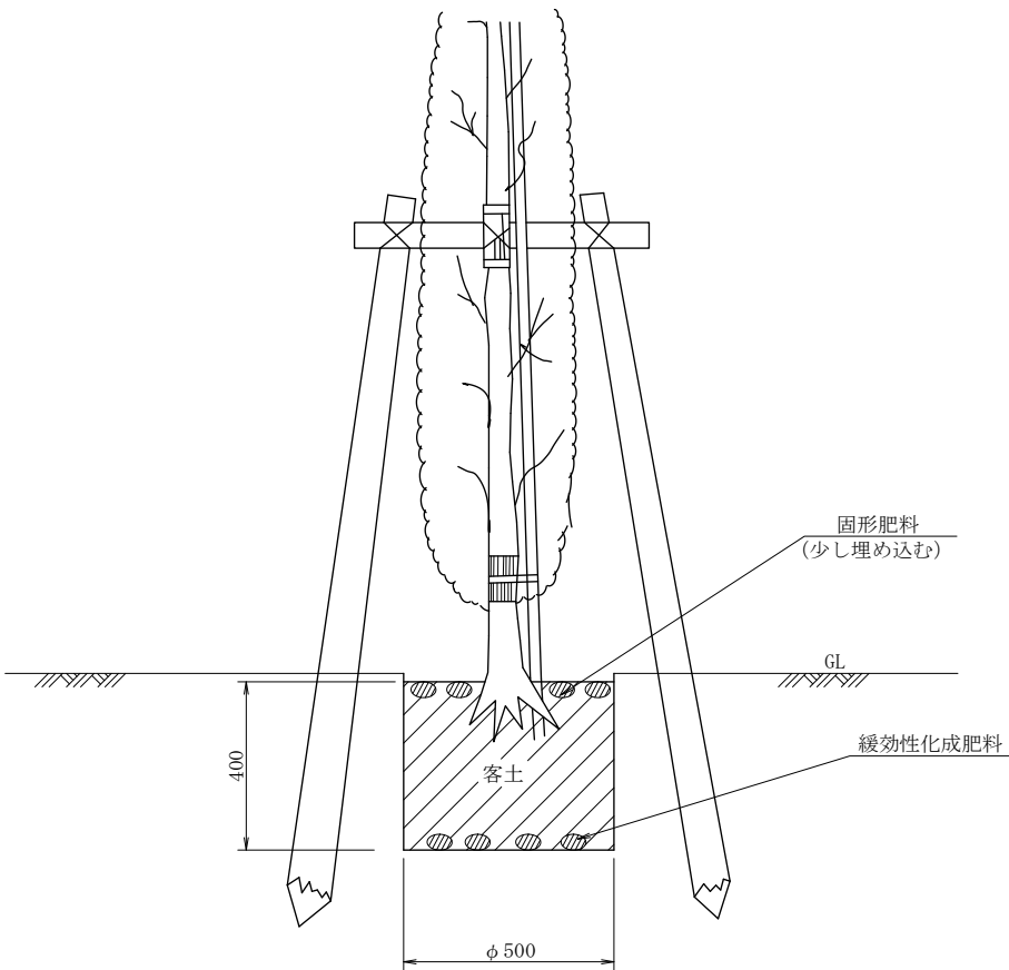
断 面 図
