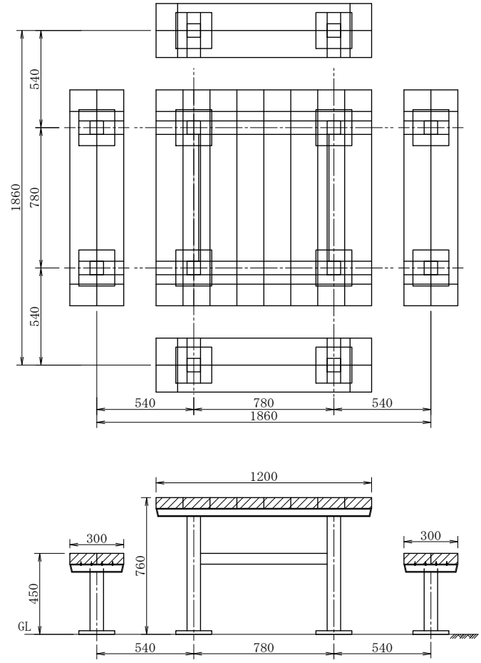
ベンチD・テーブルD位置図
