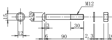
取付ボルト
