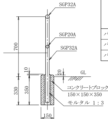
断面図 H=0.7m
