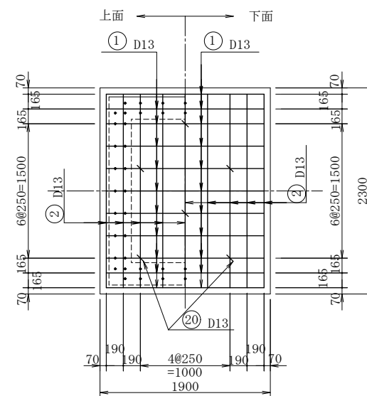
底 版
