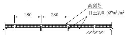
(D') 断面図
