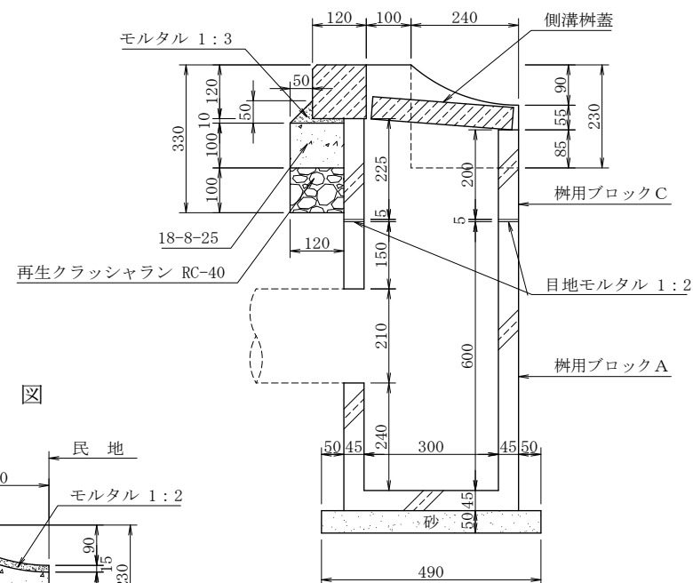
A-A 断 面 図
