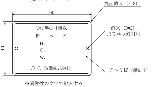
支柱プレート
