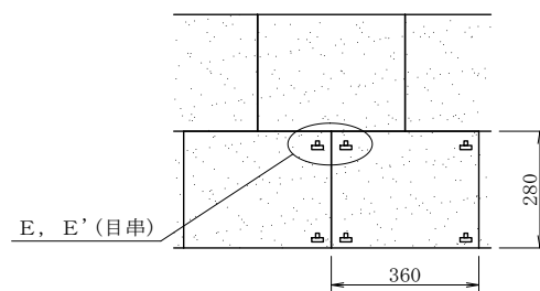
D・E 平面図
