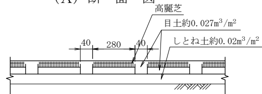
(A) 断面図
