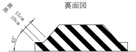
(塗 装 構 成)
