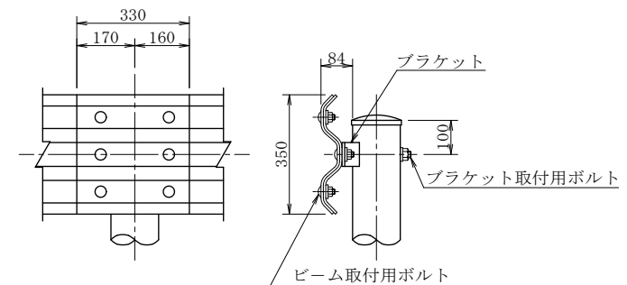
取付詳細図
