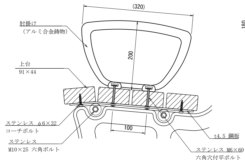
取合詳細図
