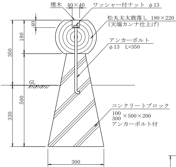
断 面 図
