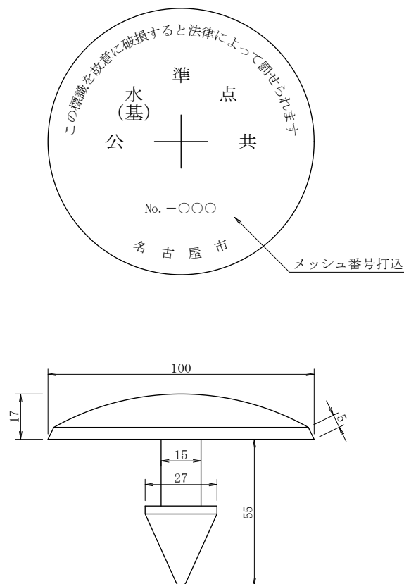
測量標(水準点・多角水準点)設置工材料表
