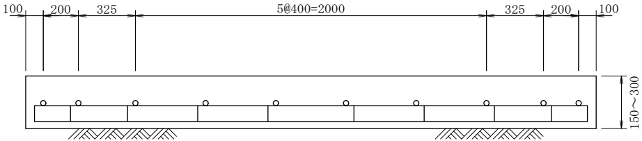
断 面 図
