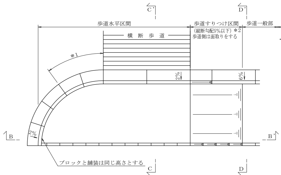
平面図
