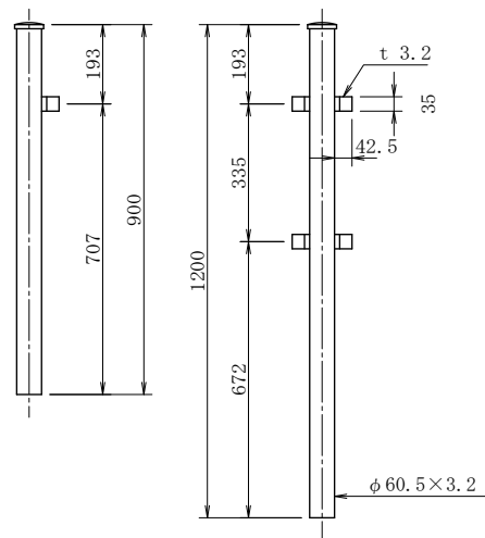
支柱
