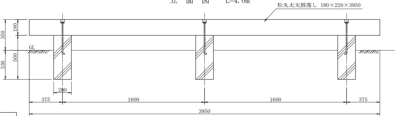
立 面 図 L=4.0m
