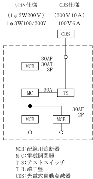
分電盤内結線図
