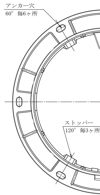
② 受枠平面図
