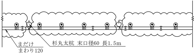
正面図
