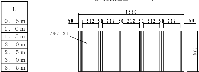
標識板裏面図 S=1/30
