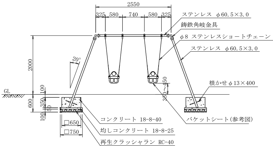
正 面 図
