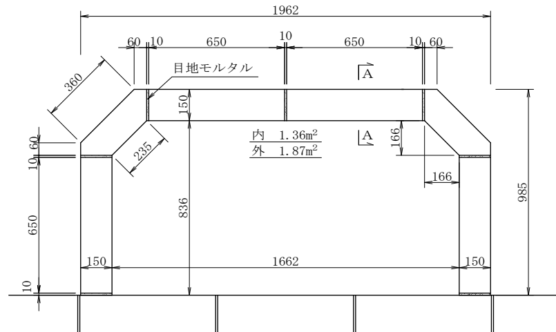
C 平 面 図
