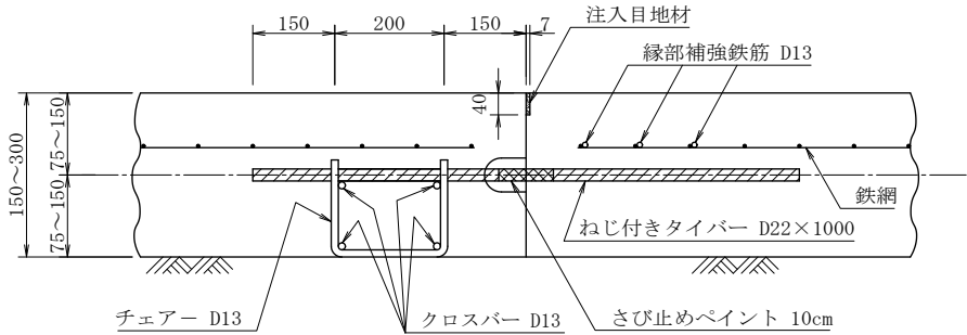
突 合 せ 目 地
