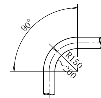
曲部詳細図
