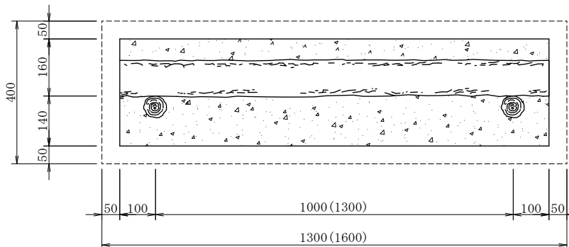
平 面 図
