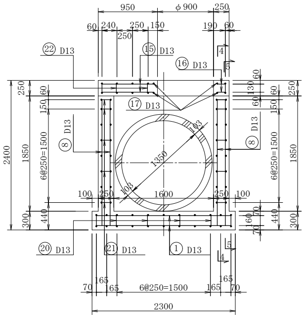
3 - 3 断 面
