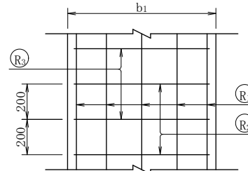
P3型（管きょ：360°固定基礎）寸法および材料表
