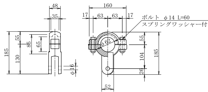
鋳鉄回転軸詳細図
