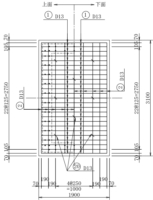
底 版
