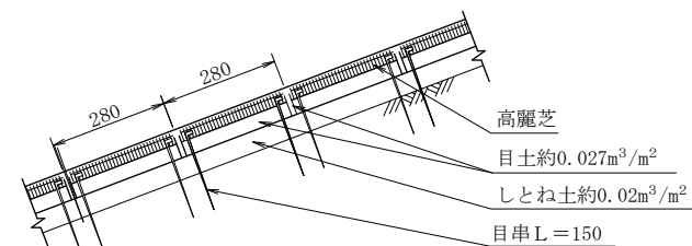
(E') 断面図
