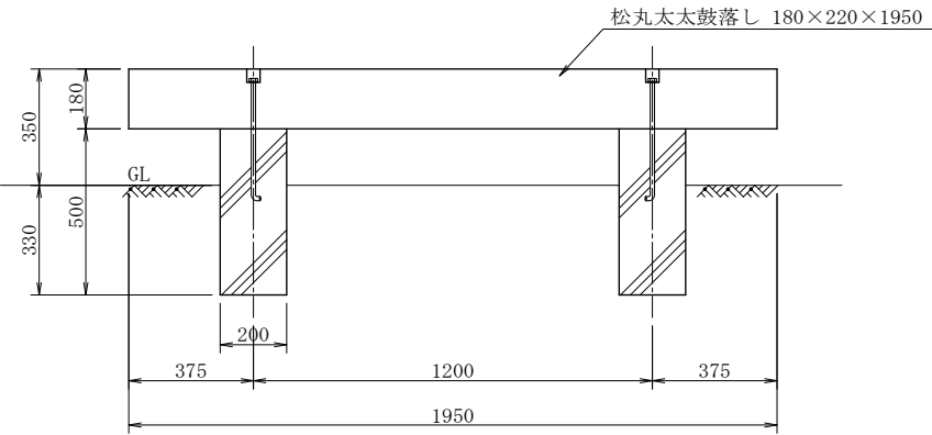
立 面 図 L=2.0m
