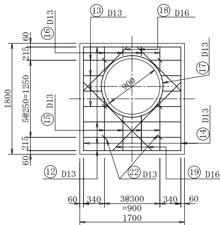
頂 版 上・下面共通
