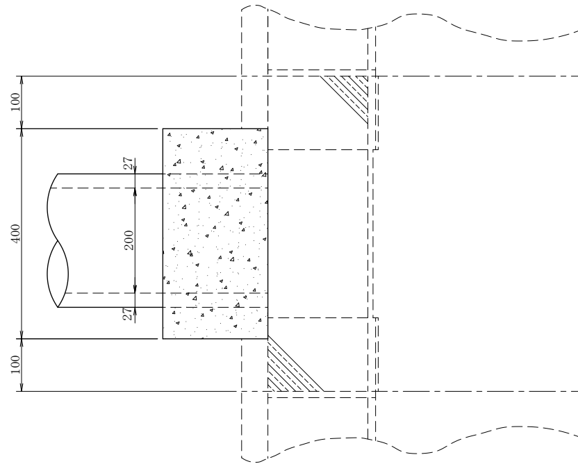
平 面 図
