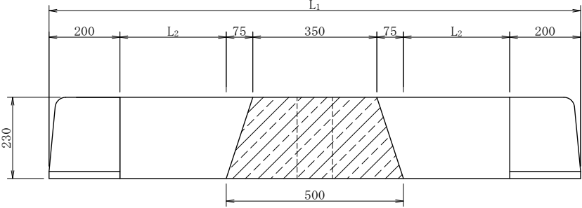
断面図
