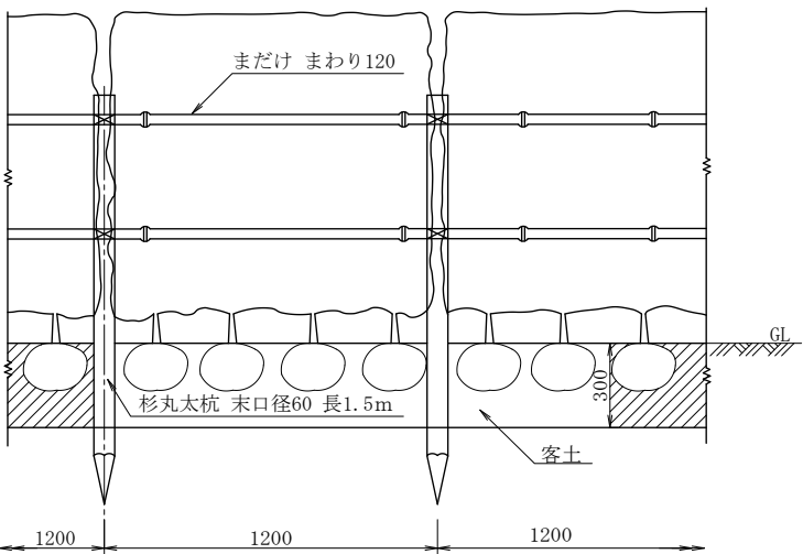
正面図
