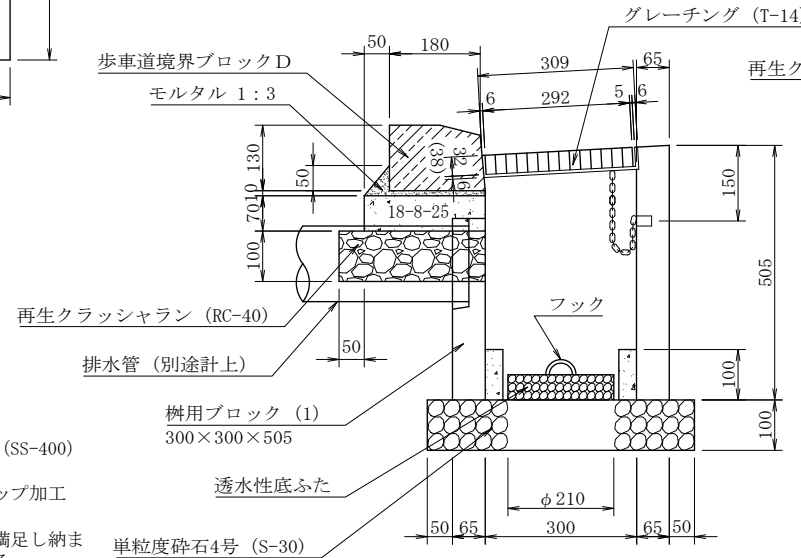
A-A 断面図
