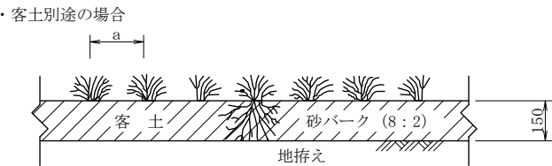
公園地被客土工
