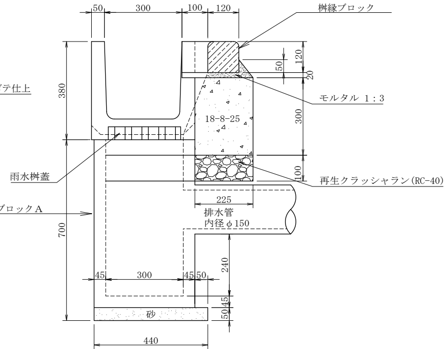
A-A 断面図
