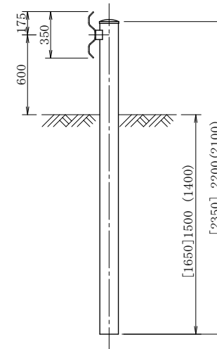
支柱
