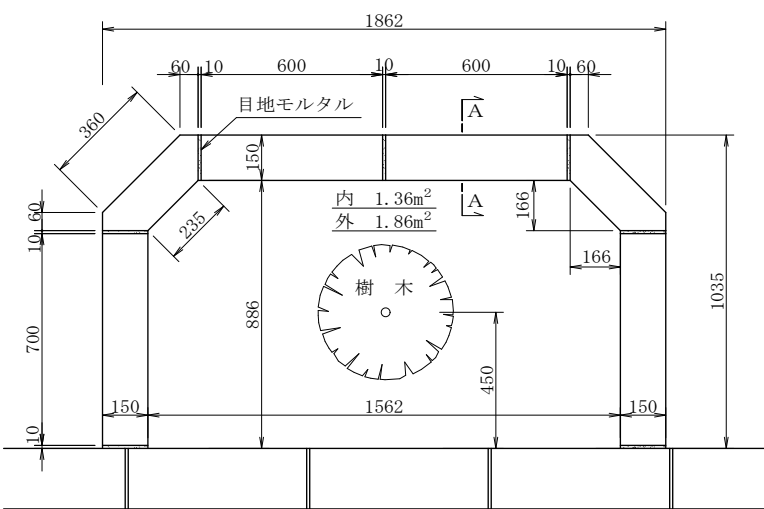
A 平 面 図
