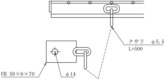
並目用クサリ・FBアンカー詳細
