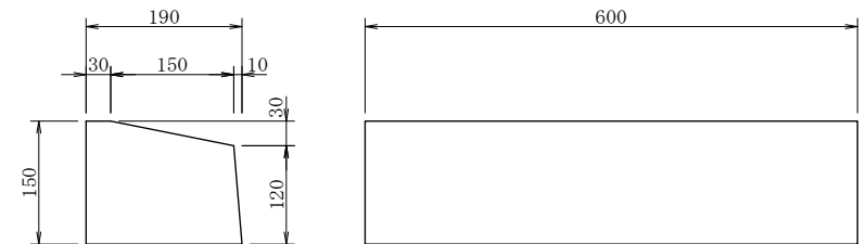
ブロック寸法
