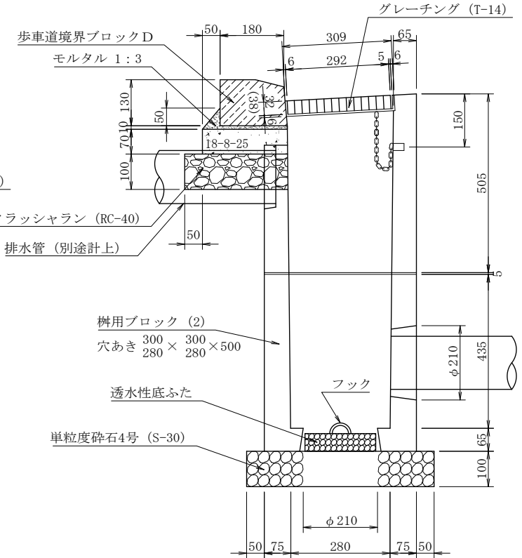
A-A 断面図
