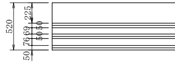
案内標識板 (裏面)
