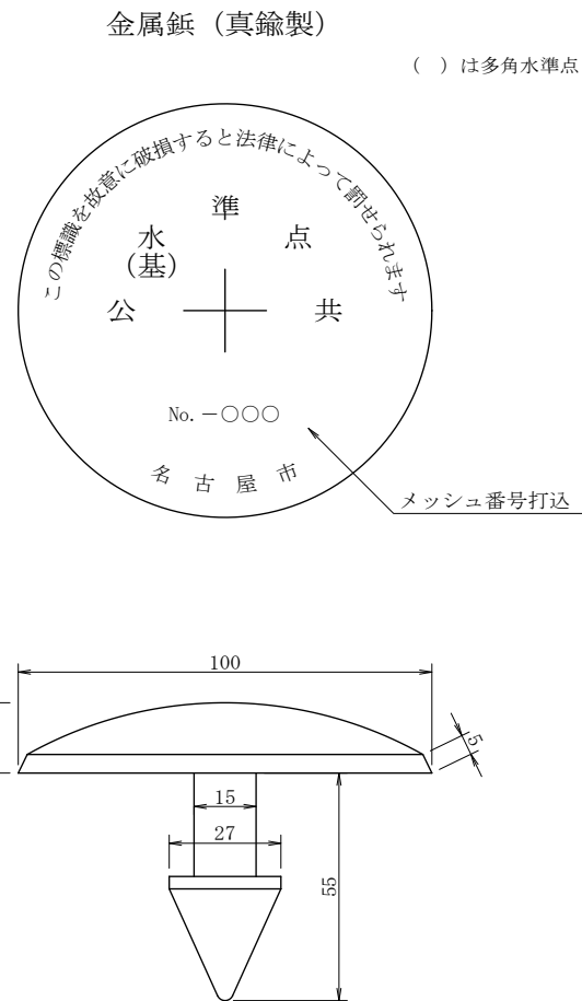
測量標(水準点・多角水準点)設置工材料表
