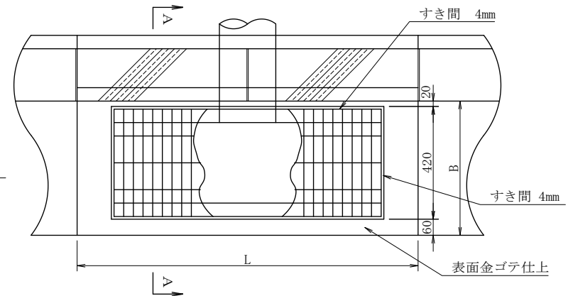
名 称 寸 法 表 単位 (mm) 摘 要 B b 1 b 2 b 3 b 4 H h 1 h 2 h 3 h 4 h 5 t t 1 t 2 L 街渠櫛工 500B用 現 場 打 560 205 255 600 700 1270 250 150 210 120 1050 150 90 50 1270 ブロック 500 205 255 540 640 1240 250 150 240 120 1020 120 60 20 1210 街渠櫛工 500C用 現 場 打 560 210 260 600 700 1320 300 200 210 170 1050 150 90 50 1270 ブロック 500 210 260 540 640 1290 300 200 240 170 1020 120 60 20 1210 街渠櫛工 500A用 ブロック 500 170 220 540 640 1240 200 150 240 120 1020 120 60 20 1210
