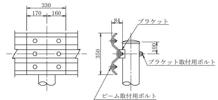
取付詳細図
