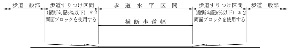
A-A' 断面
