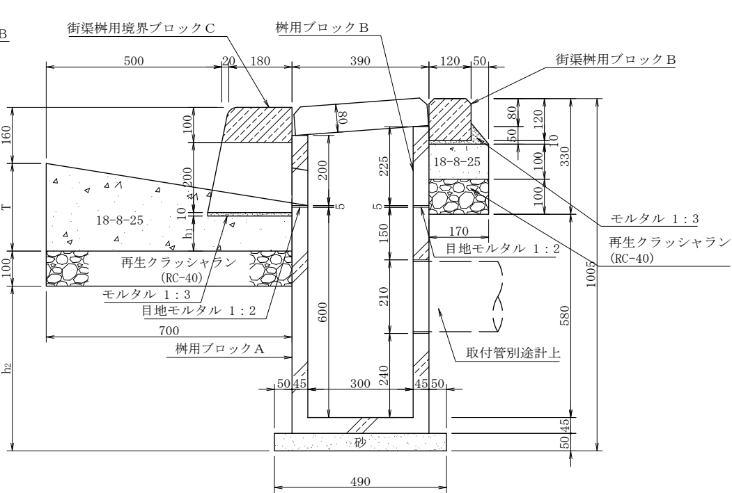
A-A 断面図
