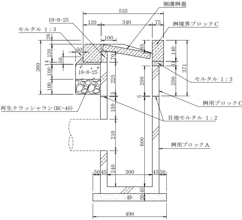
A-A断面図
