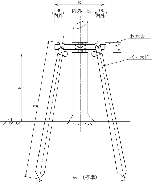
正 面 図
