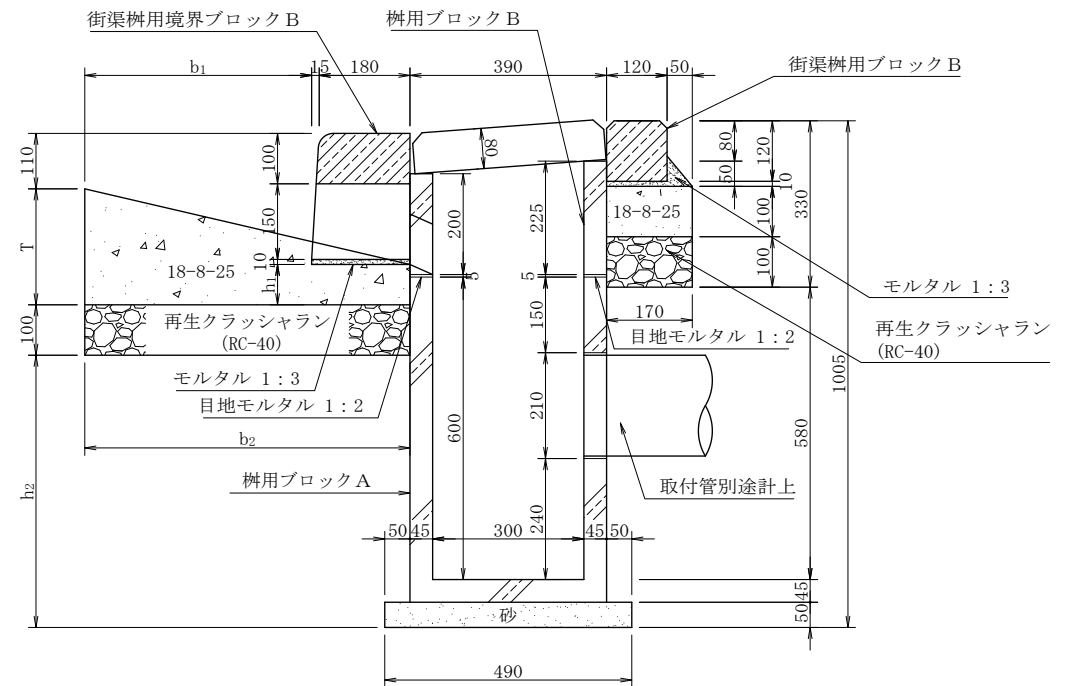
A-A 断面图
