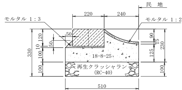
特殊柵工 A 材料表
