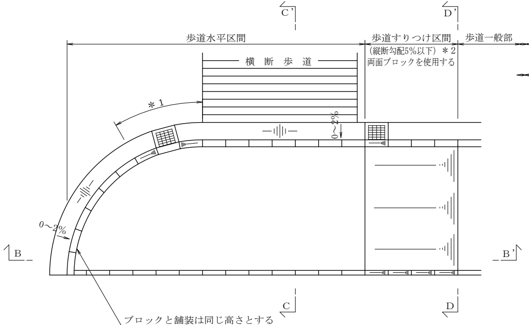
平面図
