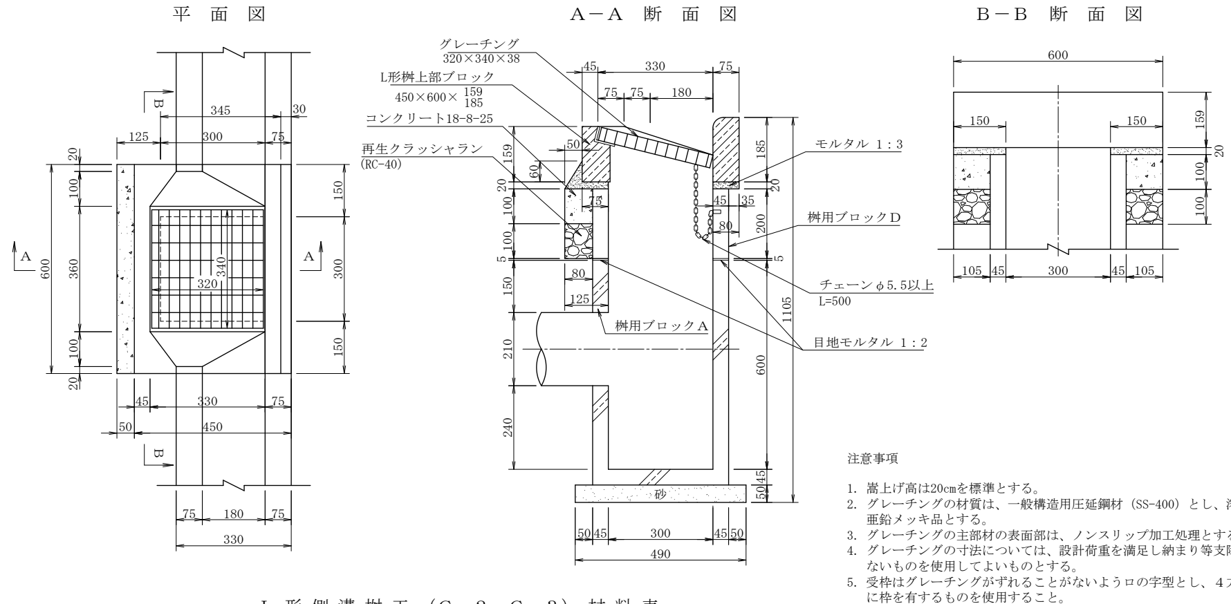
L 形側溝柵工（C-2, C-3）材料表
