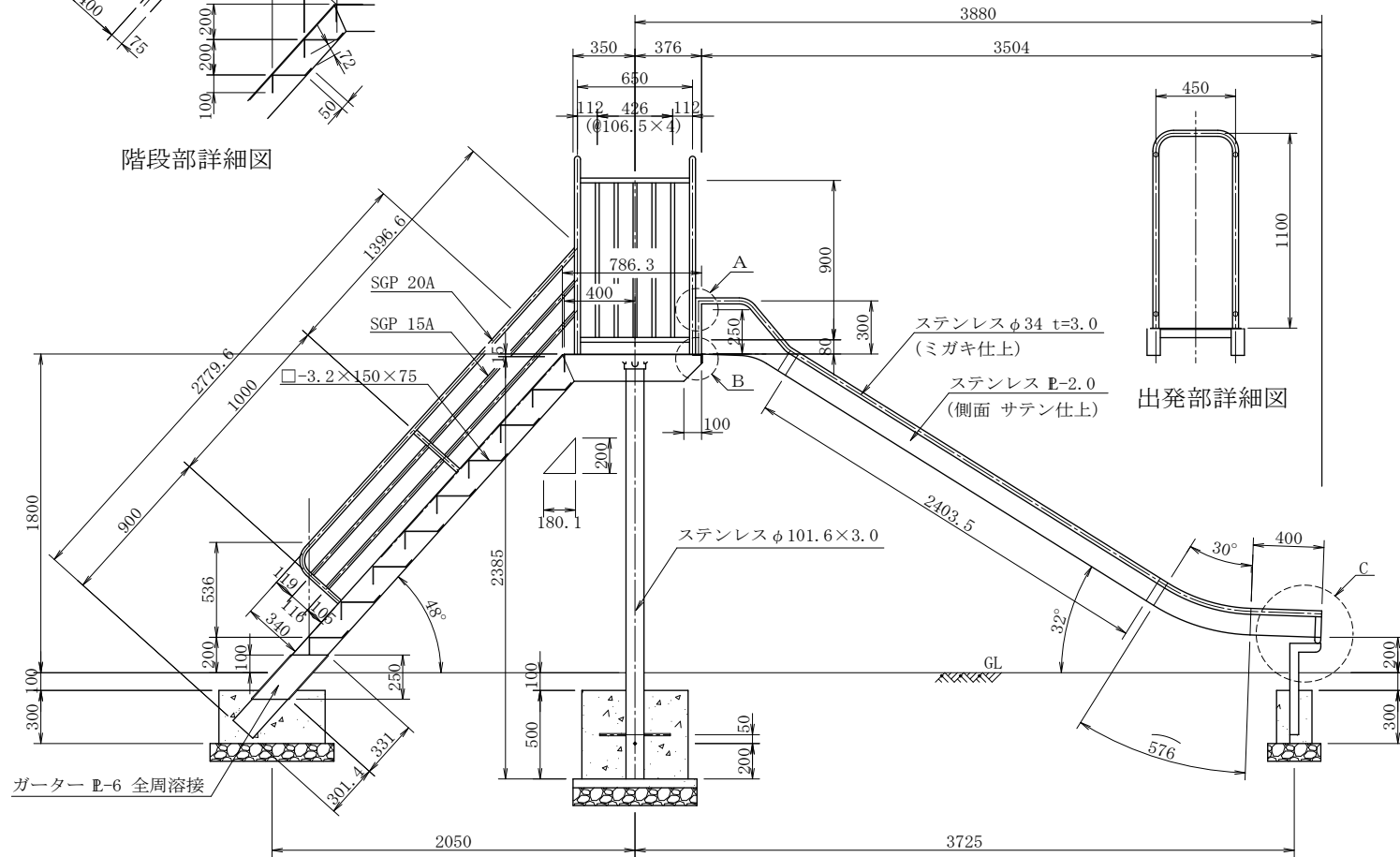
立面詳細図
