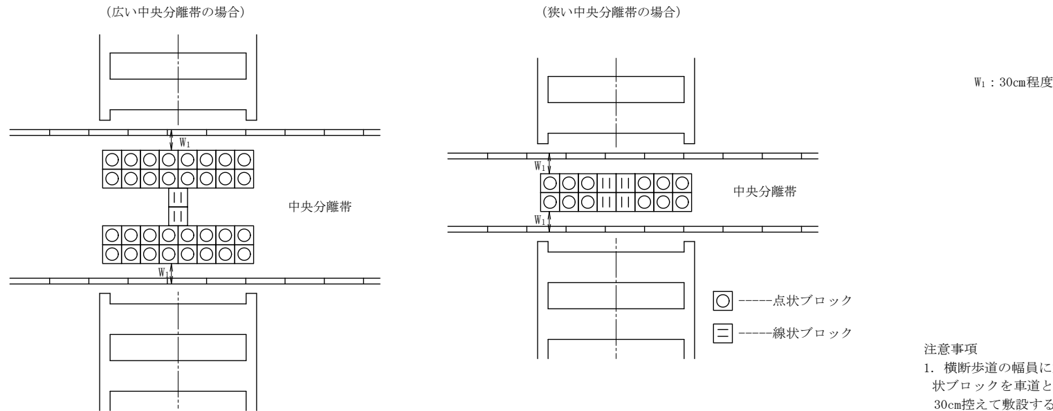
配列図 E (中央帯部)
