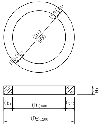
上部ブロック受口（1号丸）
