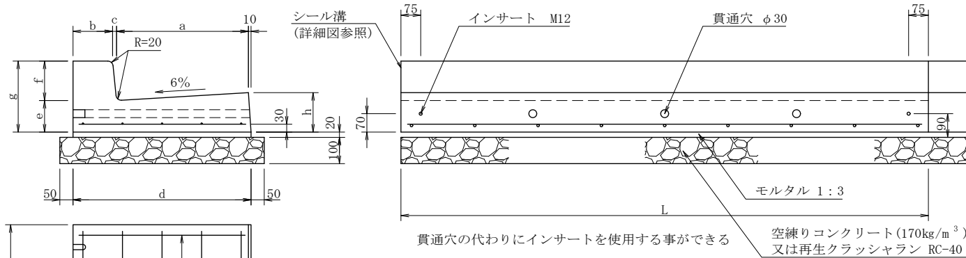
ジョイント部詳細図
