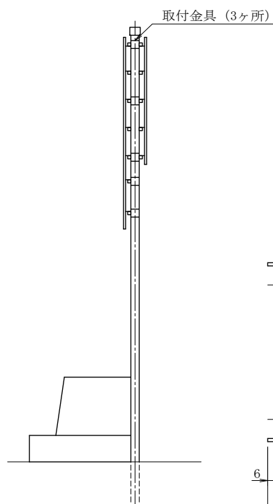
取付金具
