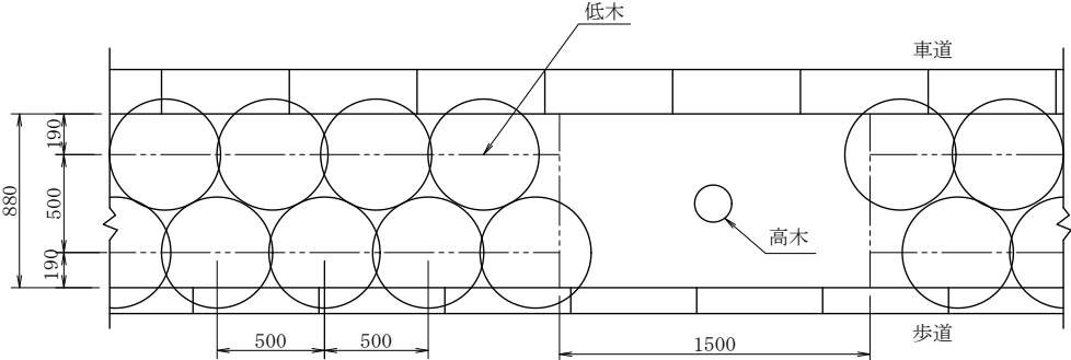
標準平面図
