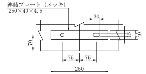
連結部詳細図
