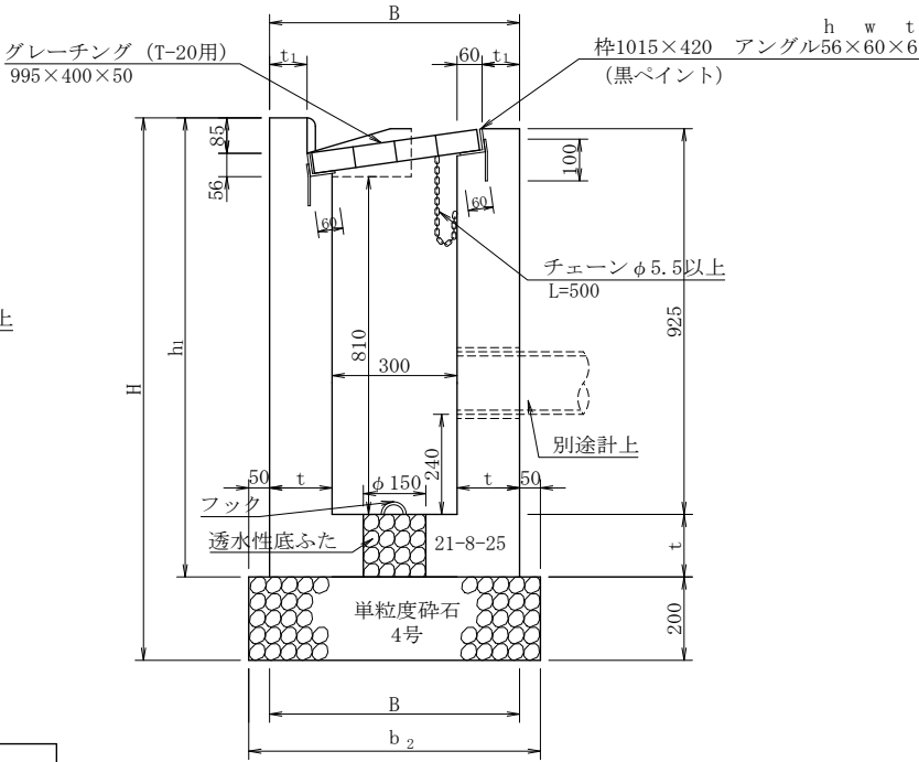
A-A 断 面 図
