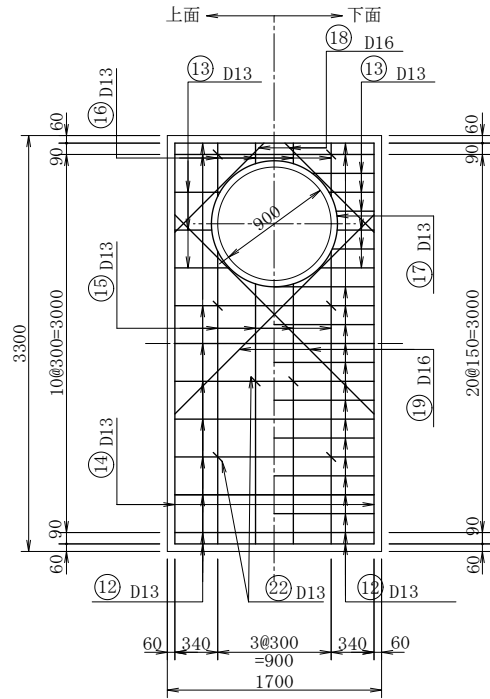
頂 版
