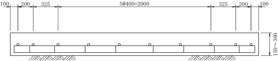
断 面 図
