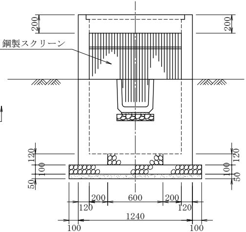
B-B 断面図
