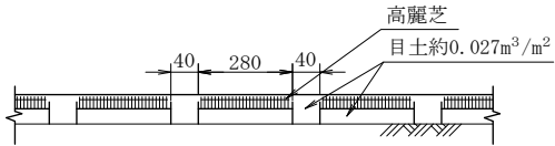
(A') 断 面 図
