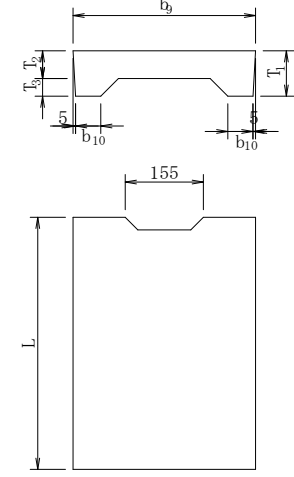
U形側溝B用ふた
