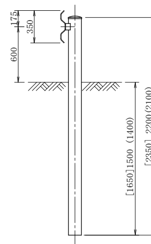
支柱
