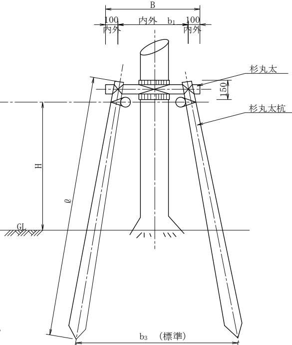
正 面 図
