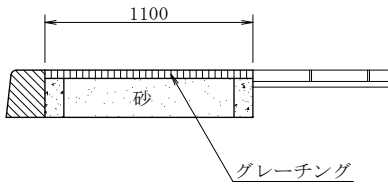
B－B 断 面 図
