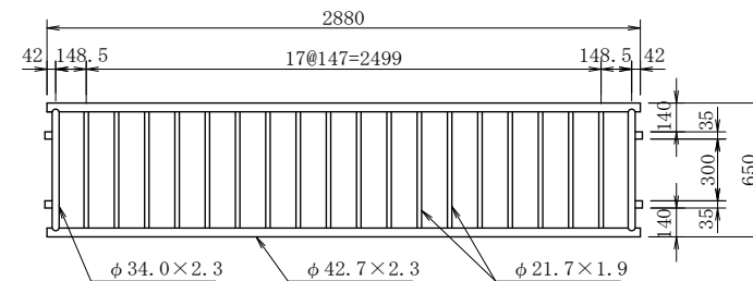
パネル詳細図 (中間パネル)
