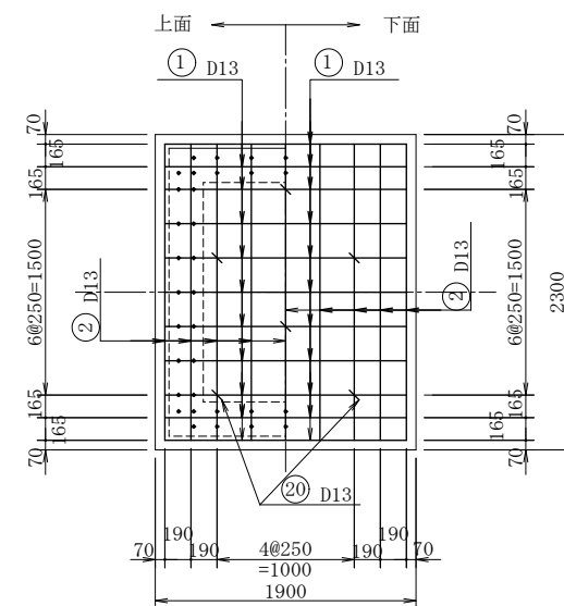
底 版
