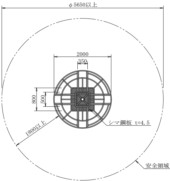
平 面 図
