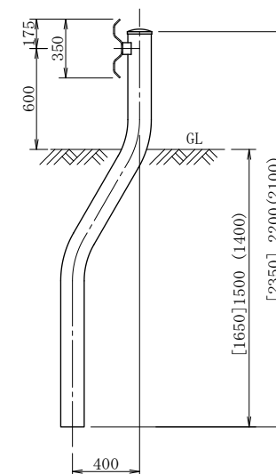
曲柱
