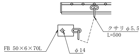
並目用クサリ・FBアンカー詳細
