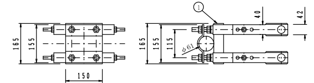
取付金具詳細図 S=1/15 溶融亜鉛メッキ仕上げ
