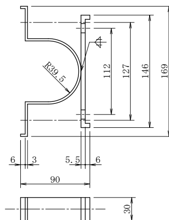
取付金具
