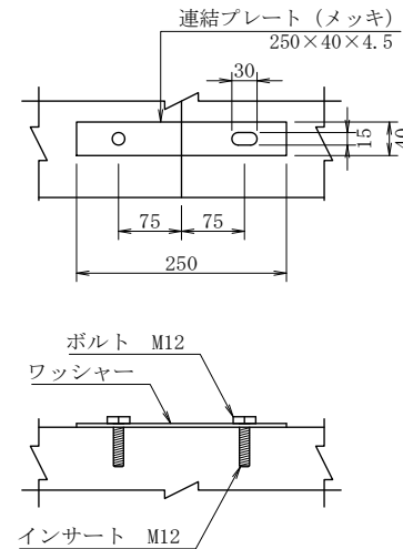
連結部詳細図
