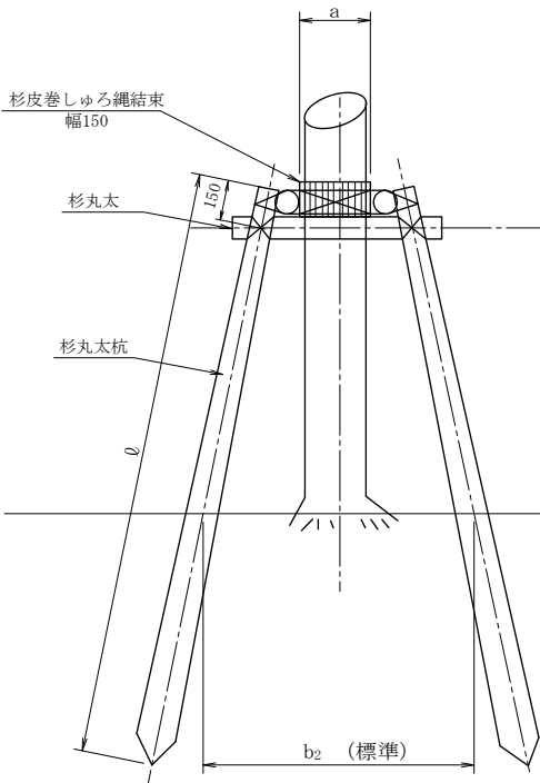
側 面 図
