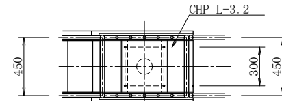
デッキ部平面図
