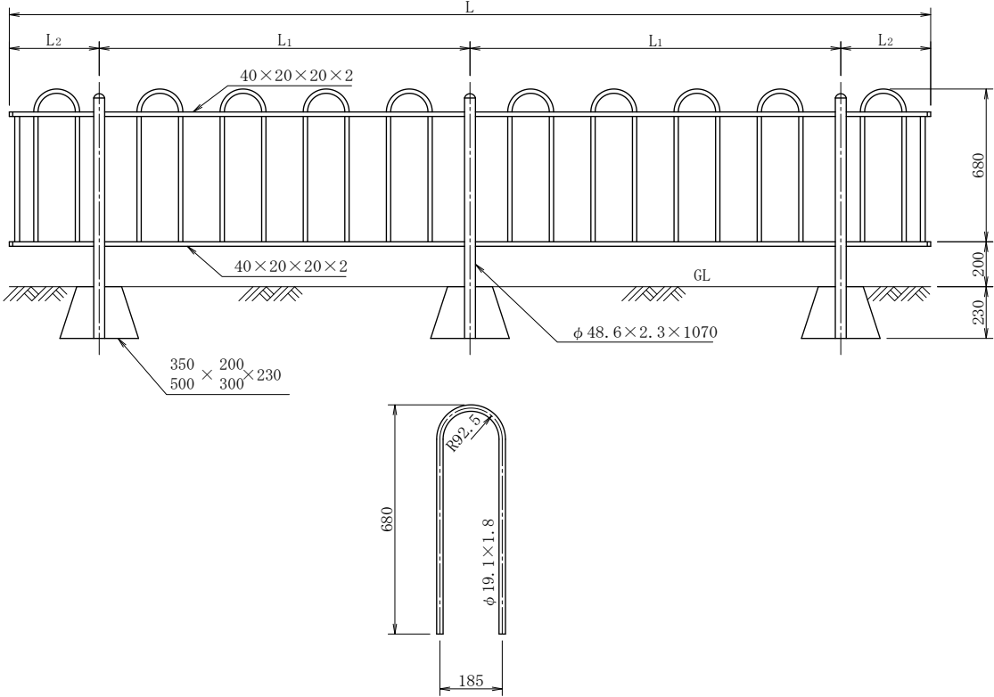
側面図
