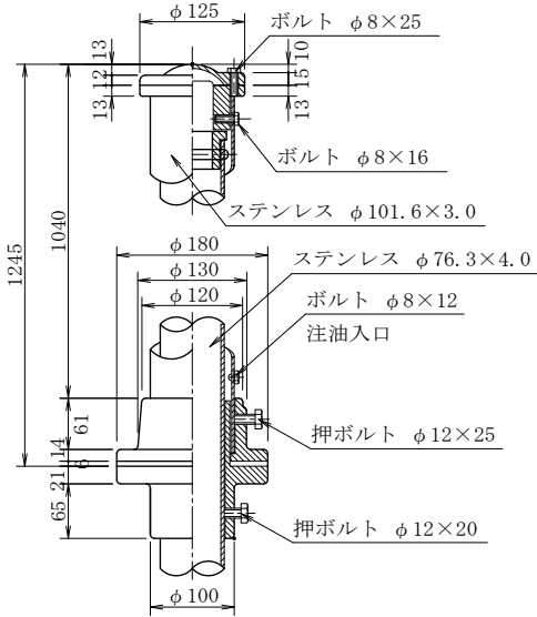
ツカミ部詳細図
