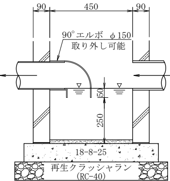
寸法表
