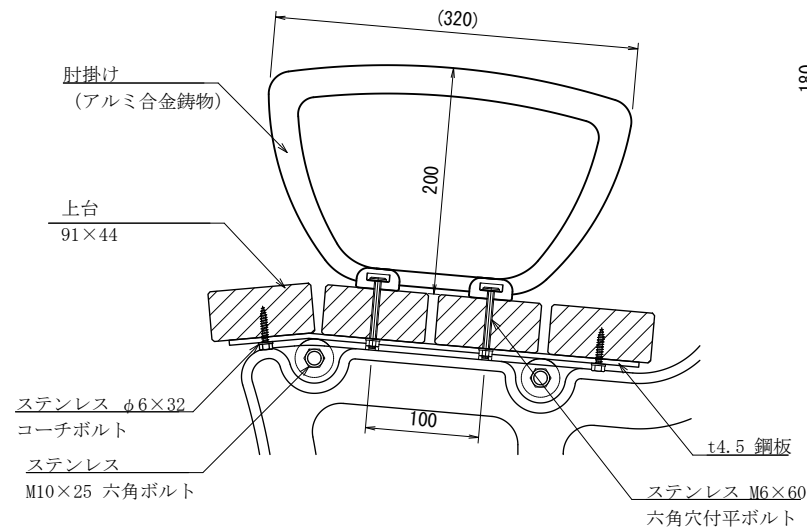
取合詳細図
