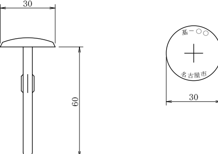
金属鋳 (黄銅製)
