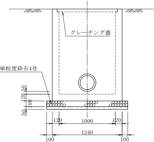
C-C 断面図
