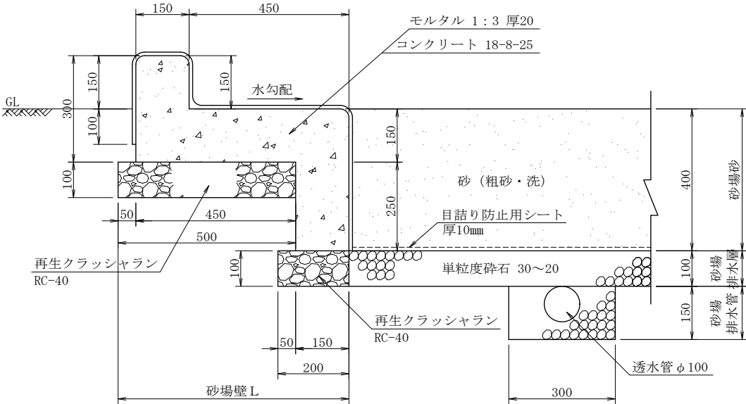
砂 場 壁 L
