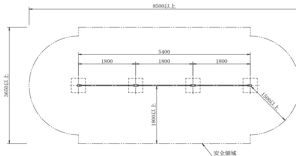
平面図
