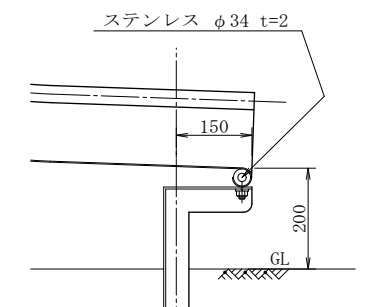
C部取付詳細図
