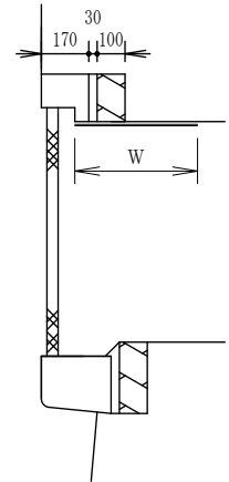
断 面 図
