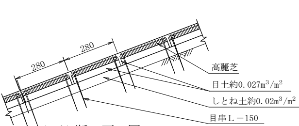
(E) 断 面 図
