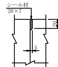
接合部詳細図
