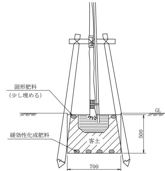
断 面 図
