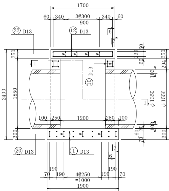
2 - 2 断 面
