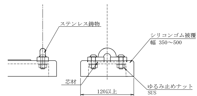
乗板参考図
