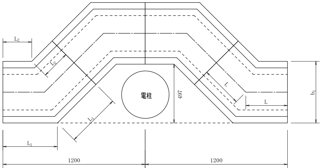
平 面 図
