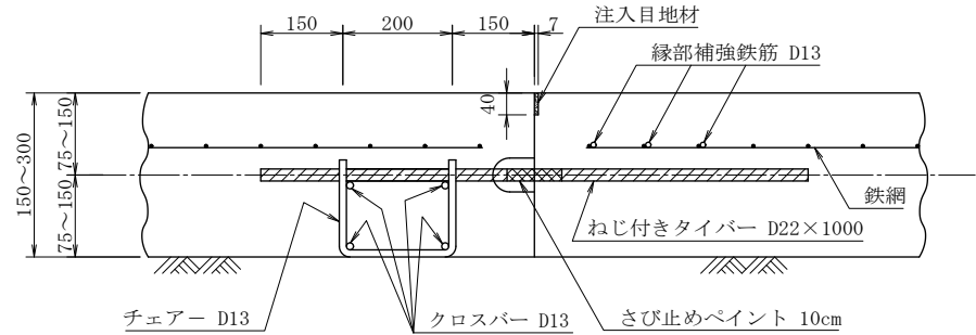
突 合 せ 目 地
