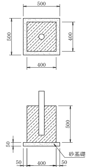
基礎工図 (E)
