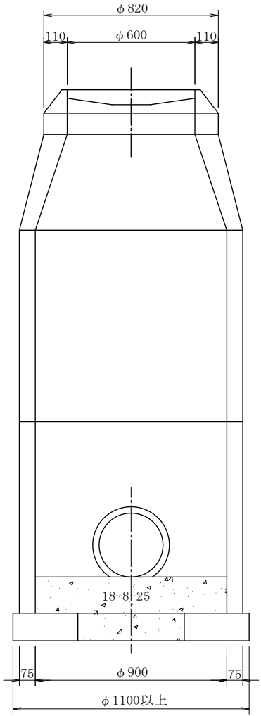
1 号直壁ブロック寸法表
