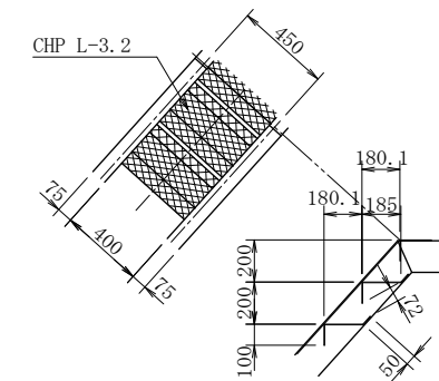
階段部詳細図
