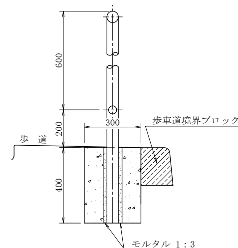
基礎工詳細図
