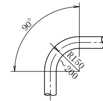
曲部詳細図
