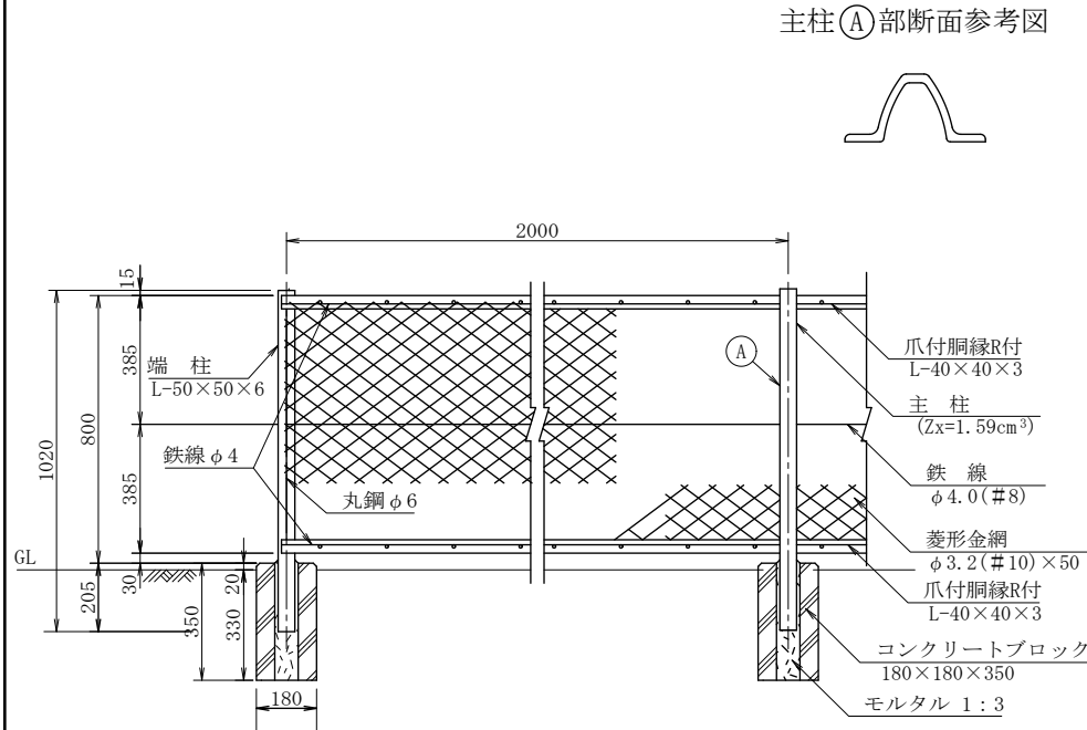
正面図 H=0.8m
