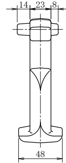
③ 蝶番金物詳細図
