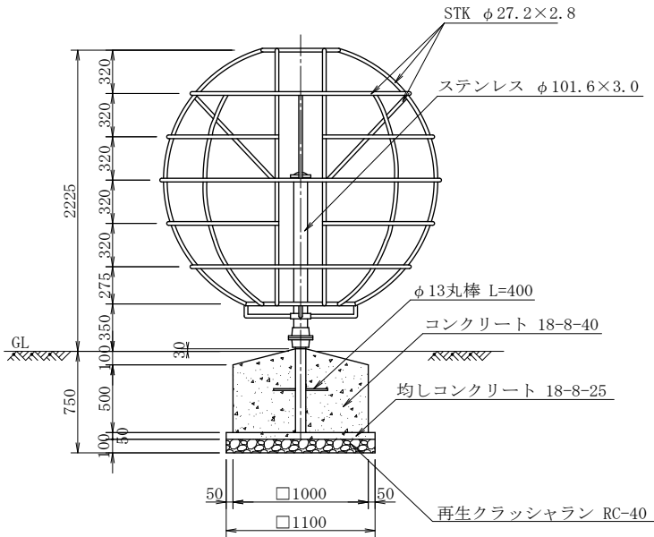
立 面 図
