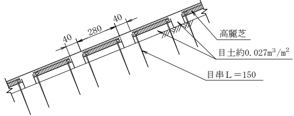
(B') 断 面 図
