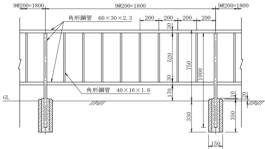
立 面 図
