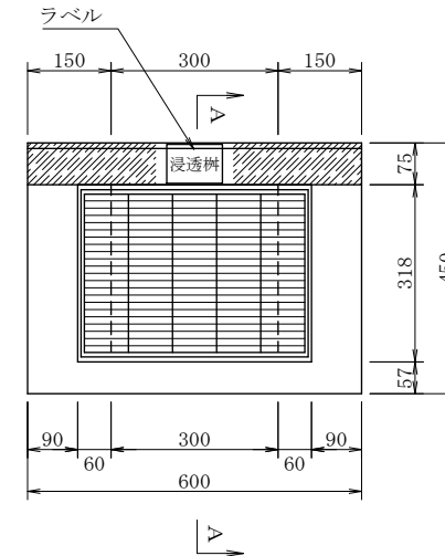
平面図
