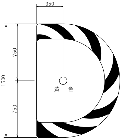
側 面 図
