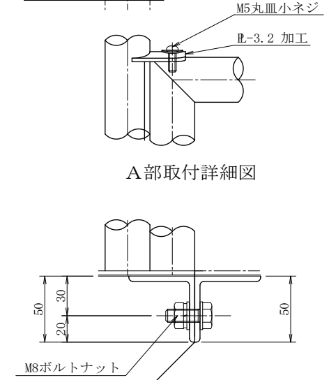
B部取付詳細図
