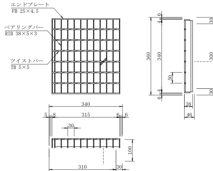
並目グレーチング
