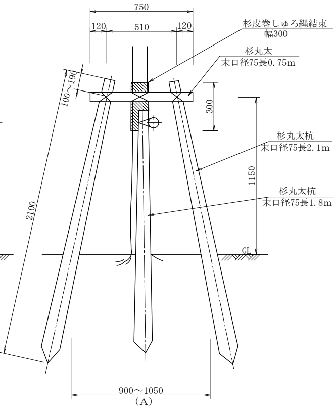
側 面 図
