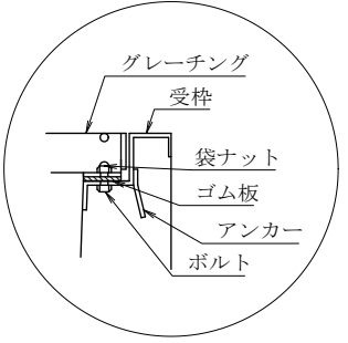
蓋取付部 (参考図)
