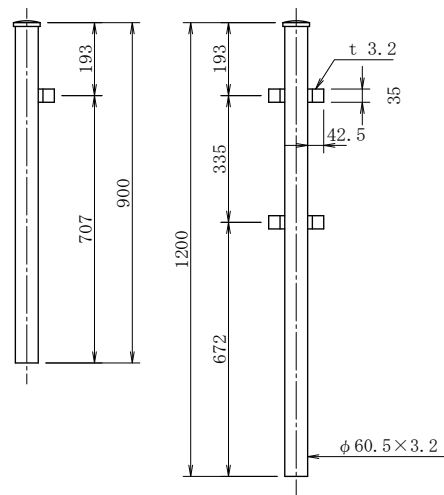
支柱
