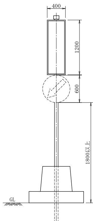
正 面 図
