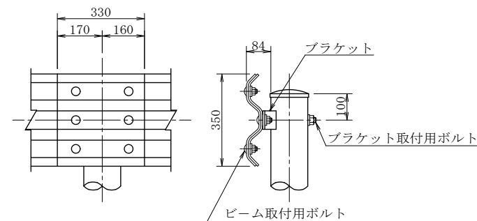
取付詳細図
