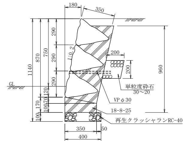
正 面 図 (参考図)
