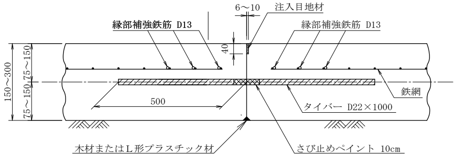
ダ ミ ー 目 地
