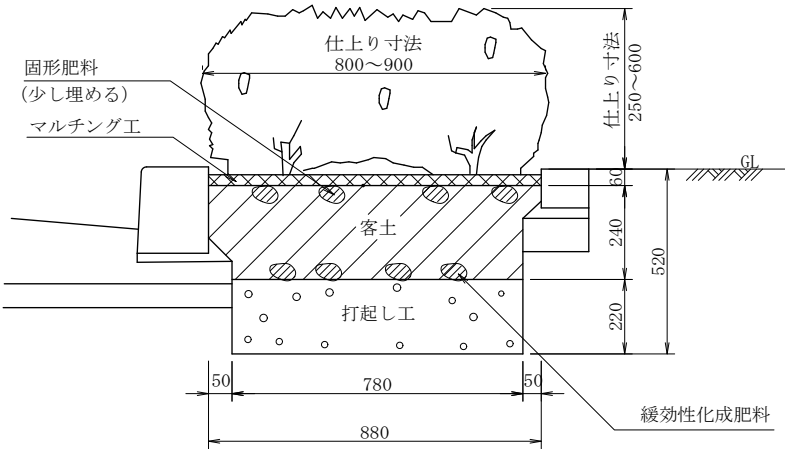
断面図
