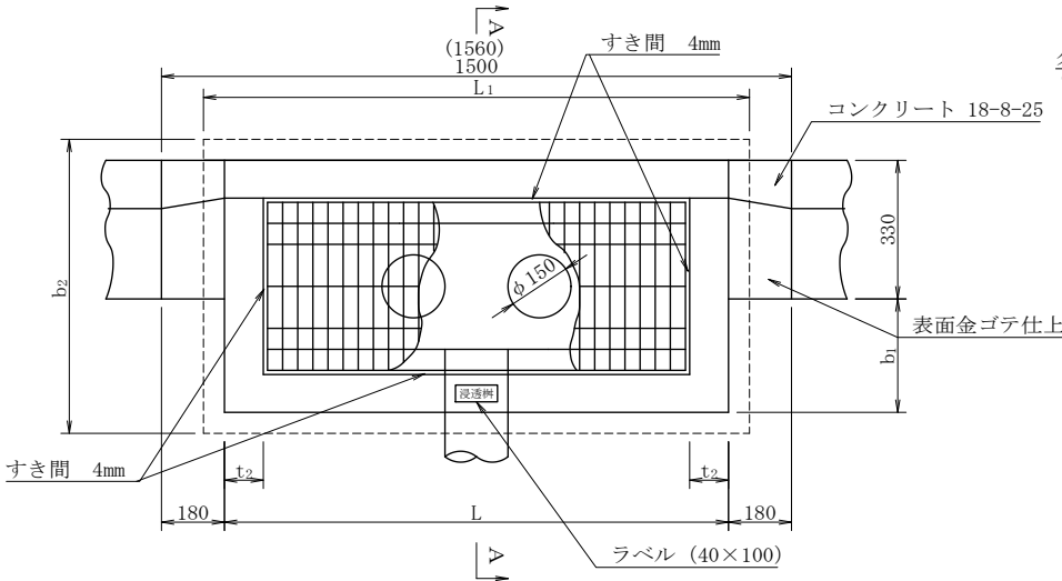
平 面 図
