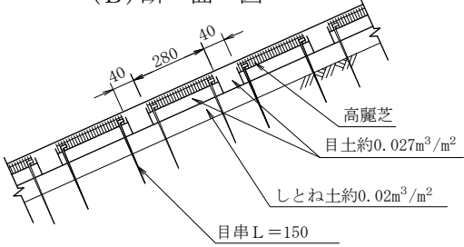
(B') 断 面 図
