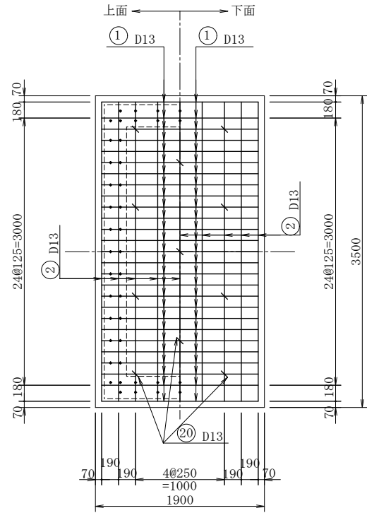
底 版
