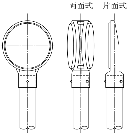
頭 部 詳 細 図
