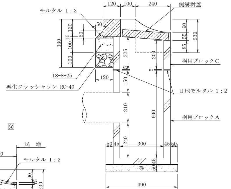
A-A 断 面 図
