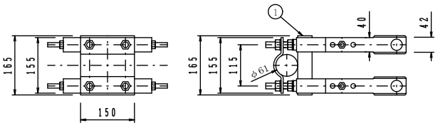
取付金具詳細図 S=1/15 溶融亜鉛メッキ仕上げ
