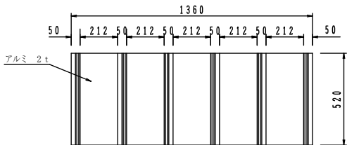
標識板裏面図 S=1/30
