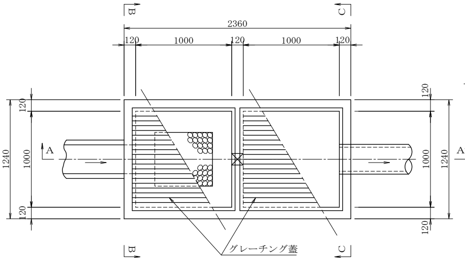
平面図
