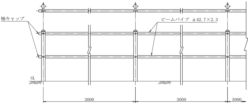
組立図
