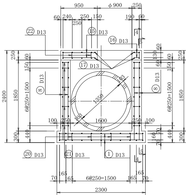
3 - 3 断 面
