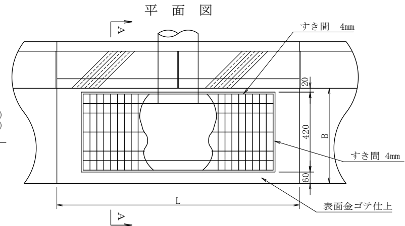
街渠柵工 (500A, 500B, 500C用) 寸法表
