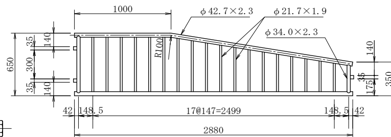
(端部パネル)
