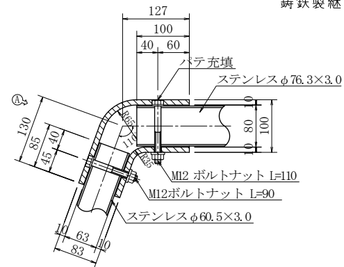
鋳鉄製継手詳細図
