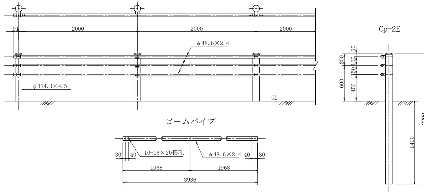
端部詳細図
