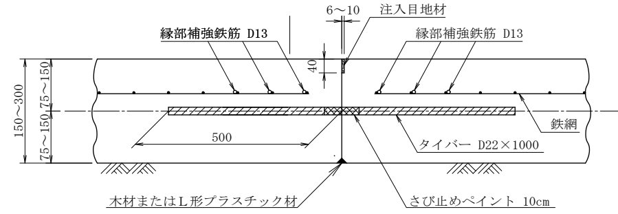
ダ ミ ー 目 地
