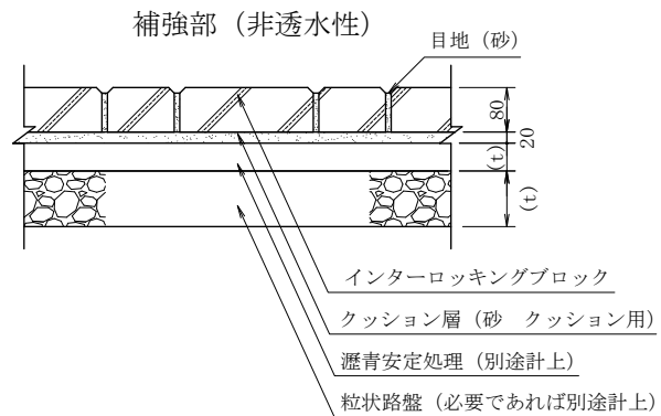
ブロック舗装工（歩道用）材料表
