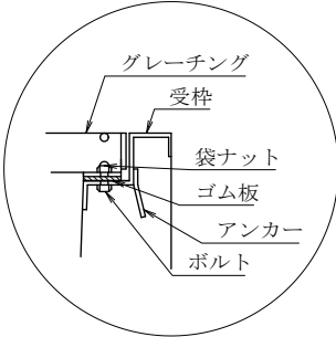
蓋取付部 (参考図)
