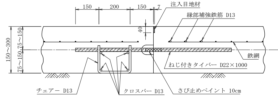
突 合 せ 目 地
