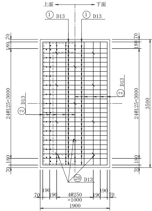
底 版
