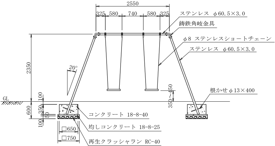
正 面 図
