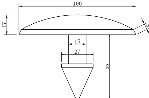
測量標（水準点）設置工材料表
