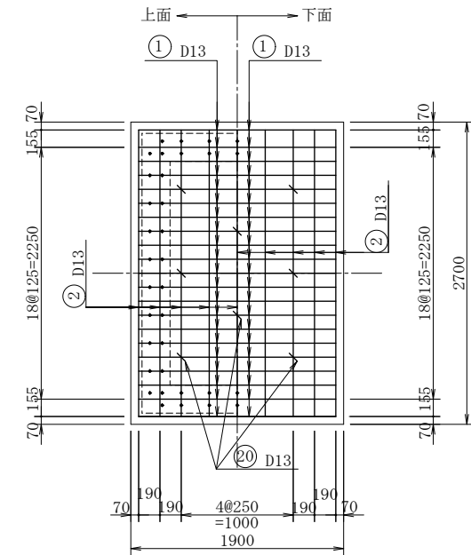
底 版
