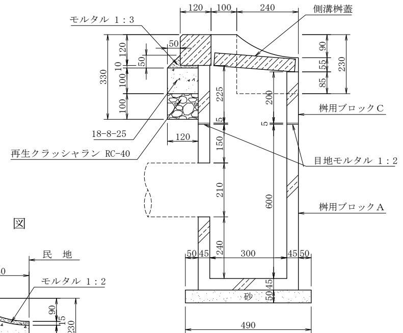
A-A 断面図
