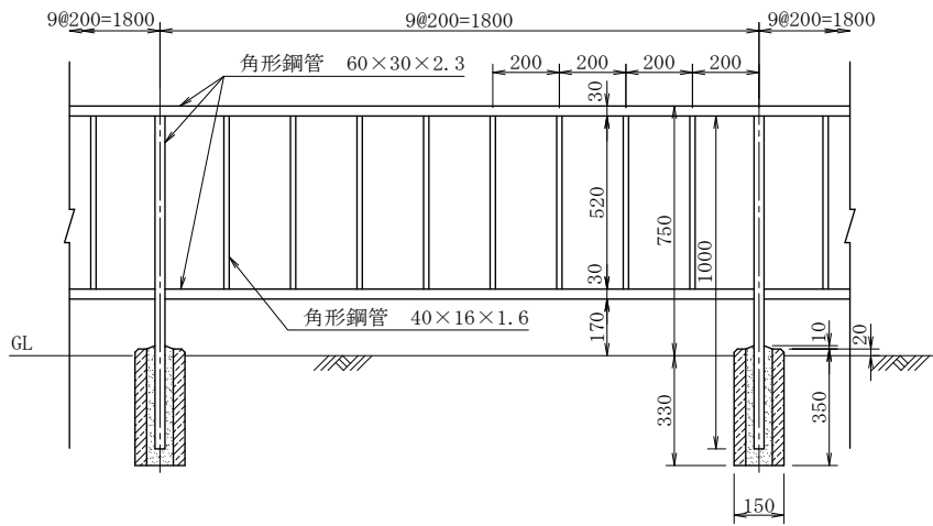
立 面 図
