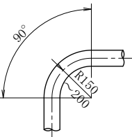
曲部詳細図
