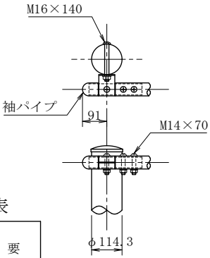
端部詳細図
