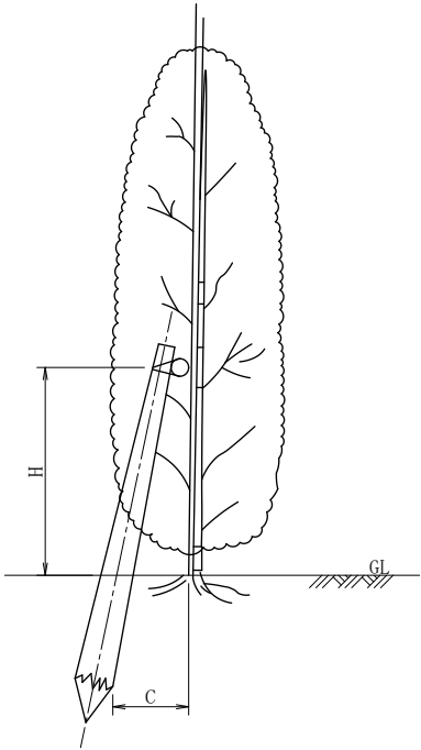
側 面 図
