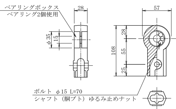
吊金具詳細図
