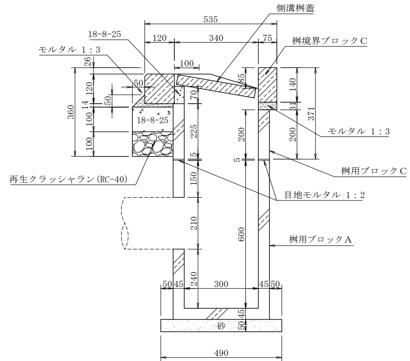
A-A 断面图
