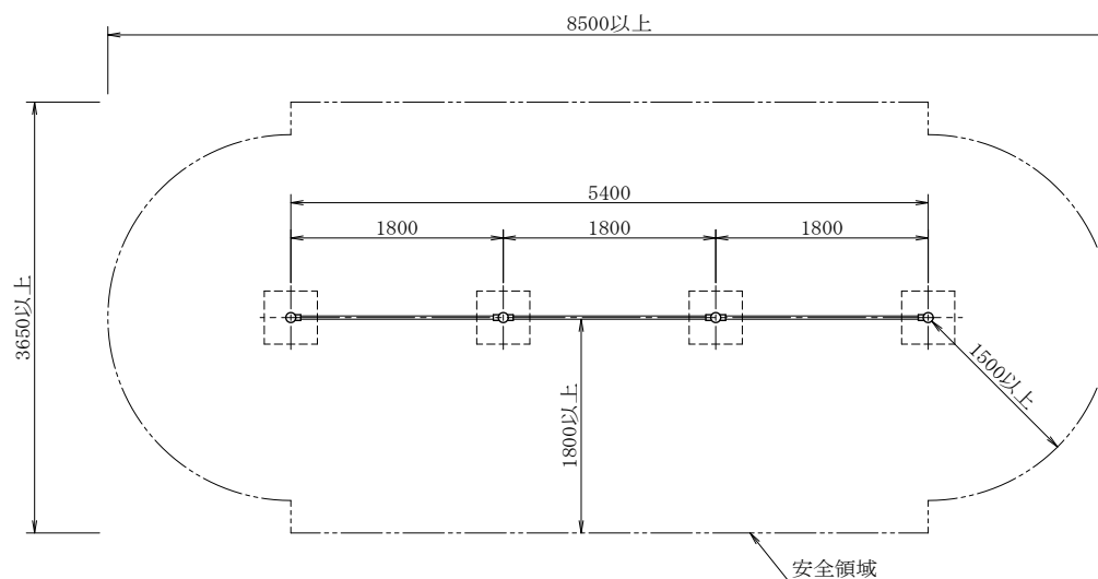
平面図
