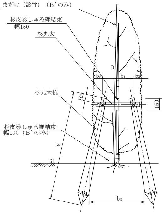
正 面 図
