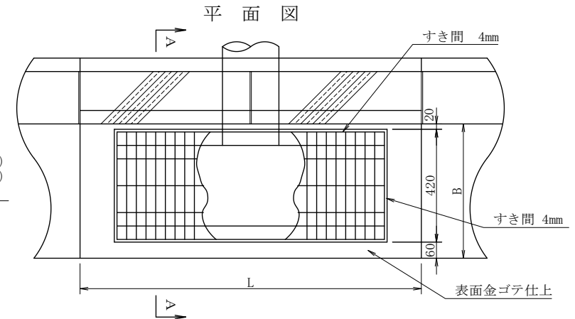
名 称 寸 法 表 単位 (mm) 摘 要 B b 1 b 2 b 3 b 4 H h 1 h 2 h 3 h 4 h 5 t t 1 t 2 L 街渠柵工 500B用 現 場 打 560 205 255 600 700 1270 250 150 210 120 1050 150 90 50 1270 ブロック 500 205 255 540 640 1240 250 150 240 120 1020 120 60 20 1210 街渠柵工 500C用 現 場 打 560 210 260 600 700 1320 300 200 210 170 1050 150 90 50 1270 ブロック 500 210 260 540 640 1290 300 200 240 170 1020 120 60 20 1210 街渠柵工 500A用 ブロック 500 170 220 540 640 1240 200 150 240 120 1020 120 60 20 1210
