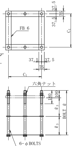
アンカーボルト詳細図
