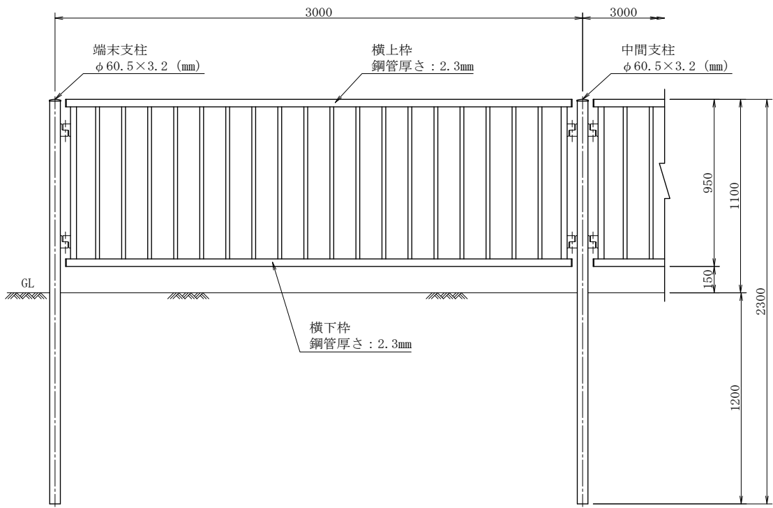
組立図
