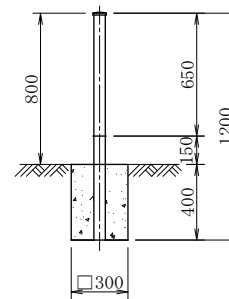
断面図
