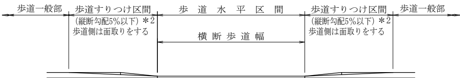
A－A' 断面
