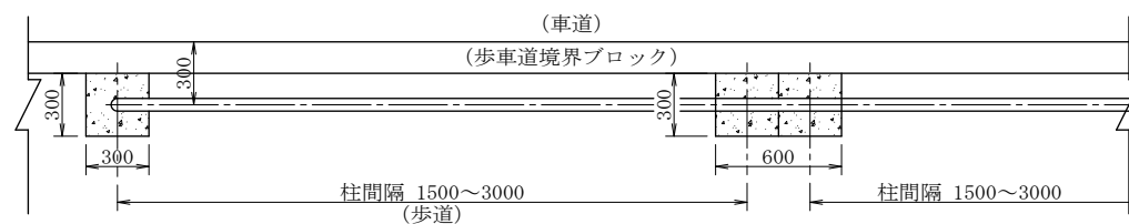
平面图
