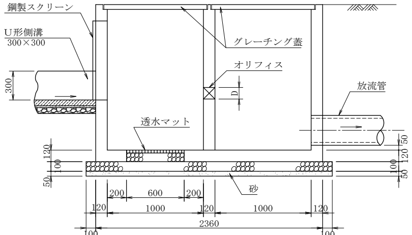
A-A 断面図
