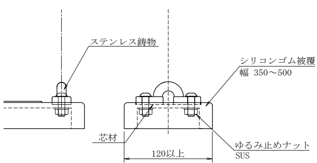
乗板参考図
