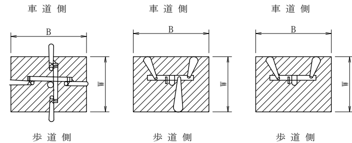
平 面 図
