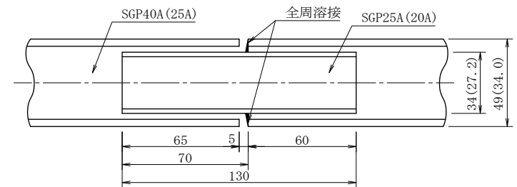
伸 縮 継 手 詳 細 図
