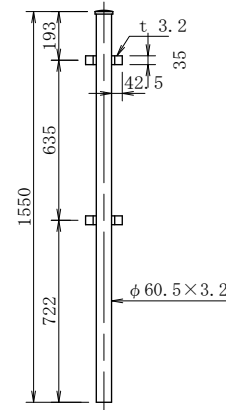
支 柱
