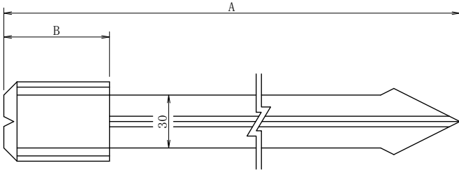
鉄杭寸法表
