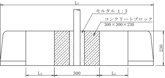
断面図
