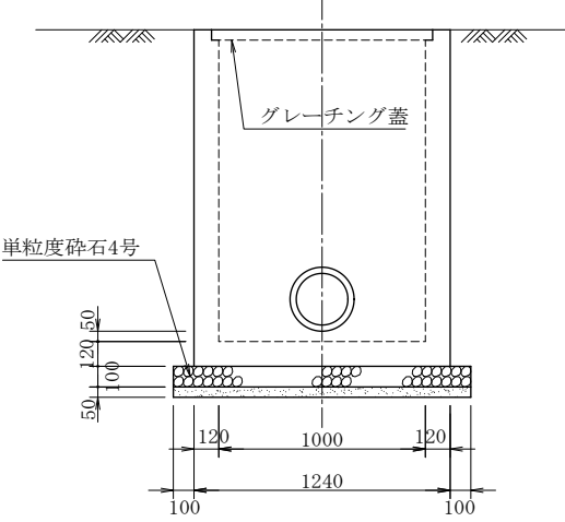
C-C 断面図
