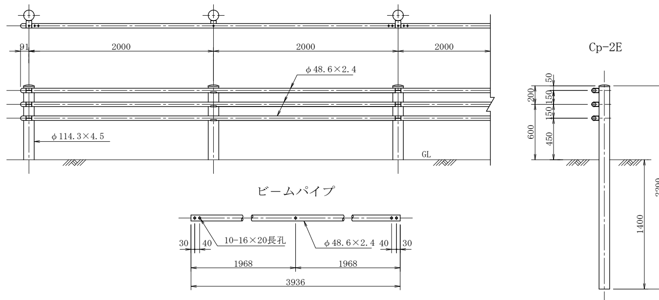
端部詳細図
