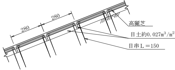
(E') 断 面 図
