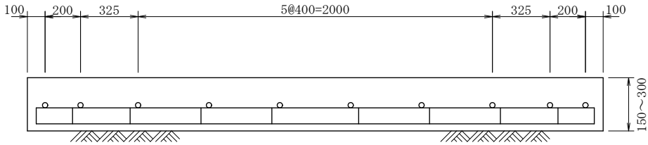
断 面 図
