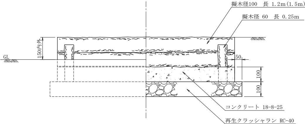
立 面 図
