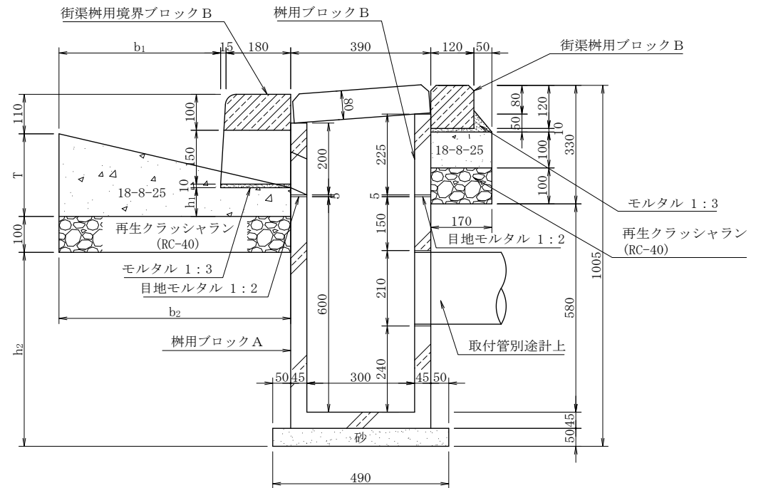
A-A 断面图
