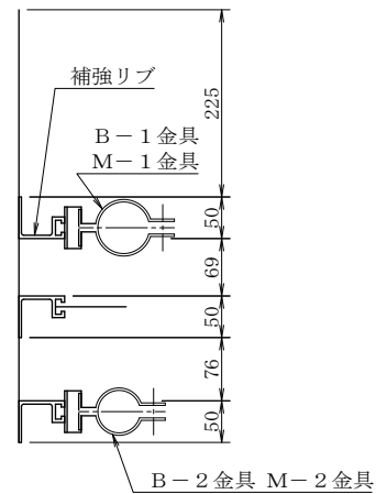
M-2 金具
