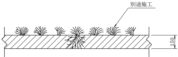
公園地被客土工
