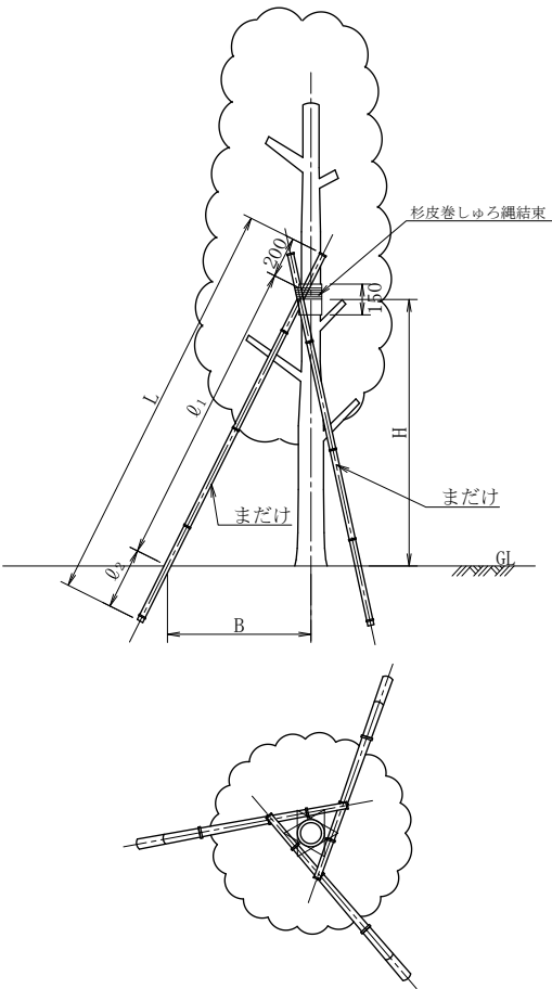
三本竹支柱
