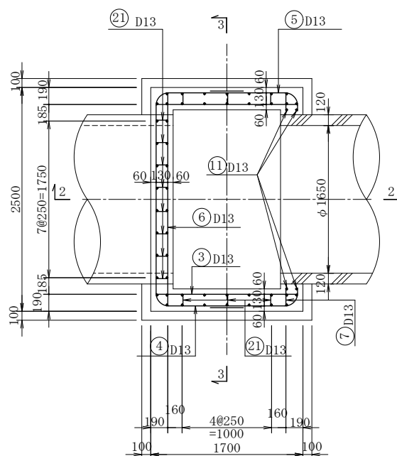
1 - 1 断 面
