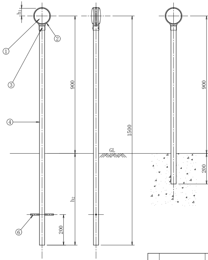
視線誘導標設置工寸法表
