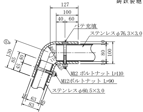
鋳鉄製継手詳細図
