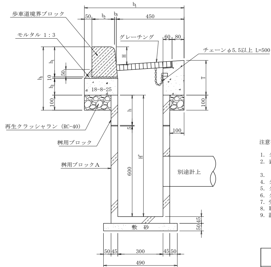
A—A 断面
