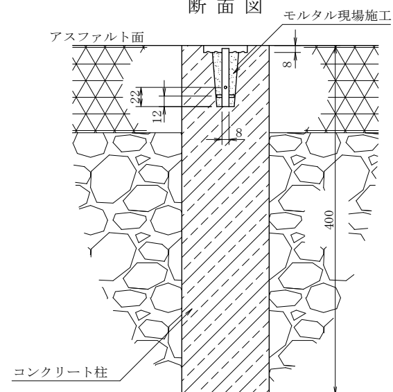
断面図
