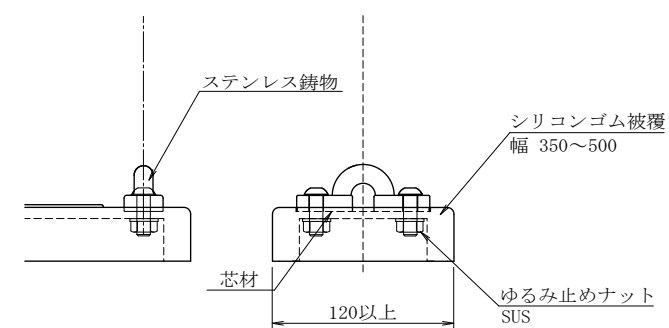
乗板参考図
