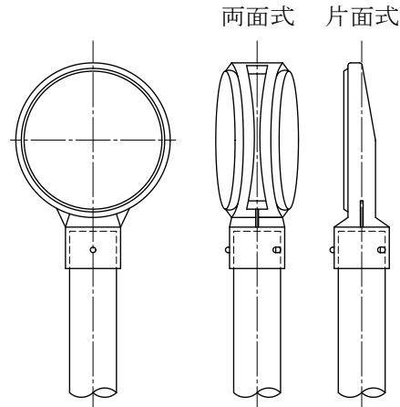
頭 部 詳 細 図
