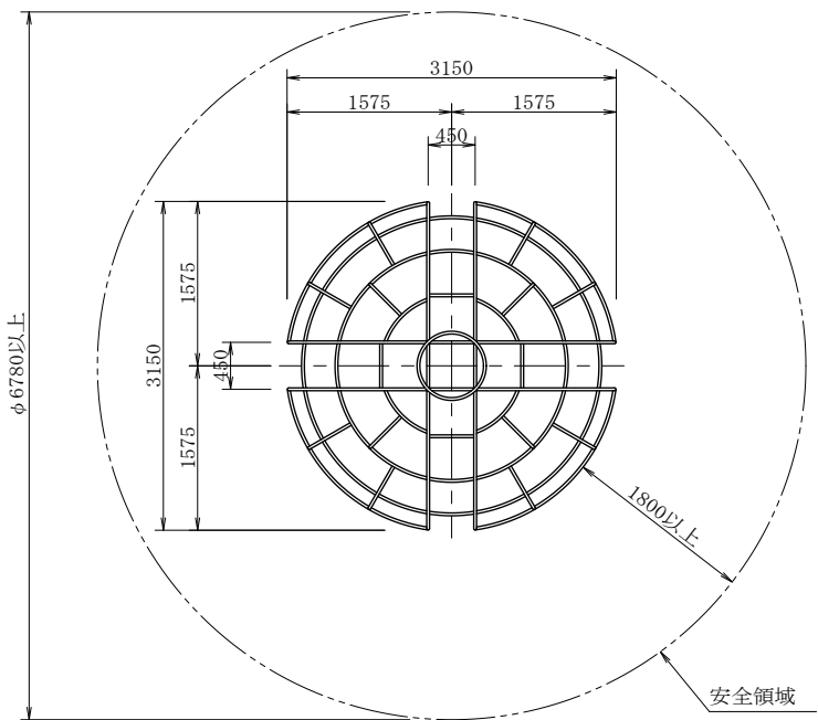
平 面 図
