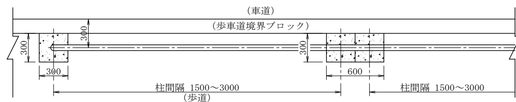
平 面 図
