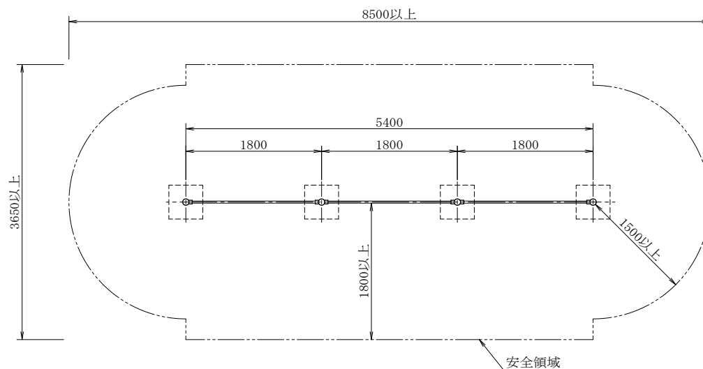
平 面 図
