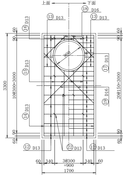
頂 版
