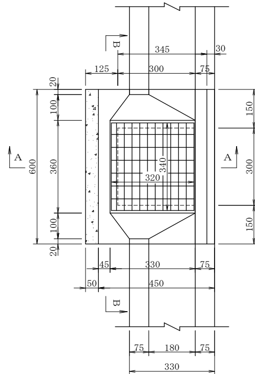
グレーチング 320×340×38 L形樹上部ブロック 450×600× 159 185 コンクリート18-8-25 再生クラッシュラン (RC-40) モルタル 1:3 樹用ブロック D チェーンφ5.5以上 L=500 目地モルタル 1:2 樹用ブロック A 砂 Dimensions (mm): Top width: 45, 330, 75 Top height: 159, 185 Middle height: 20, 100, 100, 5, 150, 210, 240 Bottom height: 45, 50, 45, 50 Total height: 1105 Total width: 490 Other dimensions: 75, 75, 180, 50, 60, 45, 35, 80, 200, 5, 600, 125, 80, 50, 45, 50
