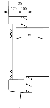
断 面 図
