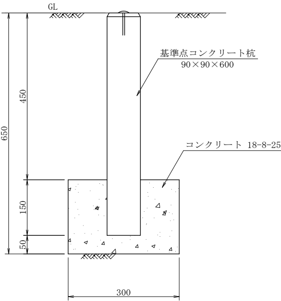
断 面 図
