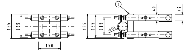
取付金具詳細図 S=1/15 熔融亜鉛メッキ仕上げ
