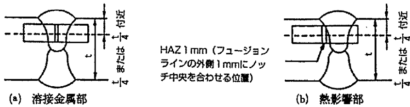
図3-2 衝撃試験片採取位置
