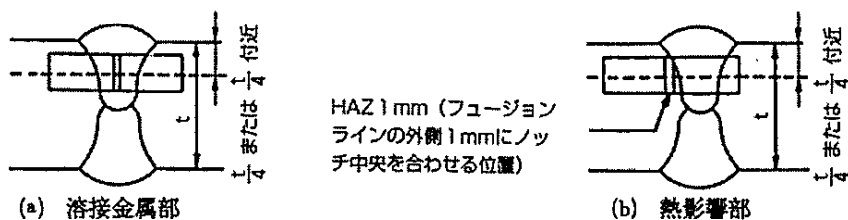
圖 3-2 衝擊試驗片採取位置
