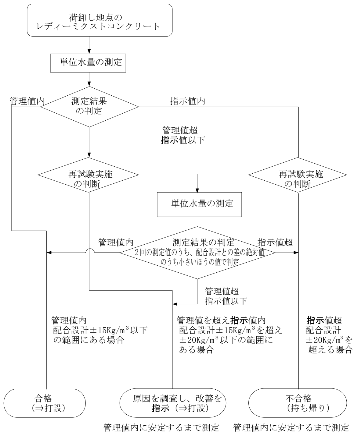
図2-2 レディーミクストコンクリート単位水量測定の実施管理フロー図
