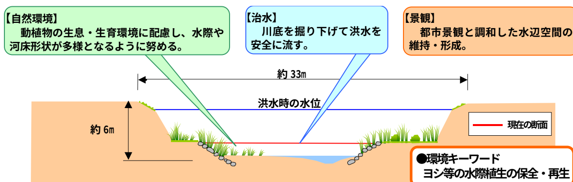
図-23 植田川横断イメージ図（0.6km 付近）
