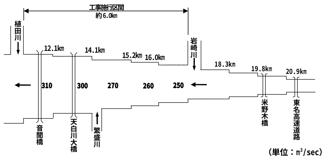
図-13 河川整備計画の目標とする流量配分図（天白川上流※）
