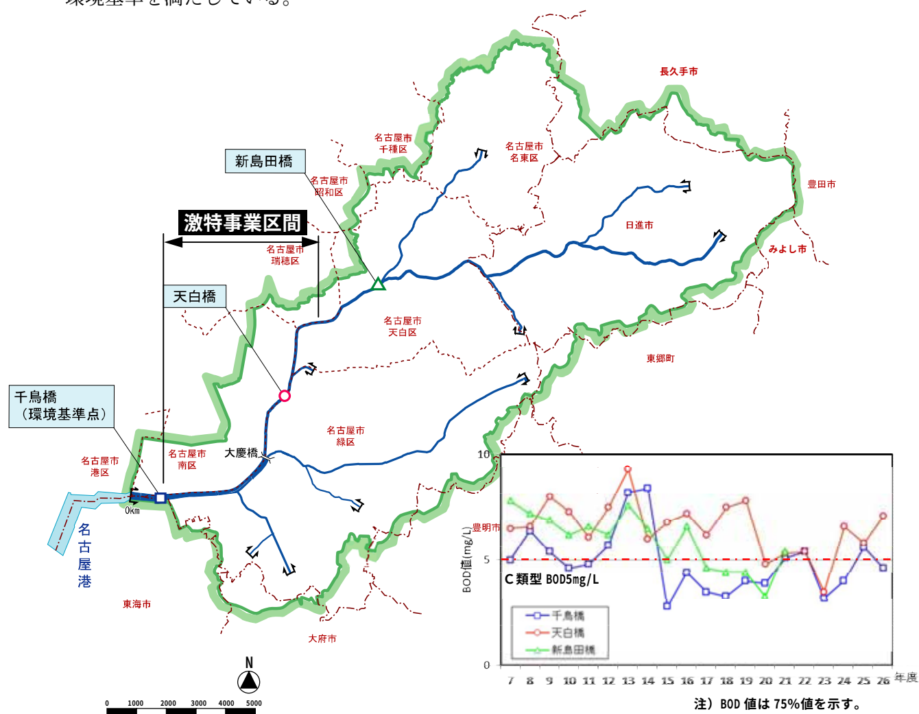
図－8 水質観測地点と水質の経年変化
