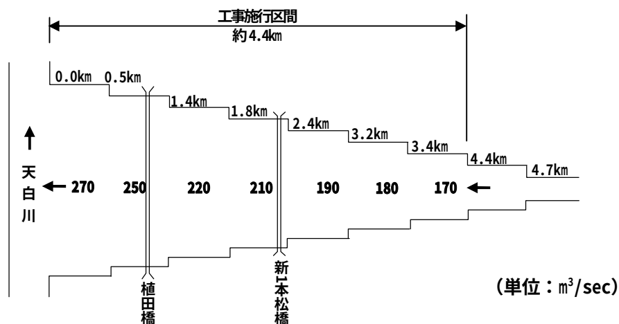
図-21 河川整備計画の目標とする流量配分図（植田川）
