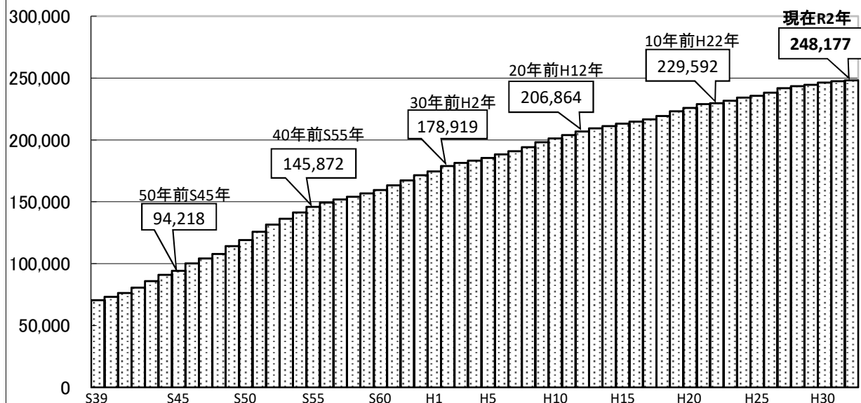
図3 人口の推移
