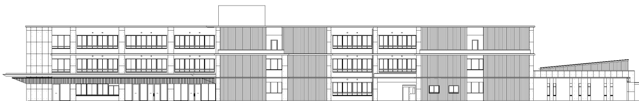
北立面图
