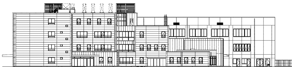
東立面图
