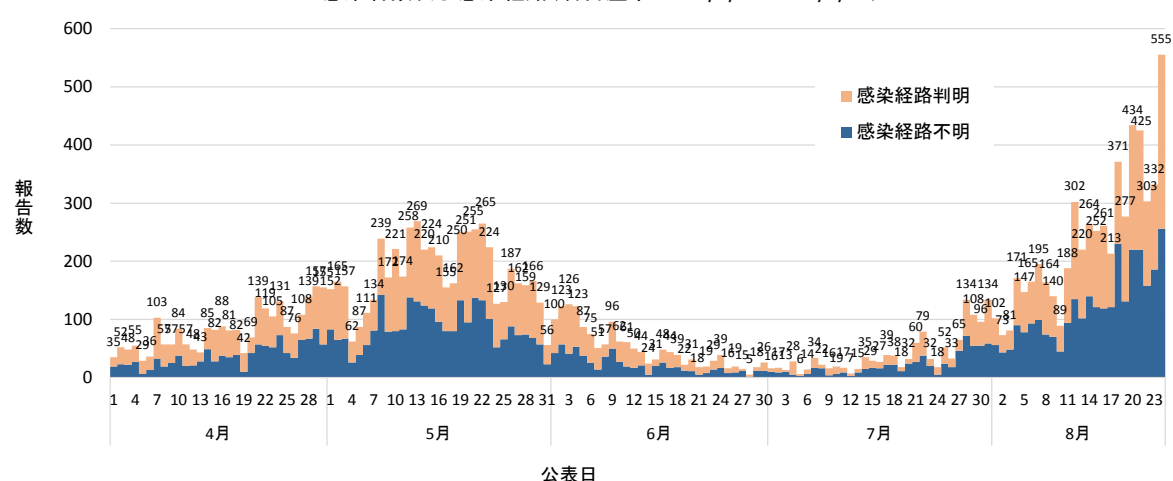
感染者数及び感染経路(名古屋市:2021/4/1～2021/8/24)
