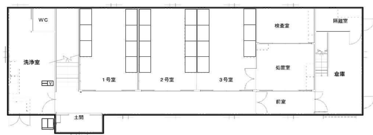
一時飼育施設 1階平面図
