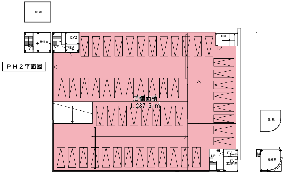
R 階平面図
