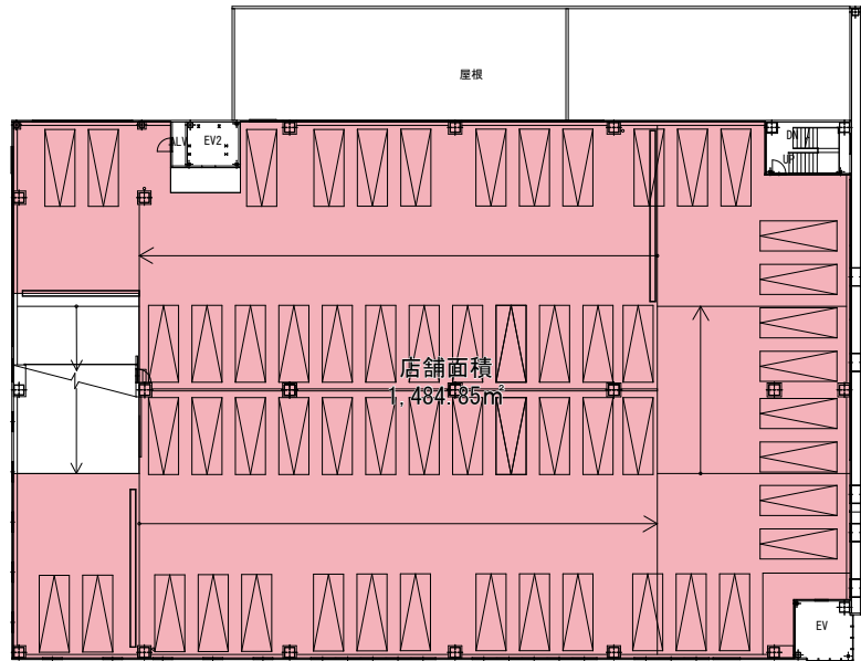
3 階平面図
