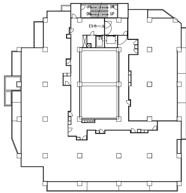
4～14階平面図
