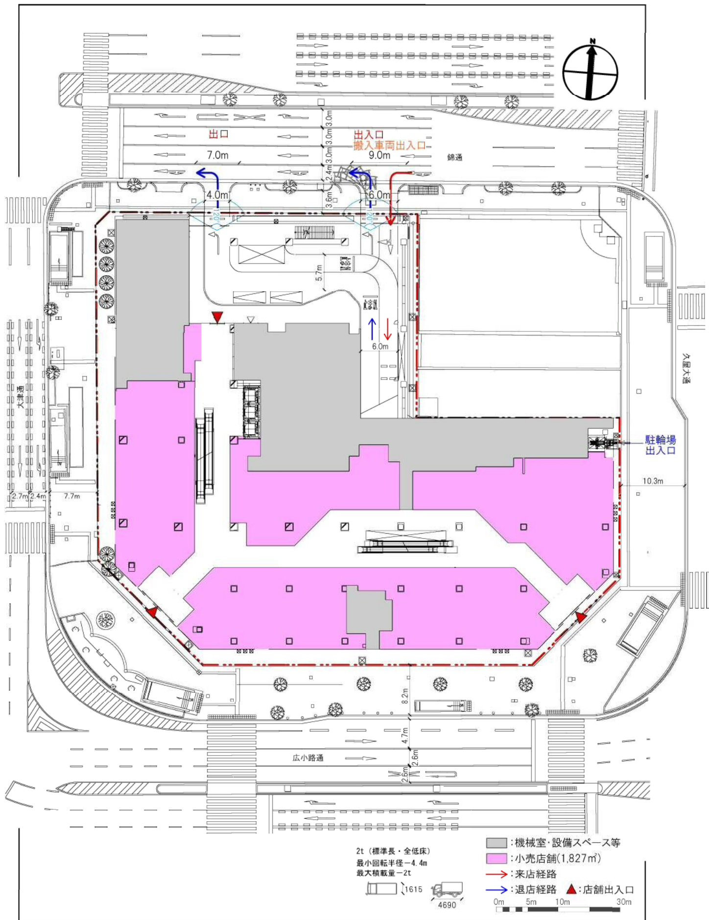
別添図面7 配置図兼1階平面図(1/600)
