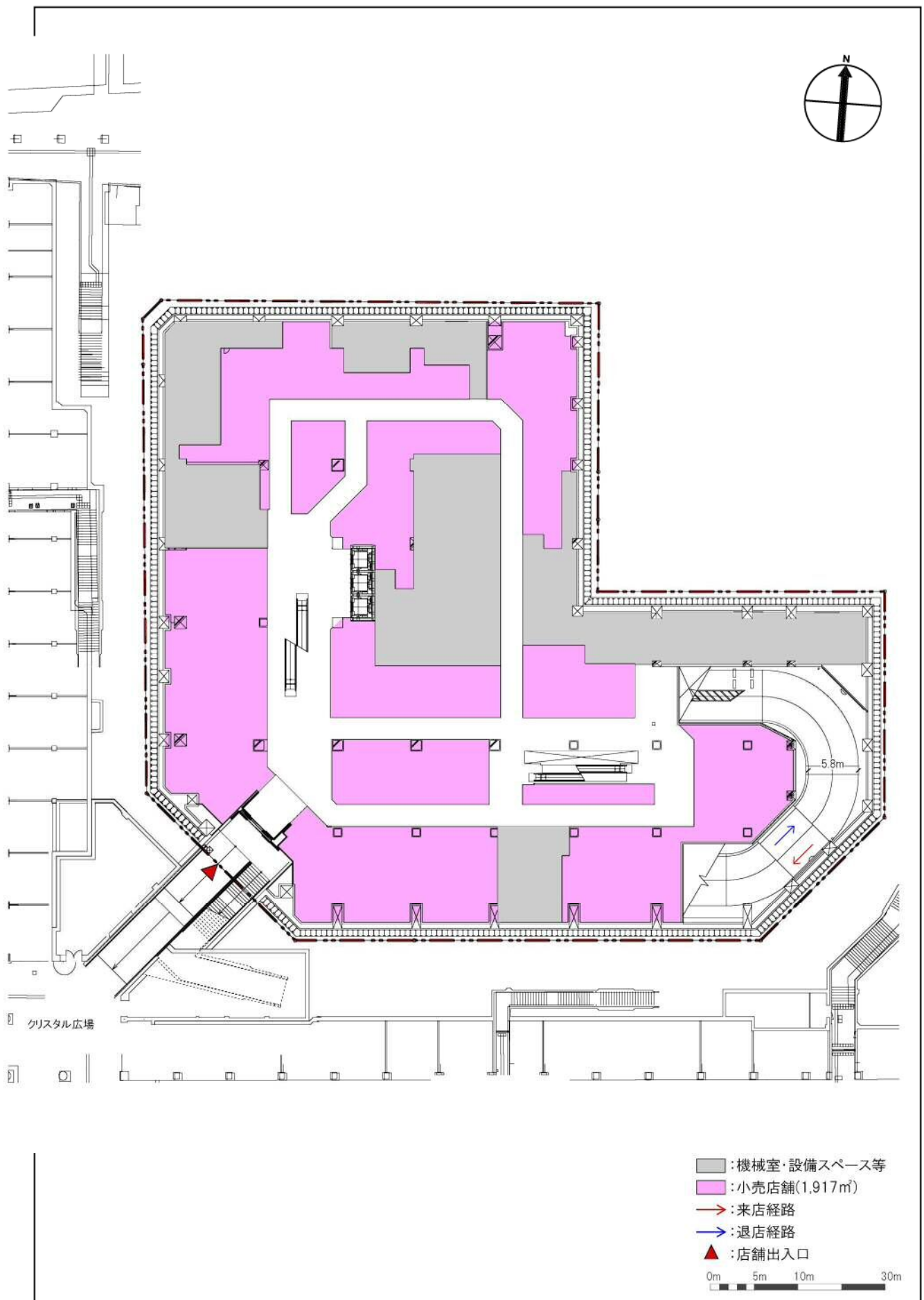
別添図面5 地下2階平面図(1/600)
