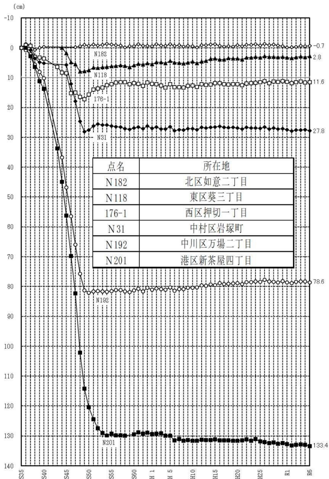
図ー1 主要水準点の累積沈下状況（昭和36年から令和6年まで）
