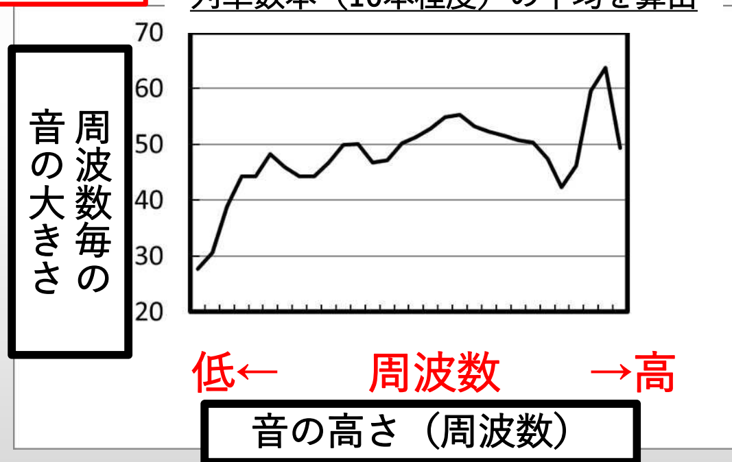
騒音周波数スペクトル
