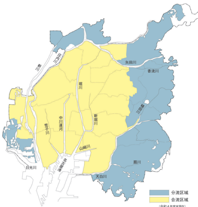
図資-11 分流式下水道・合流式下水道 区域図
