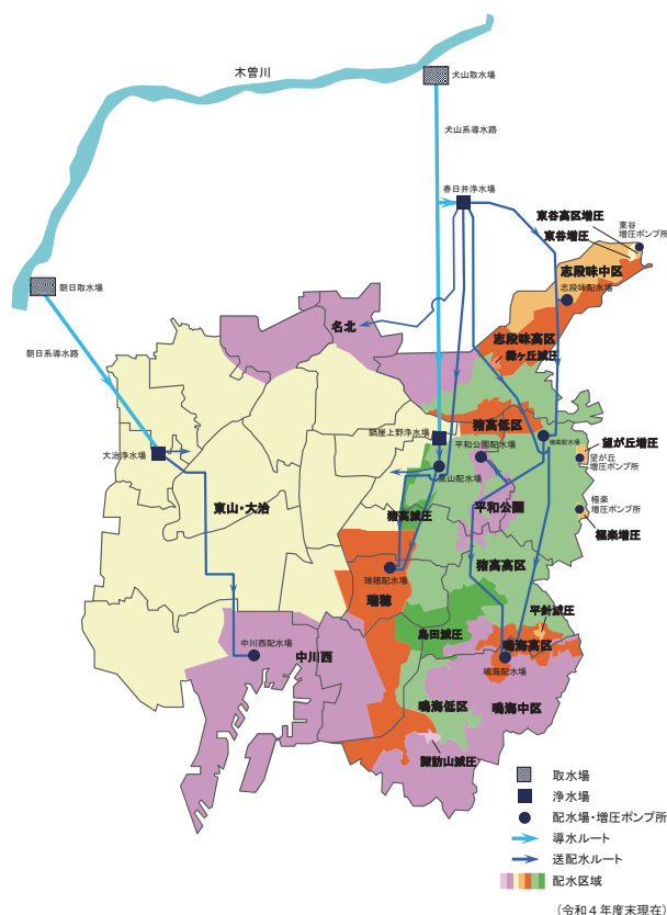
図 資-9 配水系統図 出典) 令和6年度版 なごやの水道・下水道
