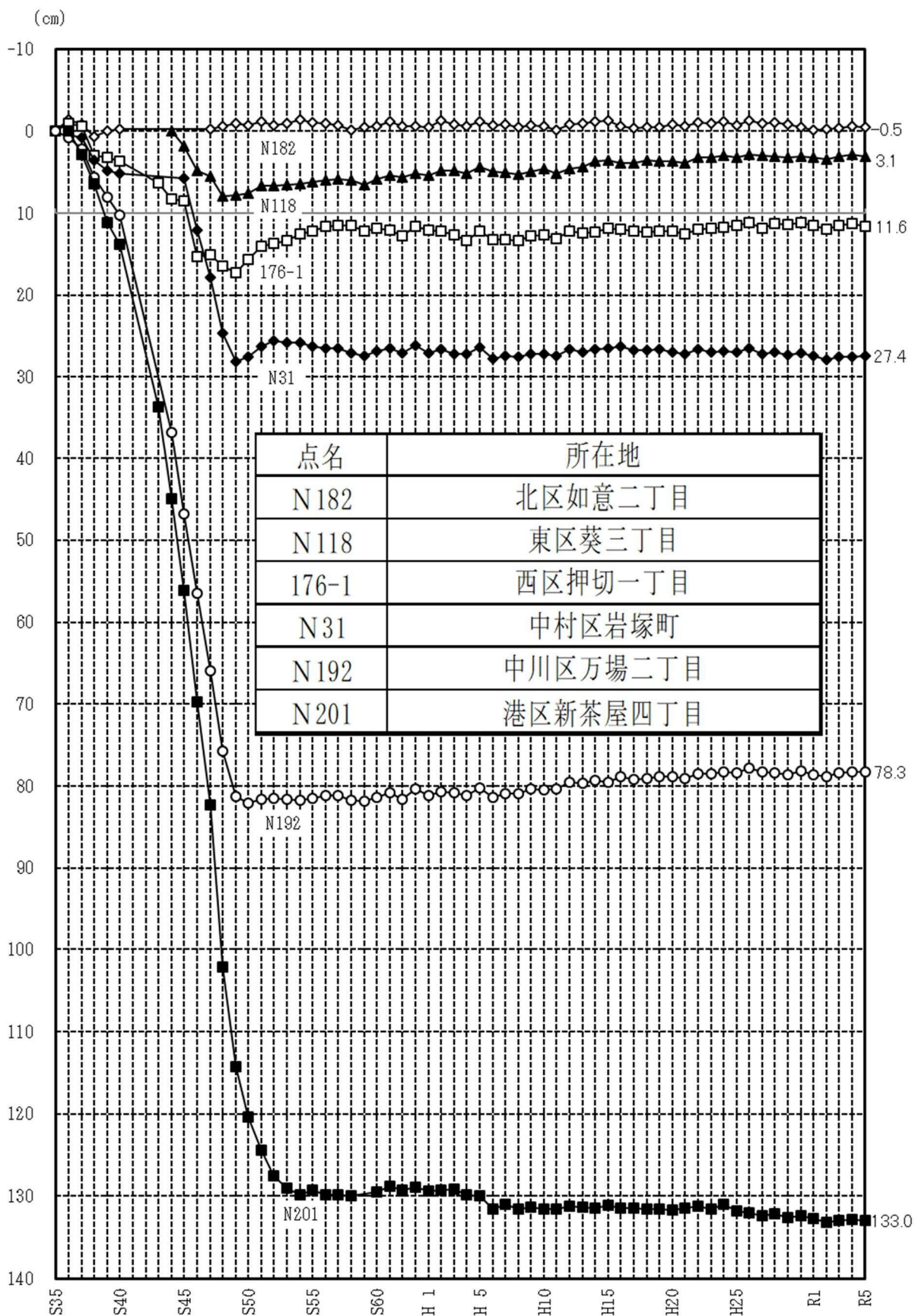
図ー1 主要水準点の累積沈下状況（昭和36年から令和5年まで）
