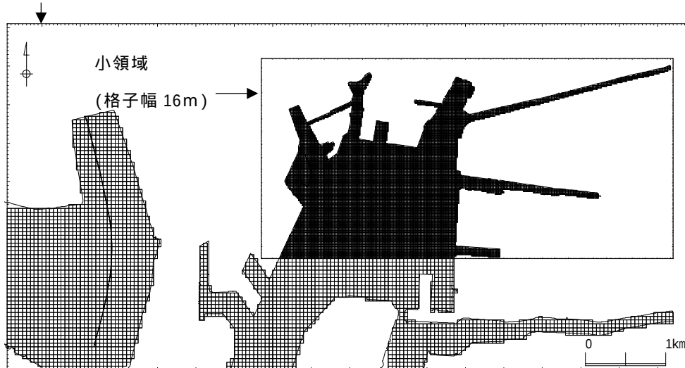
図 7-4-2(2) 格子分割図 (中領域)
