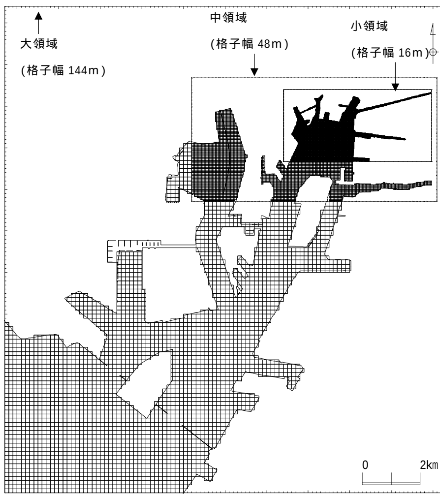
図 7-4-2(1) 格子分割図 (大領域)
