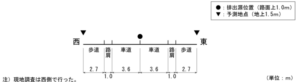
No.4 断面
