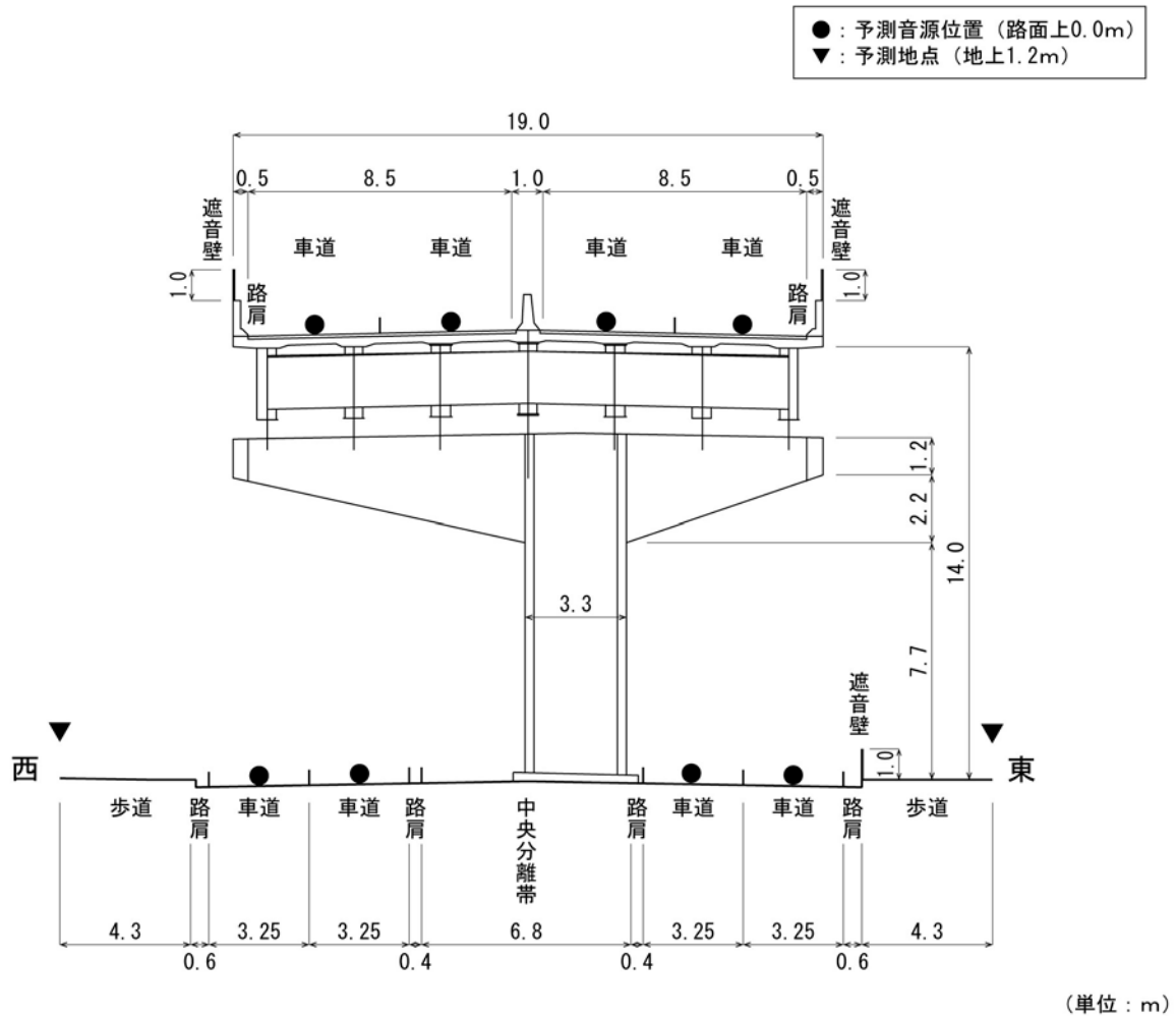
No.4 断面
