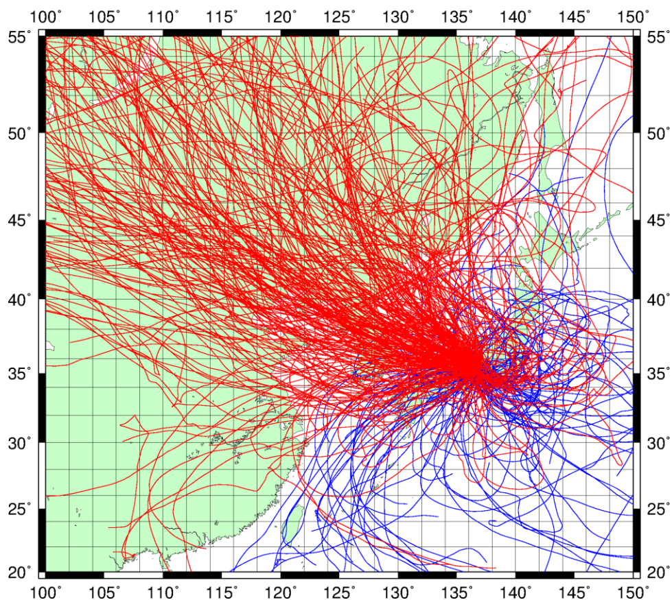
図11 後方流跡線解析による気塊の流れ（令和3年度）
