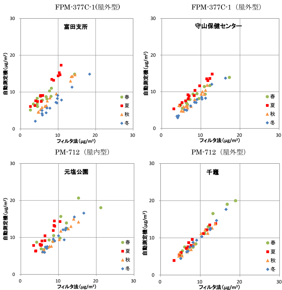
図10 標準測定法（フィルタ法）と自動測定機によるPM2.5質量濃度の比較
