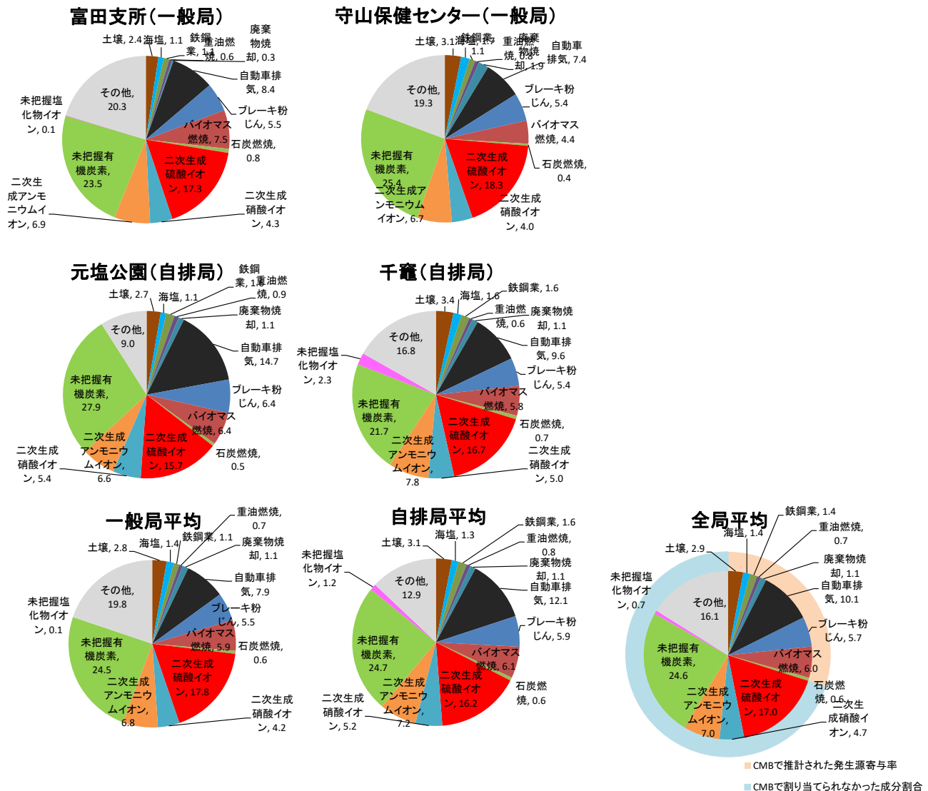
図 8 CMB 法による発生源寄与割合 (%) (令和 3 年度)
