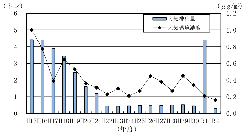
図21 スチレンの届出大気排出量と大気環境濃度
