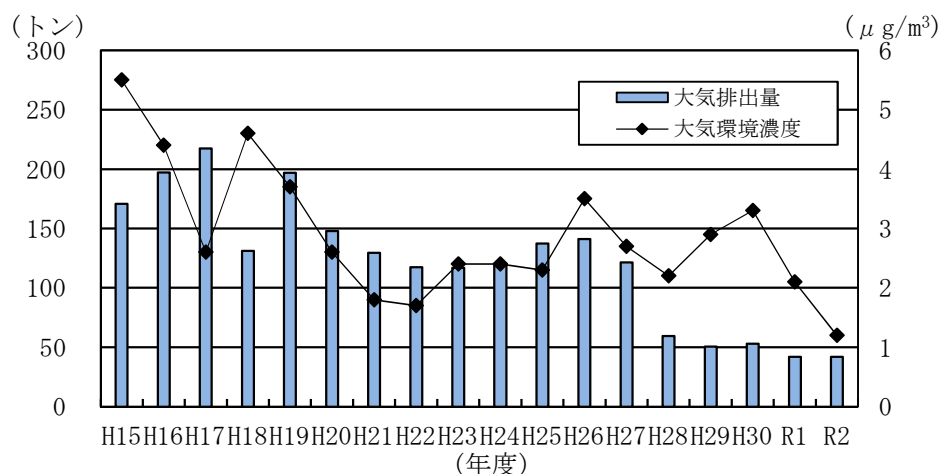
図19 エチルベンゼンの届出大気排出量と大気環境濃度
