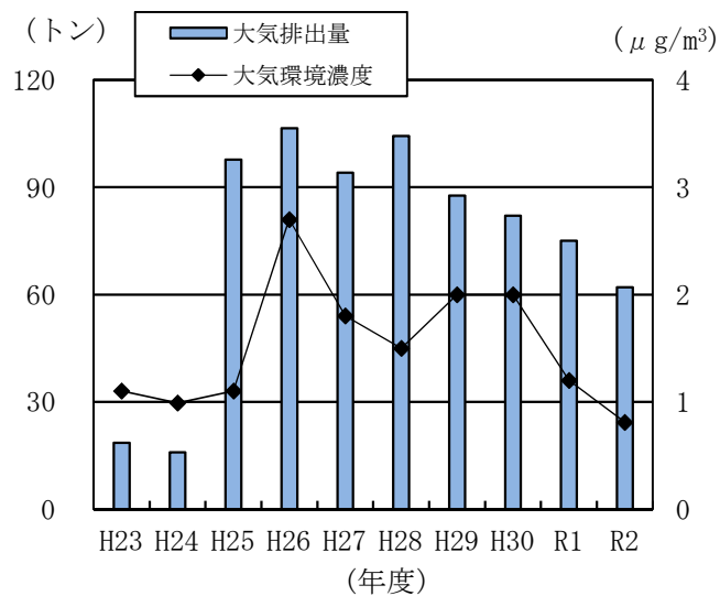
図23 1,2,4-トリメチルベンゼンの届出大気排出量と大気環境濃度
