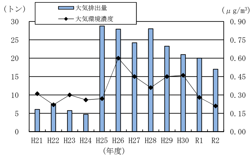
図22 1,3,5-トリメチルベンゼンの届出大気排出量と大気環境濃度
