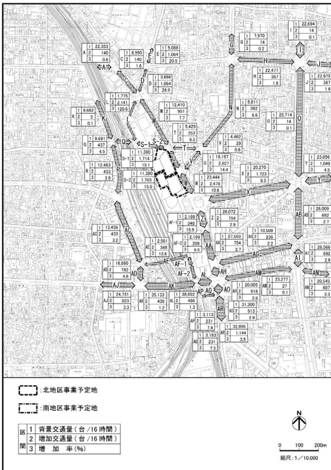
図 7-2-1(2) 供用時増加交通量及び増加率(休日)
