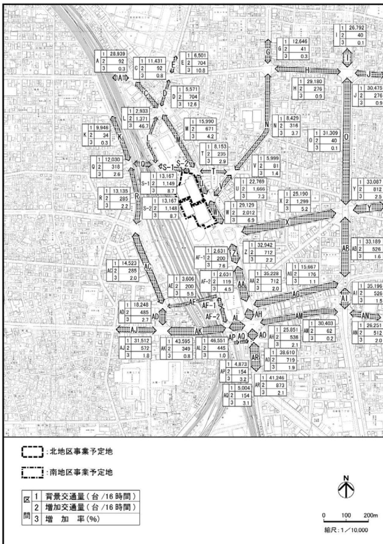
図 7-2-1(1) 供用時増加交通量及び増加率(平日)
