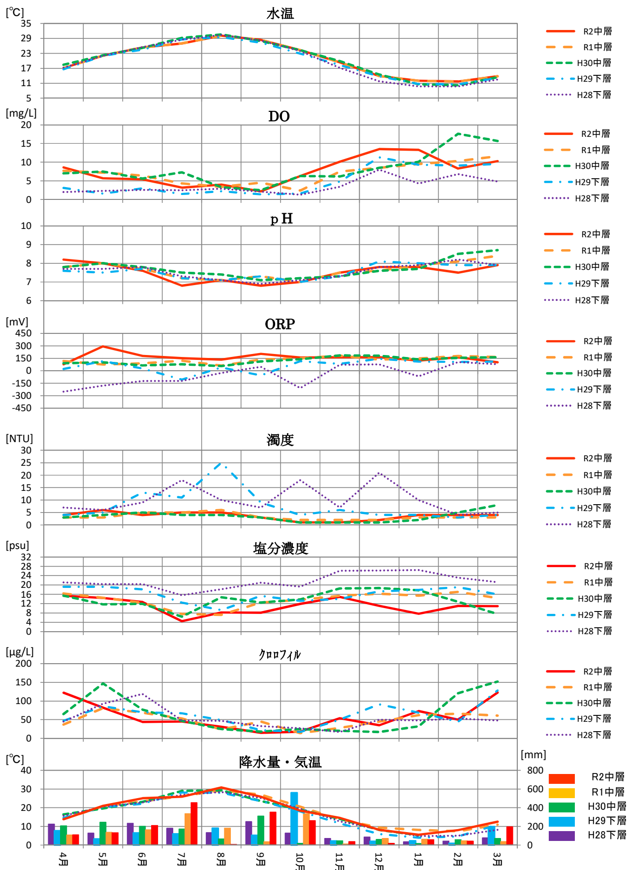
図 2-3 中川運河小栗橋中層の過去との比較 (グラフ)
