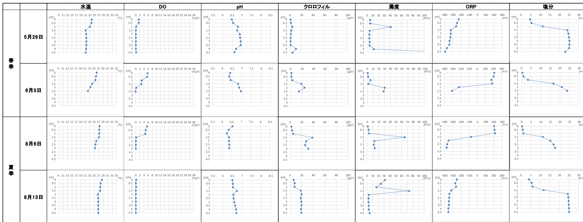
図 3-7 新堀川舞鶴橋の深さ別調査結果（その 1）
