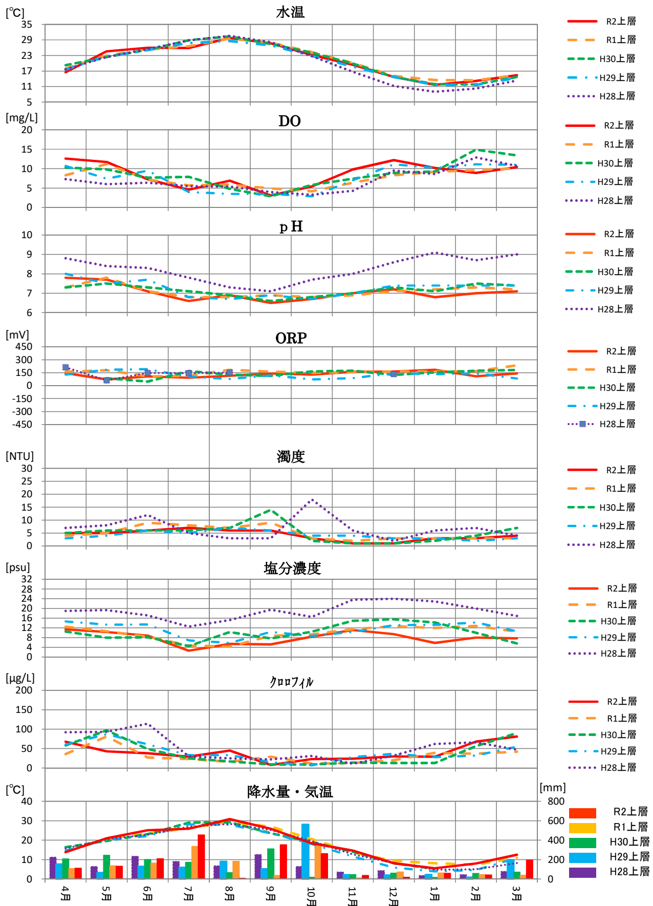
図 2-2 中川運河小栗橋上層の過去との比較 (グラフ)
