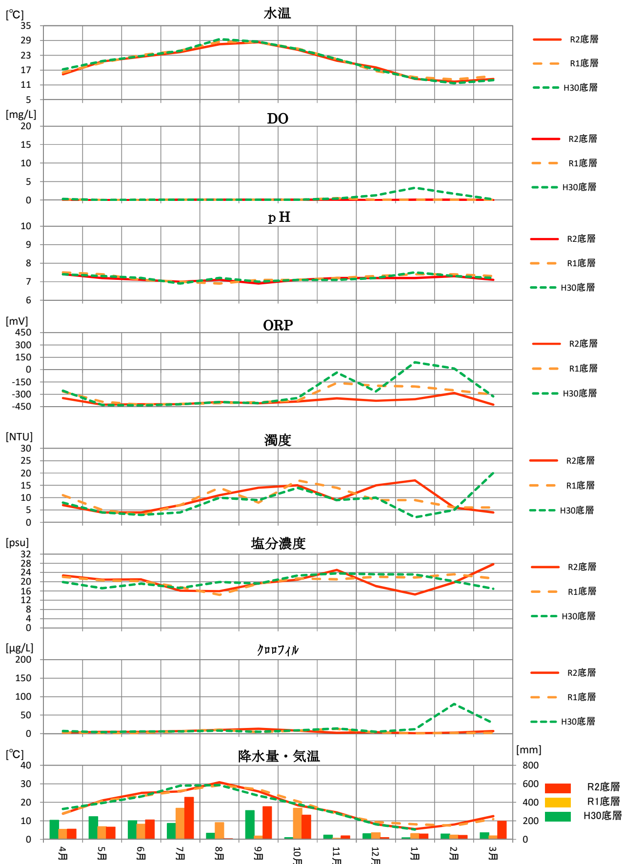
図 2-4 中川運河小栗橋底層の過去との比較 (グラフ)
